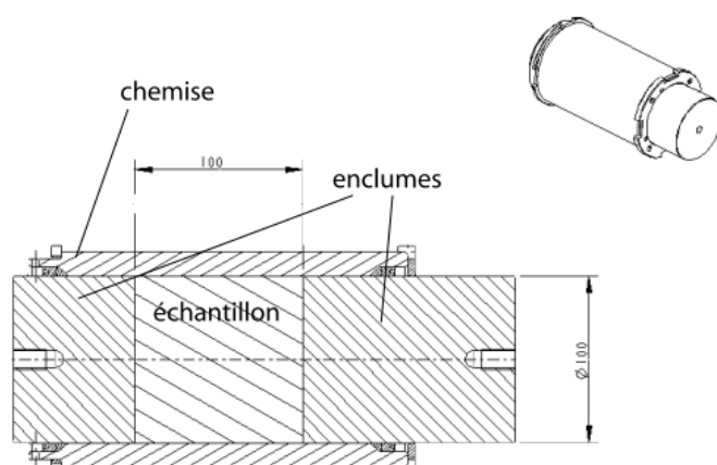
Figure 2-40. Dispositif oedométrique
