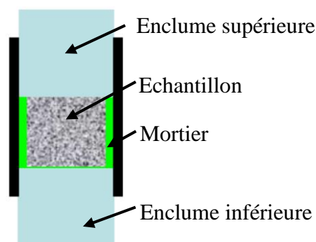
Figure 2-41. Echantillon positionné dans la chemise avant le test oedométrique
