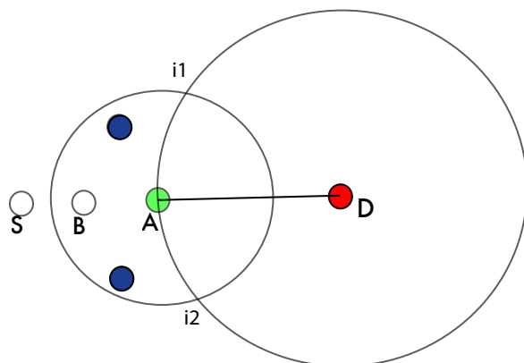
FIGURE 5.4 – N_D(A) est vide, le routage glouton vers D échoue A .
