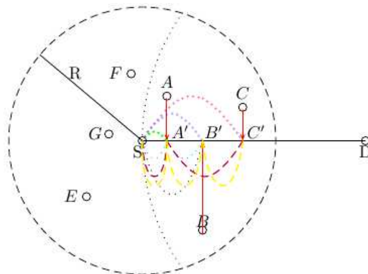
FIGURE 3.3 – Relocalisation des nœuds dans MobileR-MultipleORouting (flèches rouges). Une partie des différents chemins possibles est aussi représentée.
