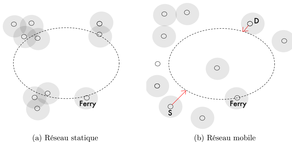
FIGURE 2.3 – Les ferries en action transportant physiquement les messages dans leur mémoire avant ré-émission.
