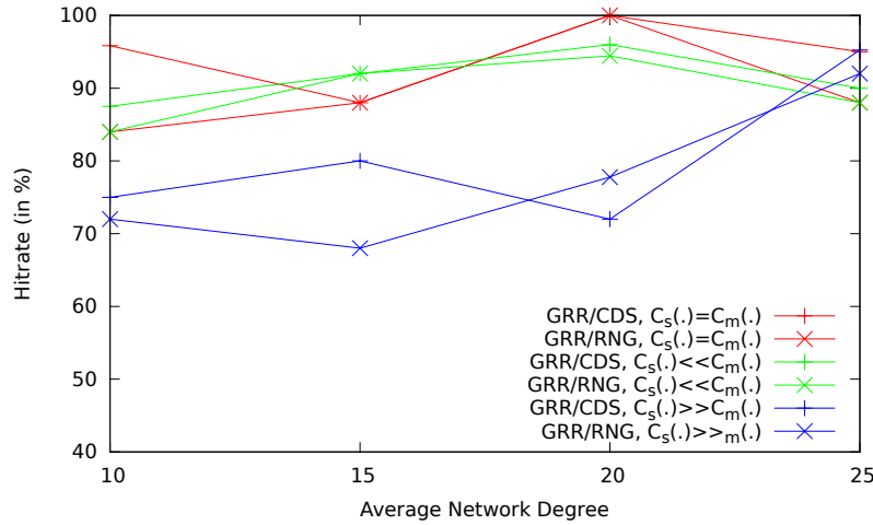
FIGURE 5.7 – Pourcentage de topologies où GRR route avec succès en fonction de \delta
