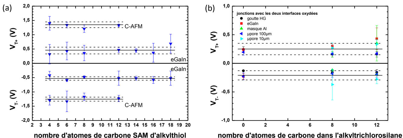
Figures 19 : Ensemble des tensions minimales V_{T+} et V_{T-} déterminées : (a) sur les SAMs d'alkylthiol par C-AFM (jonction sans oxyde) et par eGaln (avec une interface oxydée) ; (b) sur les jonctions de SAMs d'alkyltrichlorosilane avec les deux interfaces oxydées.
