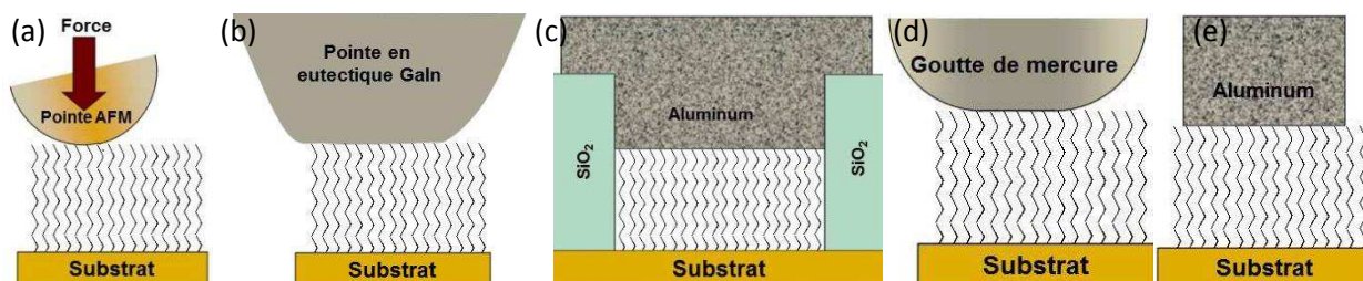
Figure 16 : Présentation schématique des différentes techniques utilisées pour caractériser électriquement les SAMs et former la jonction moléculaire : (a) par Conducting-AFM ; (b) Contact par eGaIn ; (c) Contact par goutte à mercure ; (d) Par plots d'aluminium formés par masque mécanique ; (e) Par micropore.
