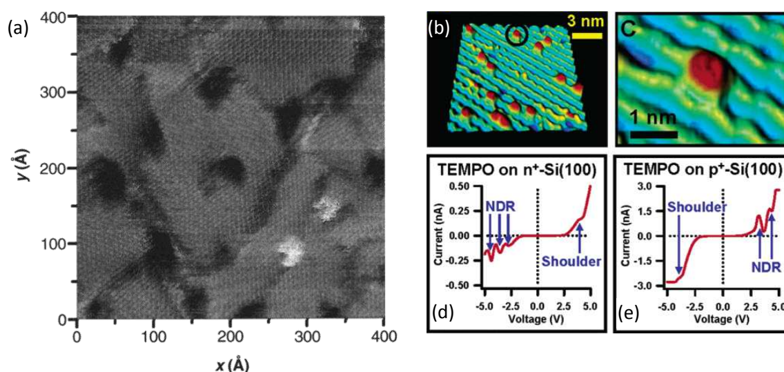
Figure 2 : (a) Image STM d'une couche mixte n-dodecanethiol avec des fils moléculaires (OPE oligophenylenevinylene) intercalés dans les défauts de la SAM de n-dodecanethiol 36 ; (b) Images STM d'une molécule de 2,2,6,6-tetraméthyl-1-piperidinyloxy (TEMPO) physisorbée sur une surface de silicium. Les courbes courant-tension mesurées sur la molécule de TEMPO sur du silicium dopé n (d) et p (e) sont tracées sous les images STM 38 .
