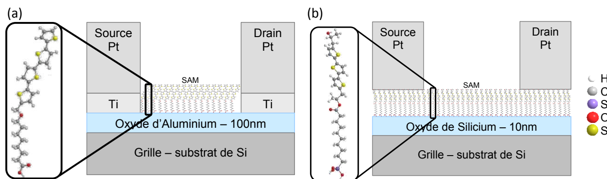
Figure 26 : Présentation schématique des deux structures comparées ici : (a) une structure bottom contact avec la SAM à base de quaterthiophène formée après les électrodes, et avec comme isolant de grille 100 nm d'alumine ; (b) une structure top contact avec la SAM à base de terthiophène formée avant les électrodes et avec comme isolant de grille 10 nm de SiO 2 .
