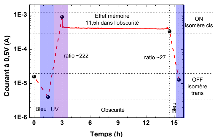
Figure 41 : Courant mesuré à 0,5\text{V} en fonction du temps pour différentes expositions lumineuses : en bleu pendant 90\text{min} , UV pendant 90\text{min} , dans l'obscurité pendant 11,5\text{h} et finalement en bleu pendant 60\text{min} .
