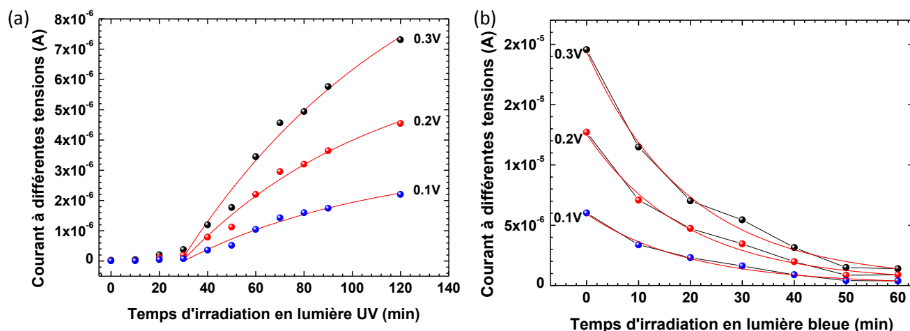
Figure 40 : Evolution en fonction du temps du courant mesuré par eGaN à différentes tensions ( 0,3\text{V} ; 0,2\text{V} et 0,1\text{V} ) et après exposition lumineuse : (a) par UV à 360\text{nm} , passage de l'isomère trans à cis ; (b) et par lumière bleue à 480\text{nm} passage de l'isomère cis à trans . Les lignes rouges correspondent à l'ajustement par une loi exponentielle pour déterminer les temps caractéristiques des cinétiques.
