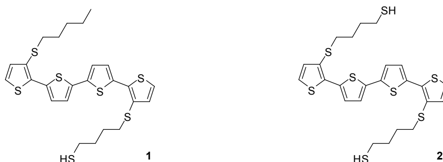
Figure 28 : Schéma des deux molécules synthétisées 176 pour cette étude, basées toutes deux sur un quaterthiophène avec un (1) ou deux (2) chaînes alkanethiol attachée(s) en position β par une liaison sulfure sur le (les) anneau(x) de thiophène externe(s).
