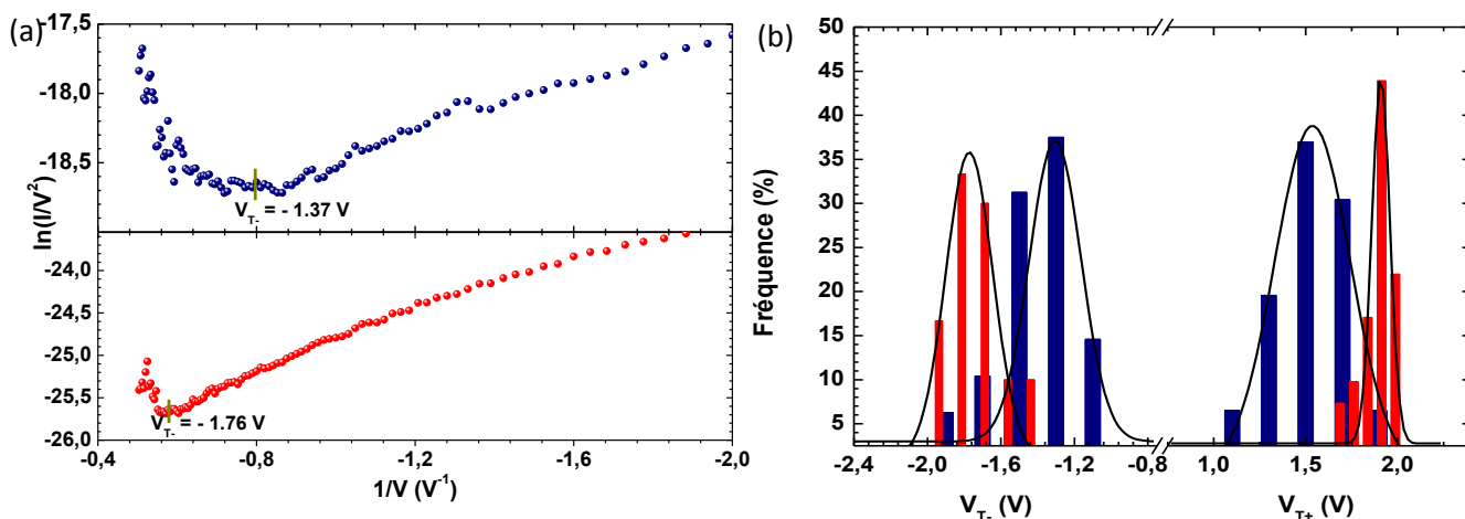
Figure 42 : (a) Exemple de courbes TVS à partir de mesures par C-AFM afin de déterminer le V_{T-} pour les deux isomères cis (•) et trans (•). (b) Histogramme des V_{T-} obtenus sur les mesures par C-AFM pour les tensions positives et négatives ainsi que pour la SAM en configuration cis (■) et trans (■).
