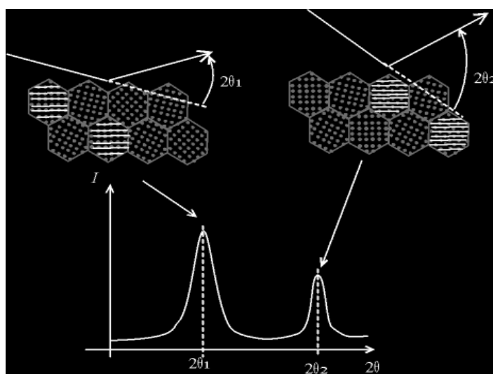
Figure II-7 Principe de la caractérisation par diffraction des rayons X [12].
