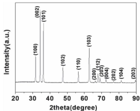
Figure II-8 Exemple de diffractogramme de nanotubes de ZnO en faisceaux faisant apparaître une structure hexagonale [13].
