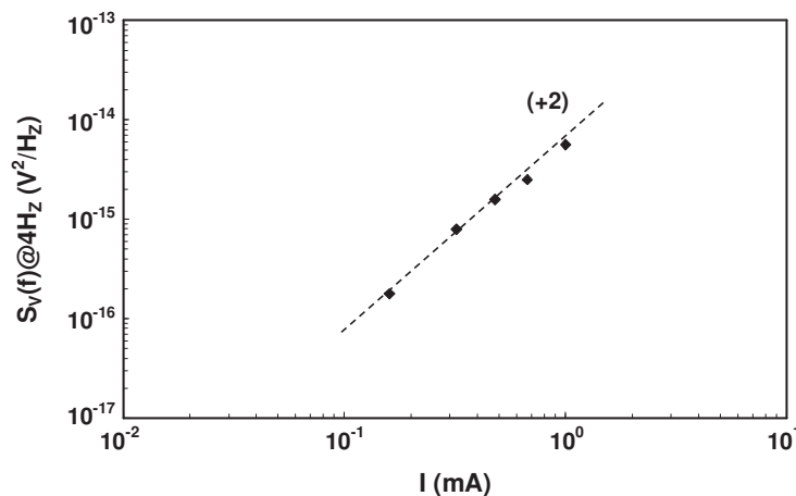
Figure III-27 Evolution de S_V(f) à 4Hz en fonction du courant continu I appliqué sur une couche déposée à 400 °C sur un substrat de Pt/Si en utilisant un plot de diamètre 0,2 mm (cf. Annexe No.25).
