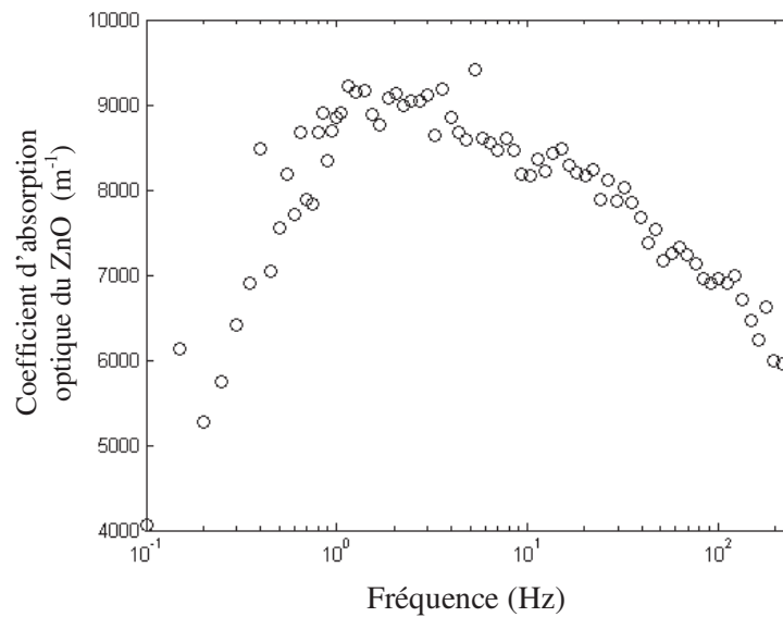
Figure IV-20 Evolution expérimentale du coefficient d'absorption optique \beta_l du ZnO obtenue par l'approximation analytique de l'expression du signal normalisé à basse fréquence.
