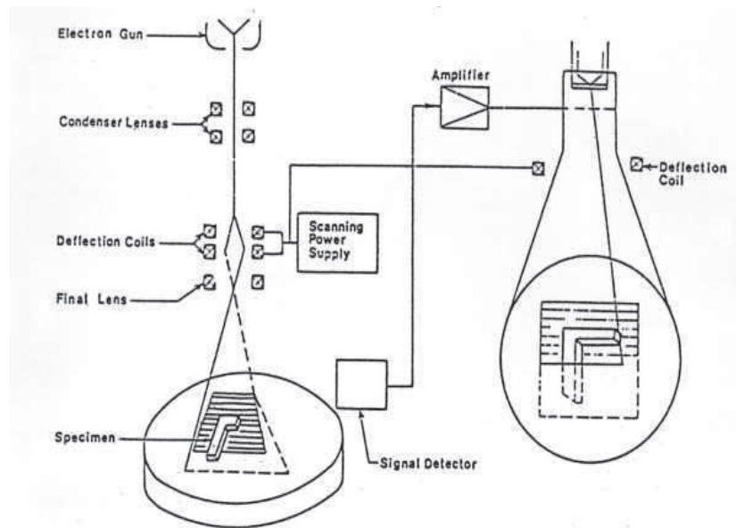
Figure II-4 Schéma de principe d'un microscope électronique à balayage [9].
