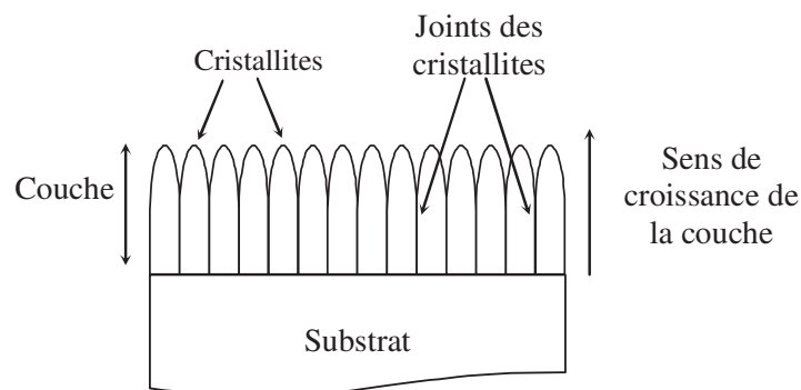
Figure I-10 Représentation de la structure cristalline du ZnO orientée perpendiculairement à la surface du substrat [30].
