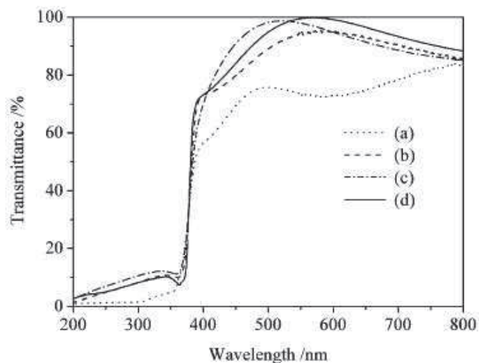
Figure I-14 Evolution de la transmission sur une couche mince de ZnO déposée sur un substrat de quartz à différentes températures et différentes pressions d'oxygène en fonction de la longueur d'onde : (a) 200 °C, 0,05 Pa ; (b) 200 °C, 20 Pa ; (c) 700 °C, 0,05 Pa et (d) 700 °C, 20 Pa [3].
