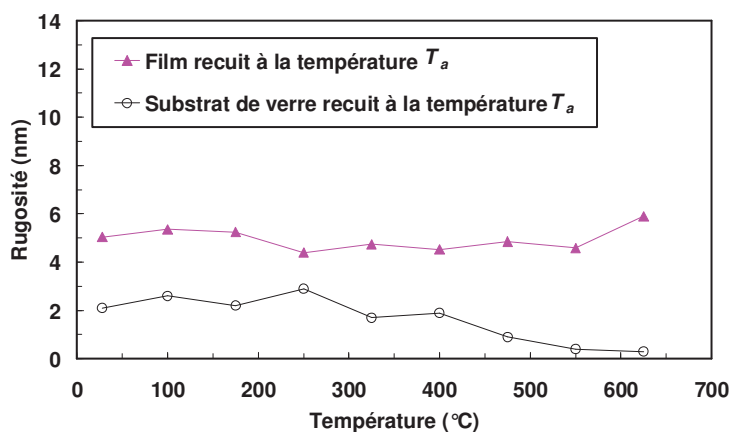
Figure II-19 ZnO sur verre : évolution de la rugosité de la surface des films déposés à l'ambiante en fonction de la température de recuit T_a à l'air (cf. Annexe No.6-14).
