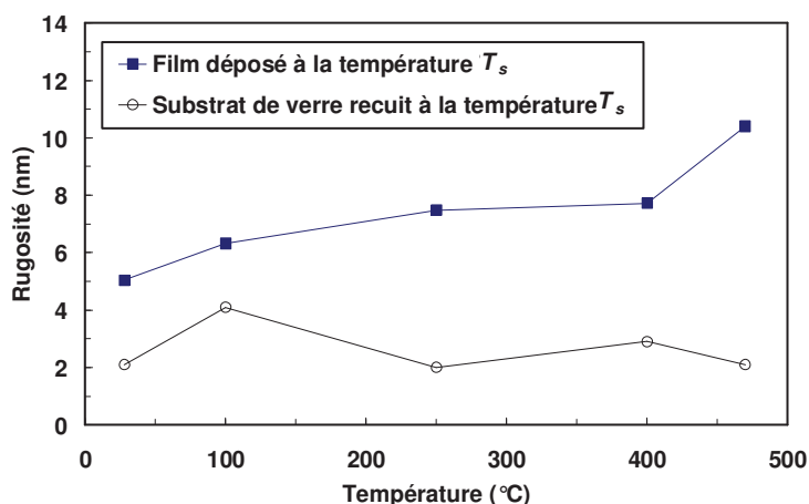
Figure II-13 ZnO sur verre : évolution de la rugosité de surface des films en fonction de la température de dépôt T_s (cf. Annexe No.6 et No.18-21).
