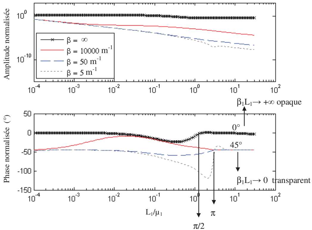
Figure IV-17 Simulation sur l'évolution de l'amplitude et la phase du signal normalisé en fonction du rapport \frac{L_1}{\mu_1} pour différentes valeurs du coefficient d'absorption optique \beta_l du ZnO.
