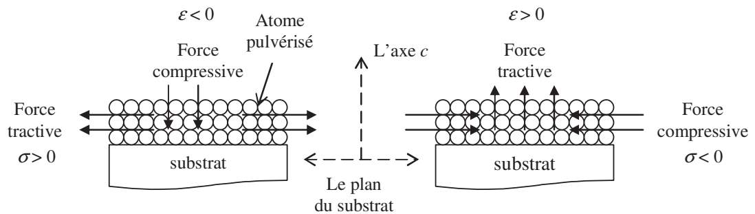
Figure II-11 Schéma des contraintes subies dans le matériau.
