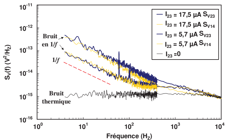
Figure III-13 Comparaison des spectres de bruit effectués sur un échantillon de ZnO déposé sur un substrat de verre à 400 °C (cf. Annexe No.20) pour 2 configurations de mesure :
