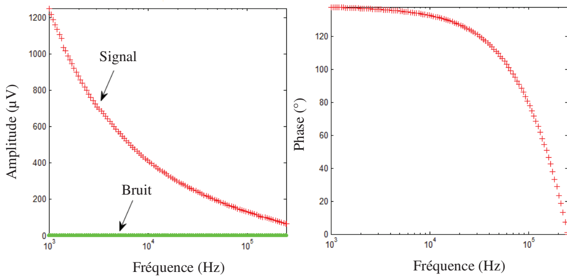
Figure IV-13 Evolution de l'amplitude et la phase du signal mesuré sur le carbone vitreux à haute fréquence (1 Hz - 100 kHz).
