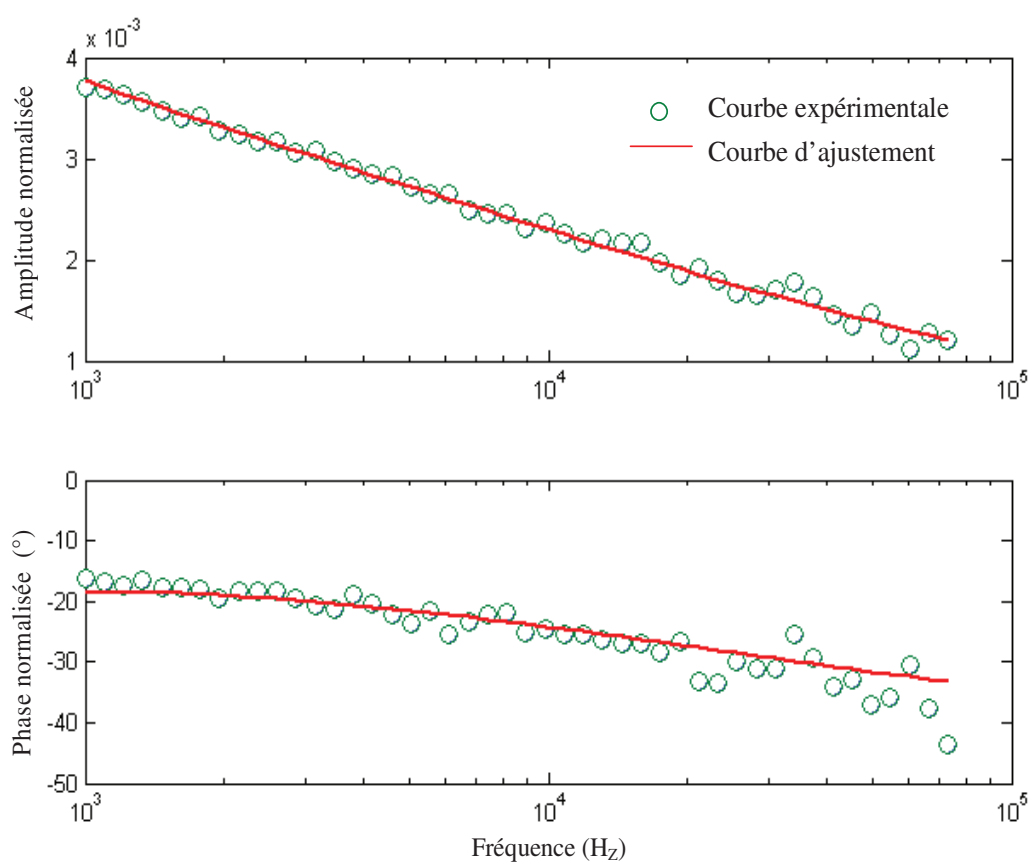
Figure IV-14 Evolution de l'amplitude et la phase du signal normalisé à haute fréquence (1Hz - 100 kHz). La courbe verte (o) représente les points expérimentaux et la courbe rouge (trait continu) représente l'ajustement numérique.
