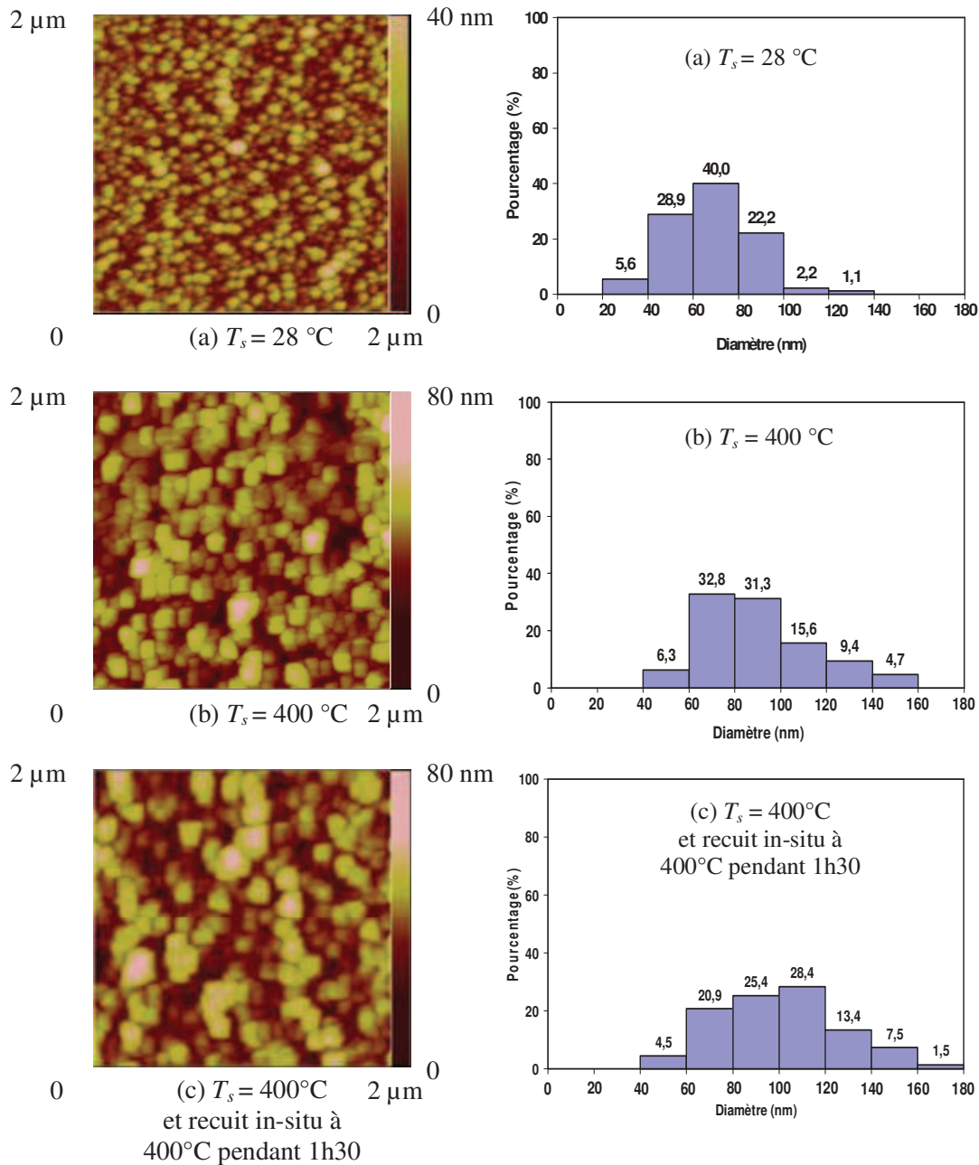
Figure II-22 ZnO sur verre : images AFM et distribution du diamètre des particules analysées par AFM pour le dépôt à : (a) T_s = 28\text{ °C} ; (b) T_s = 400\text{ °C} ; (c) T_s = 400\text{ °C} et recuit in-situ à 400\text{ °C} pendant 1h30 (cf. Annexe No.6 No.20 No.22).
