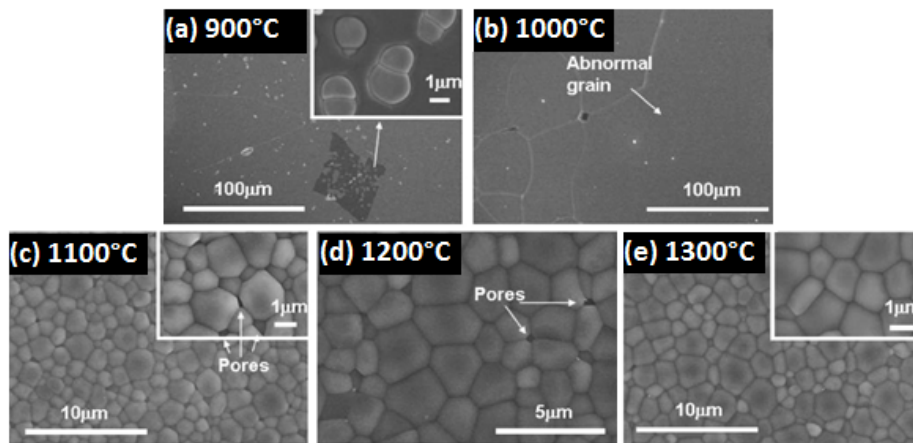
Figure 35 : Images MEB des céramiques obtenues après frittage à 1700 °C de poudres calcinées à différentes températures : 900°C (a), 1000°C (b), 1100°C (c), 1200°C (d) et 1300°C (e) [89]
