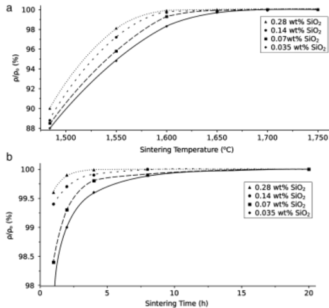
Figure 97 : Densités relatives en fonction de la température (a) et du temps de maintien (b) dans le cas du frittage naturel de Nd:YAG en présence de \text{SiO}_2 : 0,035 %, 0,07 %, 0,14 % et 0,28 % [150]
