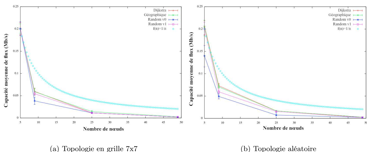
FIGURE 3.3.: capacité du flux vs routage et cardinalité : la passerelle est placée au centre du réseau
