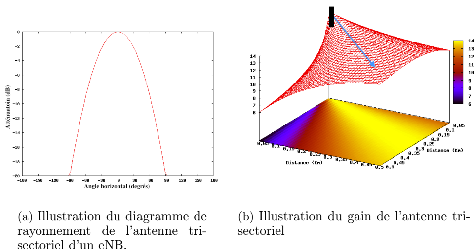
FIGURE 6.5.: Illustration de la fonction d'atténuation et du gain de l'antenne tri-sectorielle.
