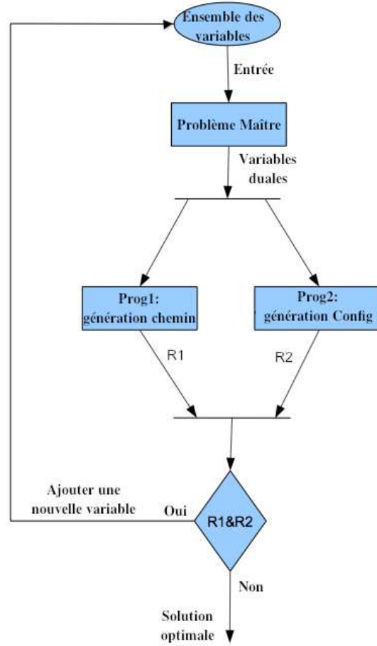
FIGURE 4.5.: Processus de génération de colonnes
