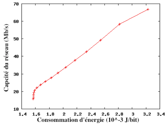
FIGURE 6.9.: Compromis capacité-énergie pour un réseau cellulaire composé de eNB, 30RNs et 40UEs dans un milieu rural.
