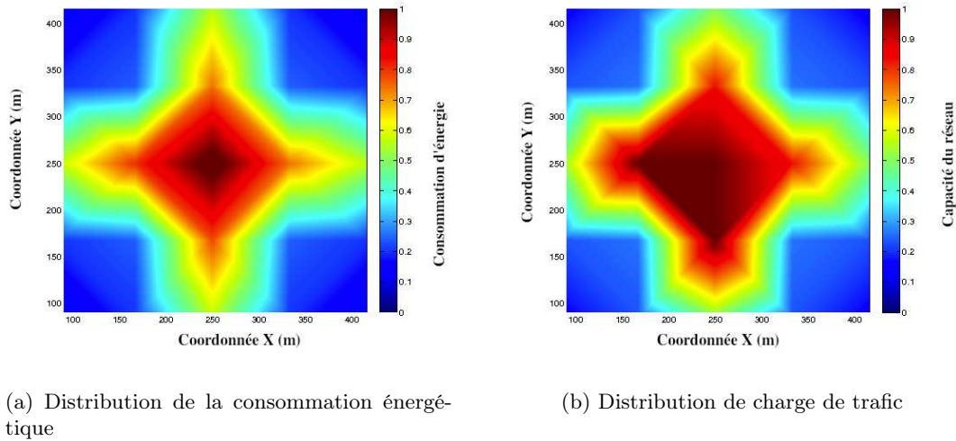
FIGURE 5.13.: Distribution de la consommation énergétique et de la charge de trafic dans un réseau en grille.
