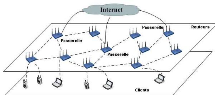
FIGURE 3.1.: Architecture du réseau maillé sans fil : les points d'accès collectent le trafic de clients mobile/fixe et l'envoient vers Internet à travers des passerelles.
