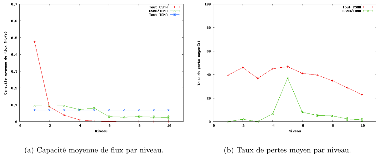
FIGURE 3.14.: L'apport, en performances du réseau, d'un ordonnancement TDMA de 4 niveaux avec augmentation de nombre de slots.
