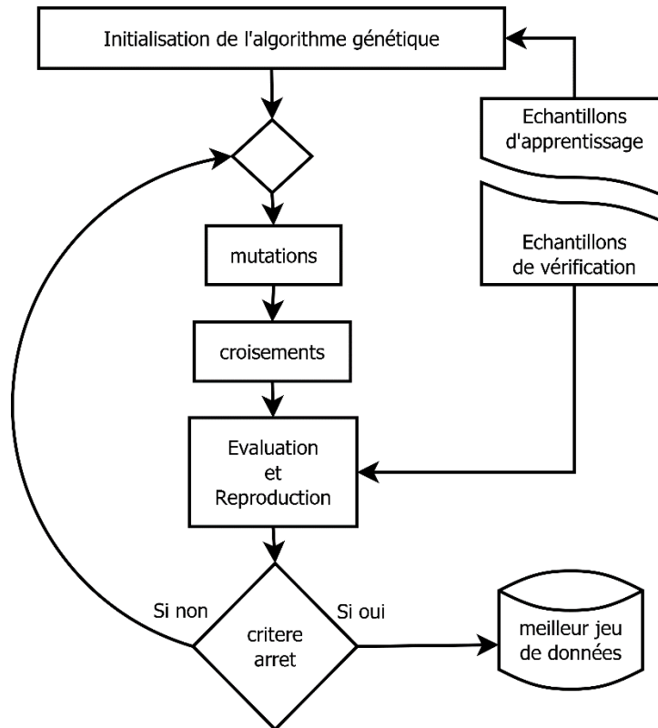
figure III.2 : Schéma d'exécution des Algorithmes Génétiques
