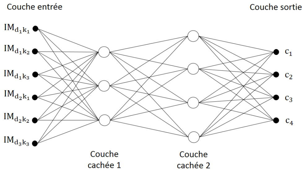
figure I.26 : Exemple de perceptron à deux couches cachées avec en entrée les images par date et par canal et en sortie une décision sous forme d'attribution de classe de l'ensemble C.
