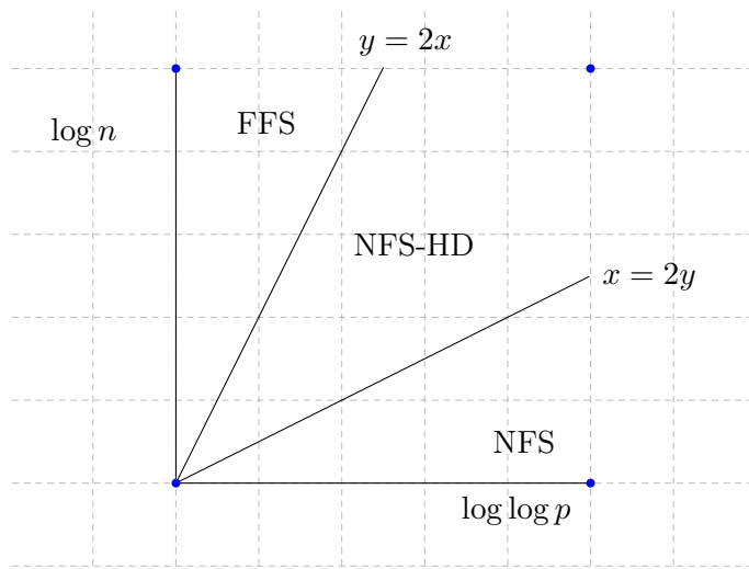
FIGURE 1: Le domaine d'application de FFS, NFS-HD et NFS selon \mathbb{F}_Q^* avec Q = p^n .
