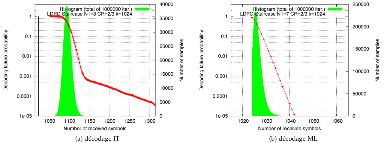
Figure 5.1: \text{Pr}_{\text{echec}} = f(\text{overhead}) en IT (avec N_1 = 3 ) et ML (avec N_1 = 5 ) des codes LDPC-Staircase avec ( k = 1024 , \text{CR} = 2/3 et G = 1 ).
