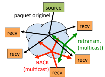
Figure 10.1: Mécanisme de retransmission avec SRM.
