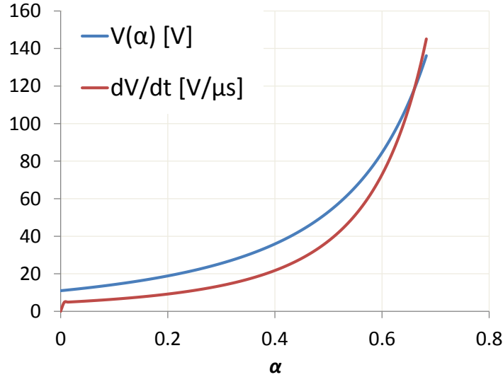
FIGURE 3.6 – Courbe de tension et sa dérivée en fonction du paramètre \alpha = \frac{t}{t_0} .
