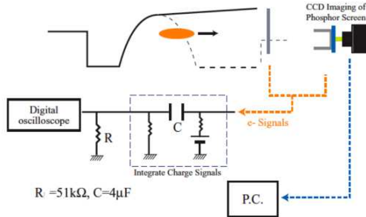
FIGURE 4.20 – Chaîne de détection des paramètres d'un plasma d'électrons. La charge est collectée sur l'écran phosphore. Le circuit de découplage permet de récolter la charge sur l'oscilloscope tout en appliquant une haute tension sur l'écran phosphore. La lumière générée par l'accélération des charges sur l'écran phosphore est recueillie par une caméra CCD pour obtenir le rayon du plasma d'électrons. Extrait de [Dupré 2011].
