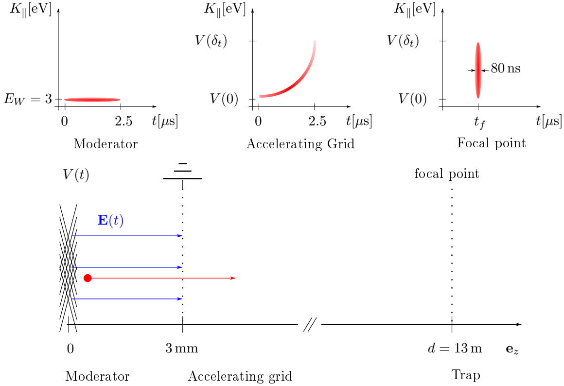
FIGURE 3.5 – Transformation de l'espace des phases du faisceau par application d'un potentiel dynamique sur le modérateur. L'espace des phases initial (à gauche) est modifié par l'application de la fonction (3.11) sur le modérateur. L'espace des phases au niveau de la grille de masse (au centre) montre la dispersion en énergie introduite par l'application de la fonction (3.11). Cette dispersion en énergie permet la réduction de la distribution temporelle au point focal (à droite).
