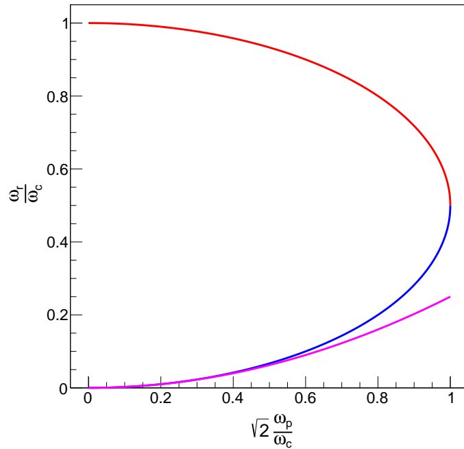
FIGURE 2.4 – Pulsation de rotation du plasma \omega_r en fonction de la pulsation plasma \omega_p . Les solutions \omega_- et \omega_+ sont représentées respectivement en bleu et rouge. La courbe rose indique la solution approximée \omega_E = \omega_p^2/2\omega_c .
