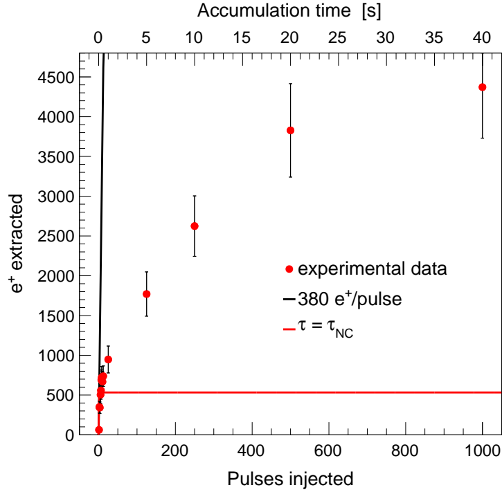
FIGURE 5.19 – Nombre de positons piégés en fonction du nombre de pulses injectés. La croissance du signal met en évidence l’accumulation des pulses. La ligne noire montre la valeur attendue dans des conditions optimales. La ligne rouge montre l’accumulation limite des charges si la durée de vie des charges \tau = \tau_{NC} est la même que lorsque le refroidissement n’est pas mis en œuvre. La mesure est réalisée à 25 Hz : 1000 pulses correspondent à 40 secondes d’accumulation. L’augmentation du nombre de charges n’est pas linéaire et semble saturer avec le temps d’injection.
