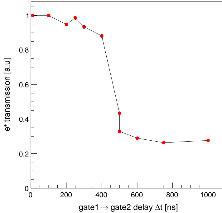
FIGURE 5.15 – Transition entre positons passants et positons piégés avec le délai \Delta t appliqué entre gate1 et gate2 . Au delà de 500 ns (durée d’ouverture de gate1 ), la fraction de flux mesurée correspond à des positons piégés. La fraction de flux obtenue est alors égale à l’efficacité de compression \eta_B = 25\% dans une fenêtre de 80 ns.
