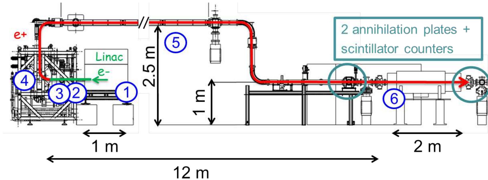
FIGURE 4.1 – Injecteur de positron de Saclay. (1) Linac d'électrons de 4.3 MeV avec un taux de répétition allant de 20 à 200 Hz, un courant crête d'électrons de 140 mA et une durée effective de pulse de 2.5 \mu s; (2) Convertisseur e^- \rightarrow e^+ constitué d'une plaque de tungstène de 1 mm de large; (3) Modérateur en tungstène qui diminue l'énergie du faisceau de e^+ dans la gamme de l'électronvolt; (4) Séparateur magnétique e^+/e^- SOPHI ; (5) Ligne de transport faisceau de 16 m de long constituée de solénoïdes produisant un champ magnétique de 8 mT; (6) Piège de Penning-Malmberg du RIKEN constitué de 27 électrodes dans un champ magnétique de 5 T produit par un aimant supraconducteur.
