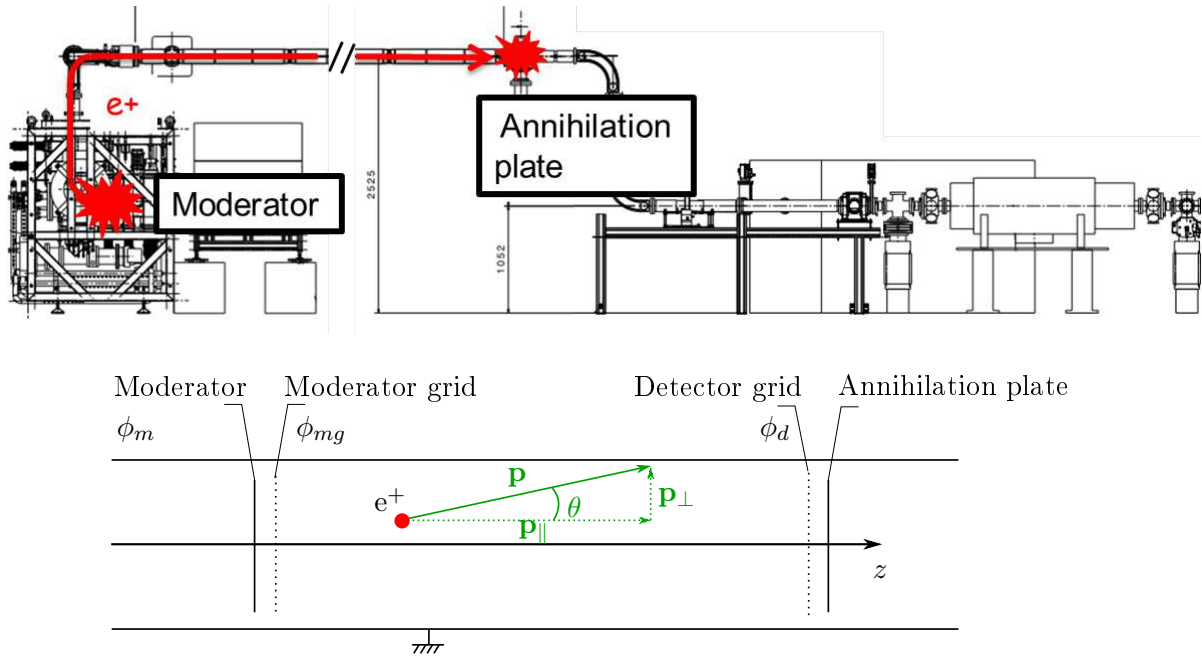
FIGURE 5.4 – En haut, dessin de la ligne faisceau présentant la position du détecteur où est réalisée la mesure. En bas, dessin schématique des différents éléments intervenant dans la mesure.
