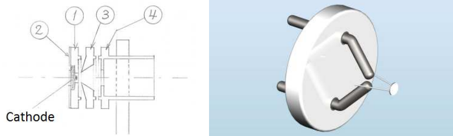
FIGURE 4.18 – A gauche, Schéma du canon à électron : 1. support, 2. plan arrière, 3. électrode extractrice, 4. anode à la masse. Schéma extrait de [Mohri 2012]. A droite, vue conceptuelle de la cathode.
