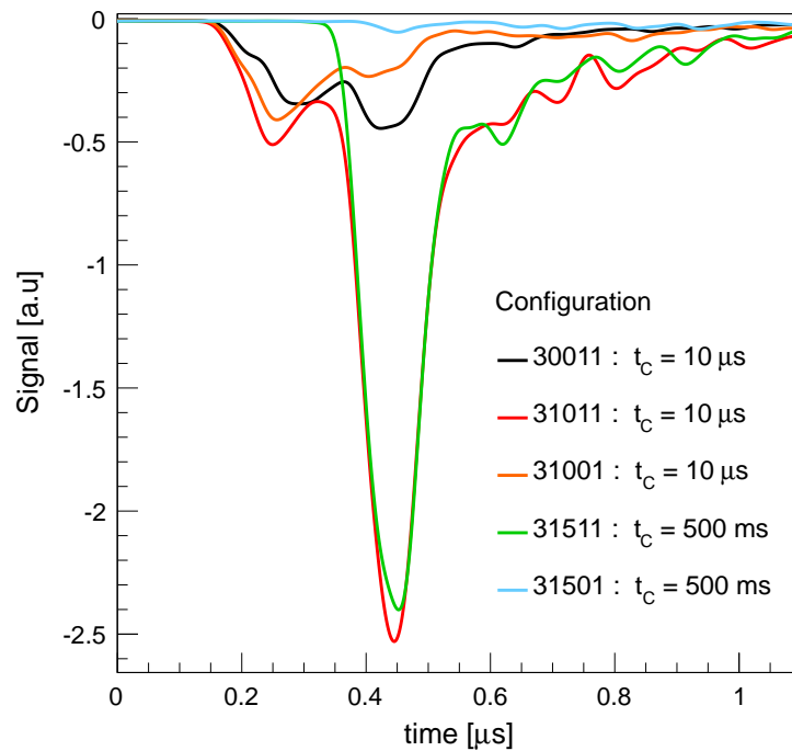
FIGURE 5.23 – Signal d'éjection des positons piégés dans différentes configurations de confinement, présentées dans le tableau 5.6. Les traces sont lissées pour améliorer la visibilité. Le temps d'accumulation est de 20 s, excepté dans la configuration 30011 où il est de 3 s.
