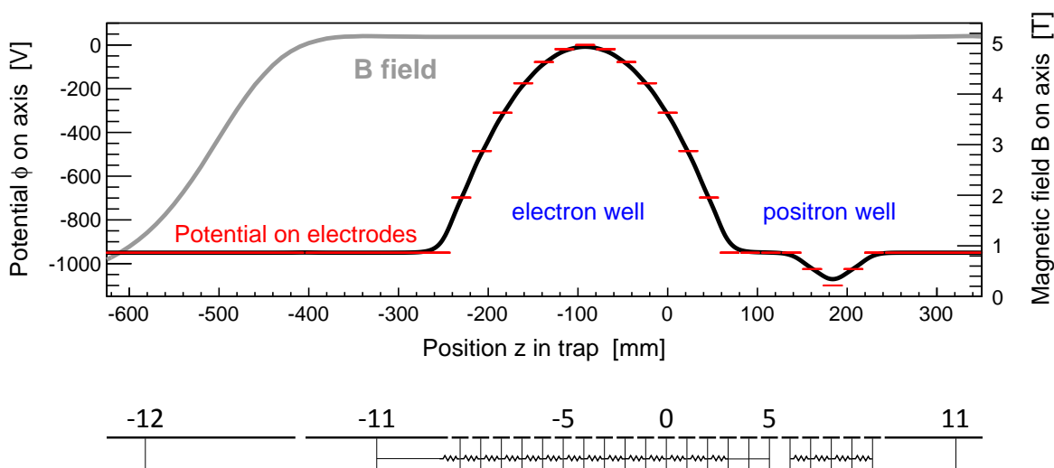
FIGURE 4.16 – Profil électromagnétique dans le piège avec deux puits de potentiel. Les électrodes et les ponts de résistances sont représentés à l'échelle sous le profil. Le premier pont de résistances correspond au puits d'électrons et le second au puits de positons. Le potentiel appliqué sur les électrodes est représenté en rouge. Le champ magnétique est représenté en gris (échelle à droite de la figure).
