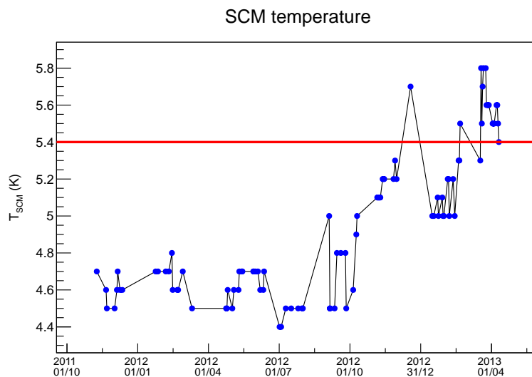
FIGURE 4.14 – Température de l'aimant mesurée au multimètre en fonction du temps. Les périodes d'arrêt du système cryogénique ne sont pas montrées pour plus de clarté. La ligne rouge correspond à la température maximale pour fonctionner à 5 T.
