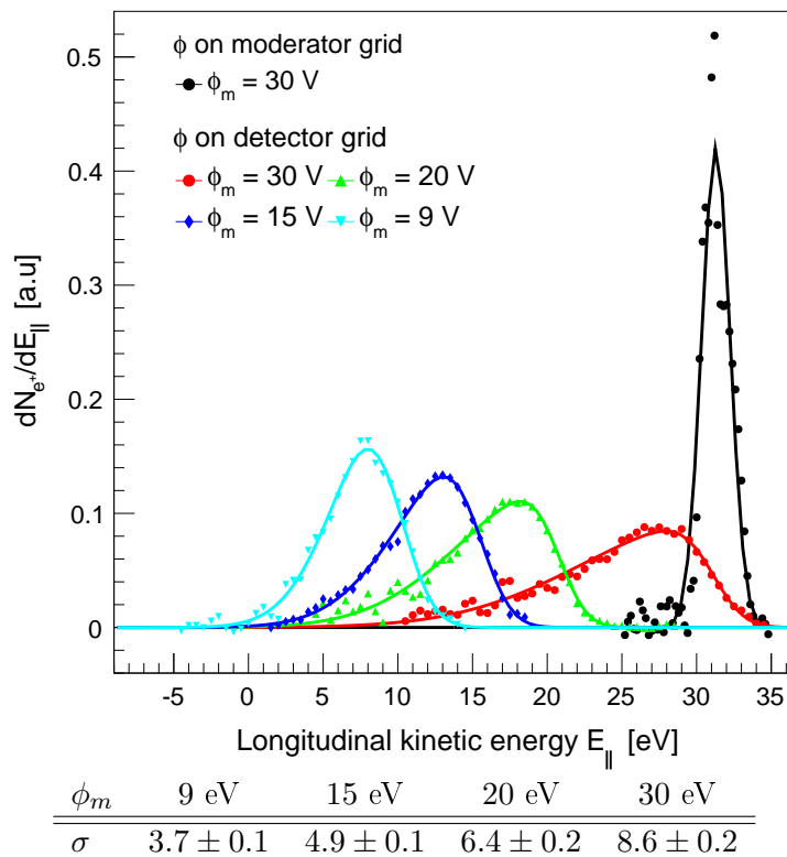
FIGURE 4.12 – Distribution en énergie longitudinale du faisceau de positons lents dans la ligne de transport en fonction de différents biais \phi_m appliqués sur le modérateur. L'énergie est mesurée par application d'un potentiel retardé \phi (voir la partie 5.3 page 80). Alors que l'écart type est de \sim 1 eV au niveau du modérateur (en noir), la distribution est très élargie au niveau du détecteur. L'élargissement de la distribution augmente avec le potentiel initial \phi_m porté sur le modérateur.
