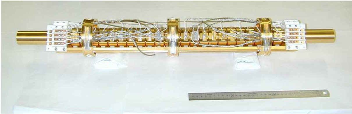
FIGURE 4.15 – Photo du bloc central des électrodes du piège du RIKEN.
