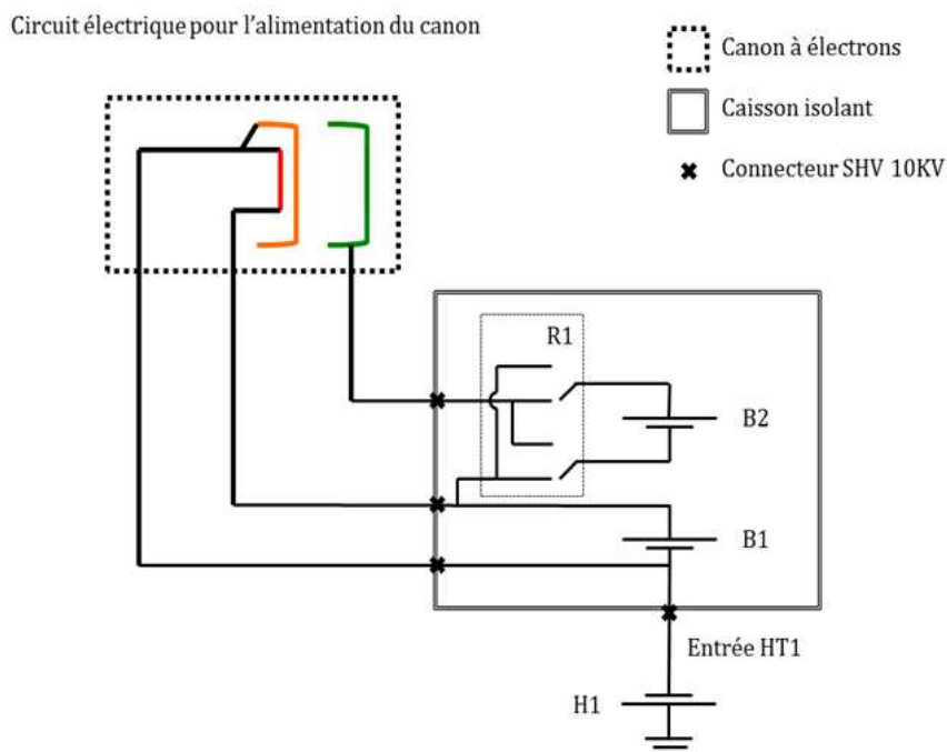
FIGURE 4.19 – Schéma électrique d'alimentation du canon à électrons. La cathode est représentée en rouge et l'anode en vert. Lorsque le relai R1 est activé dans le caisson haute tension, la polarité de l'électrode d'extraction est inversée. Extrait de [Dupré 2011].
