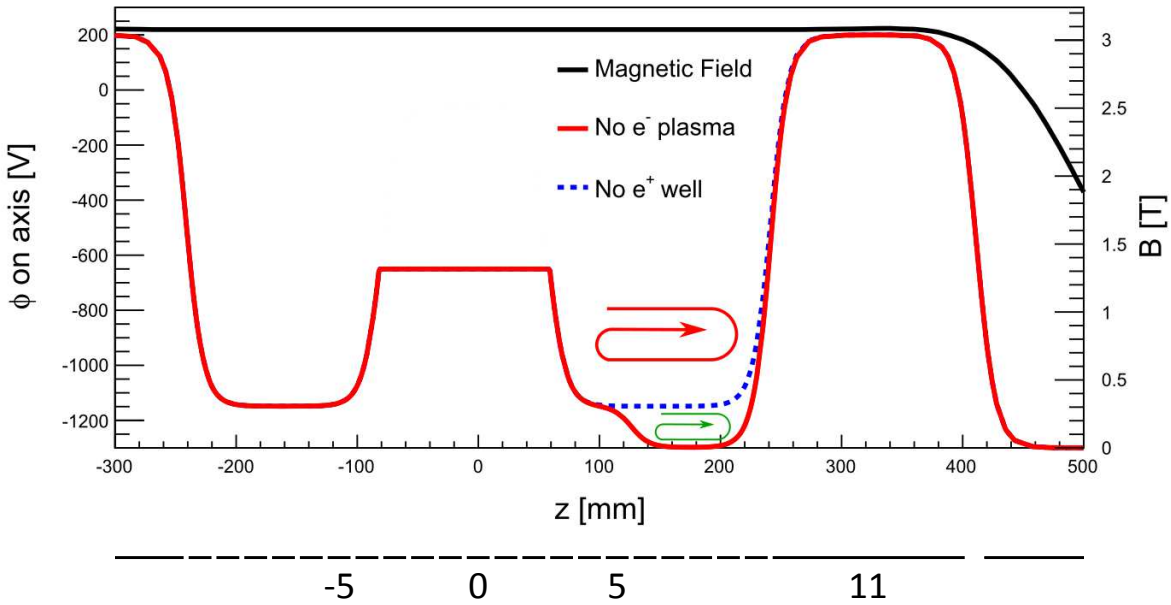
FIGURE 5.24 – configuration 3 modifiée. Lorsque l'on teste l'accumulation de positons sans plasma d'électrons, le potentiel plasma est simulé en changeant le biais sur les électrodes du puits d'électrons. Lorsque l'on supprime le puits de positons, on applique un potentiel plat dans la région du puits, à \phi_{inj} = -1150 V. Les zones de confinement supposées des deux signaux de positons mesurés sont représentées par une flèche rouge (pic 1) et une flèche verte (pic 2). La région couvrant l'intégralité de la longueur du piège est éliminée car le potentiel porté sur gate1 laisse sortir les positons vers l'amont du piège dans la configuration d'injection.
