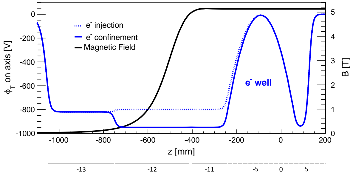
FIGURE 5.1 – Profil de potentiel \phi_T produit par les électrodes sur l'axe pour le confinement du plasma d'électrons ( configuration 1 ). La courbe noire montre le champ magnétique sur l'axe. Les électrodes produisant le champ sont indiquées sous le graphique ( -13 à +8 ). Le puits de potentiel est formé entre l'électrode -11 et les électrodes 3 , 4 et 5 ( L = 320 mm). Le potentiel de l'électrode -12 est relevé pour permettre aux électrons de pénétrer dans le puits en phase d'injection. La différence de potentiel entre le fond du puits et le bord du puits à l'injection est de 800 V (le fond du puits est connecté à la masse). Le canon à électrons est situé à \sim 150 mm en amont de l'électrode -13 .
