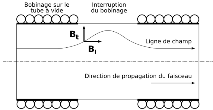
FIGURE 3.10 – Schématisation d’une interruption de champ entre deux bobinages de solénoïdes. Le champ magnétique homogène et parallèle dans le solénoïde marque une bosse dans la région de l’interruption de bobinage. Dans la ligne de transport, la variation de l’intensité du champ magnétique sur l’axe peut atteindre 20 %, pour une intensité du champ dans le solénoïde de \sim 10 mT. La taille caractéristique d’une interruption est de 100 mm. Extrait de [Ruiz 2011].
