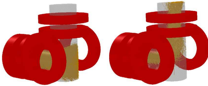
FIGURE 4.6 – Trajectoires des électrons (à gauche) et des positons (à droite) dans le séparateur e^+/e^- . Les particules chargées se propagent de gauche à droite. La configuration magnétique permet de défléchir les électrons et les positons dans des directions opposées. Le faisceau d'électrons est défléchi par le dipôle (bobines horizontale D1 et D2) dans la direction opposé à la direction de champ privilégié créé par le champ solénoïdale des bobines entourant le tube faisceau : le faisceau est éclaté dans la chambre. Au contraire, le dipôle favorise le transport des positons vers la sortie de la chambre à vide (vers le haut).
