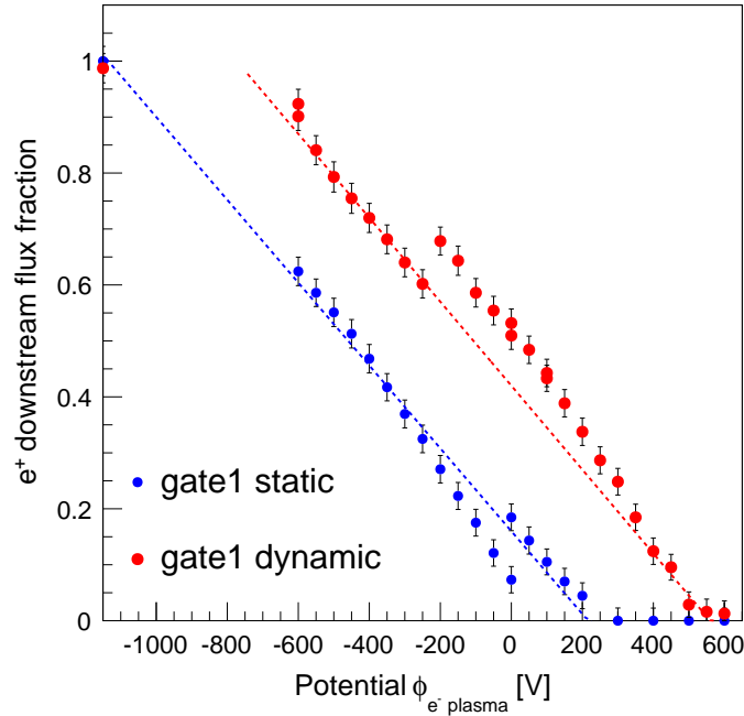
FIGURE 5.12 – Influence d'une barrière de potentiel sur la transmission dans le piège. On détecte le flux de positons sur l'écran phosphore en fonction de la barrière de potentiel portée sur les électrodes -2 à +3 . La distribution en énergie parallèle des positons qui ont franchi le miroir est alors quasi-constante. Les discontinuités que l'on observe sont dues à des défauts pendant la mesure : un arrêt du linac (points rouges) et l'inversion de polarité de la barrière de potentiel (points bleus).
