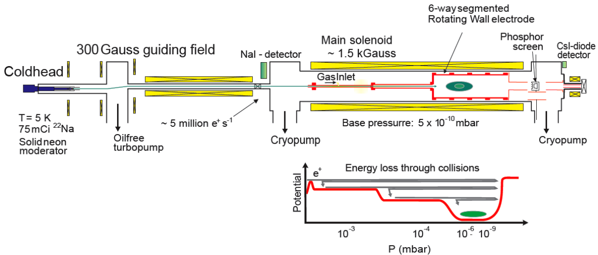
FIGURE 3.1 – Schéma de principe d'un accumulateur par refroidissement avec gaz tampon de \text{N}_2 .
