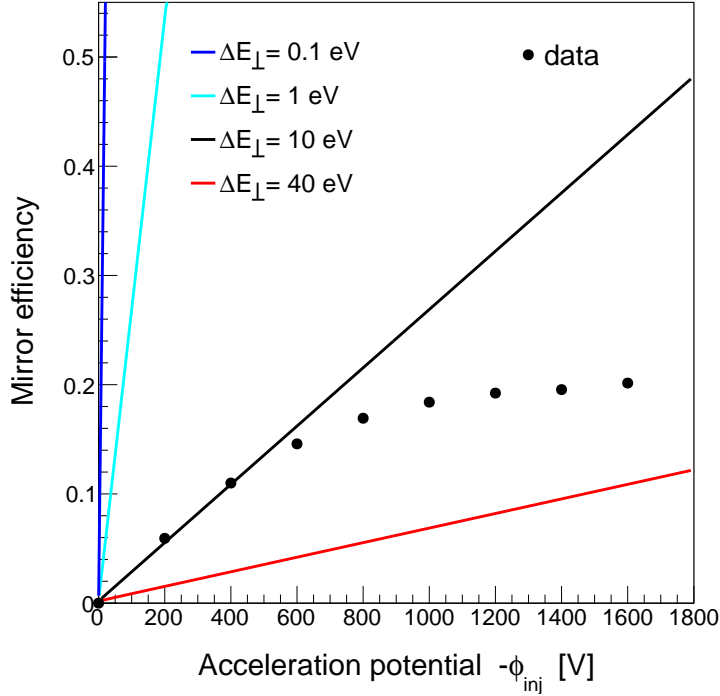
FIGURE 5.11 – Transmission dans le miroir magnétique. La mesure correspond aux cercles pleins noirs. Chaque point correspond à la transmission, rapport du flux détecté en aval sur le flux en amont du piège, mesurée pour un potentiel d'accélération donné. Les droites représentent la fonction donnée à l'équation (5.12) pour différentes valeurs de \Delta E_{\perp} . Avec l'élargissement de la distribution en énergie de la distribution comprimée en temps, on s'attend à une largeur \Delta E_{\perp} comprise entre 7 eV et 35 eV, ce qui correspond à la mesure.
