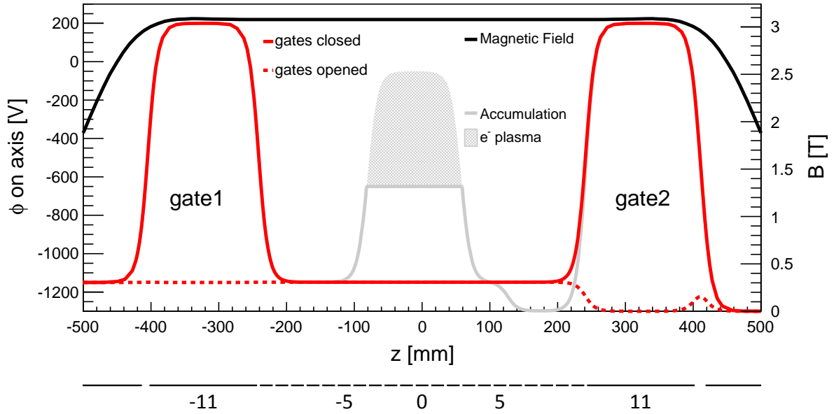
FIGURE 5.13 – Profil de potentiel \phi sur l'axe pour le piégeage des pulses de positons. Les électrodes -10 à +10 sont portées au potentiel de -1150 V. gate1 bascule entre -1150 V et 200 V pour passer de la configuration d'injection à la configuration de confinement des positons ; gate2 bascule entre 200 V et -1300 V pour passer du confinement à l'extraction des positons. Le profil de potentiel qui sera utilisé lors de l'accumulation ( configuration 3 ) est montré en grisé.
