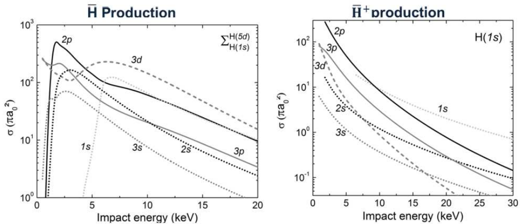
FIGURE 1.3 – A gauche : sections efficaces de formation de \bar{\text{H}} dans les niveaux 1s à 5d en fonction de l'énergie incidente des antiprotons, pour différents niveaux d'excitation du positronium. A droite : sections efficaces de formation de \bar{\text{H}}^+ en fonction de l'énergie incidente de \bar{\text{H}} dans l'état 1s, pour différents niveaux d'excitation du positronium. Données extraites de [Comini and Hervieux 2013].
