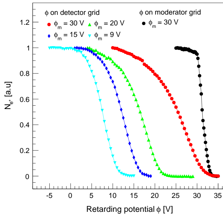
FIGURE 5.6 – Nombre de positons mesuré en fonction de la barrière de potentiel appliquée sur la grille devant le détecteur (en rouge, vert, bleu et cyan) et sur la grille du modérateur (noirs). Les données sont normalisées, les lignes sont des guides pour les yeux. Les cercles pleins noirs et rouges correspondent aux mêmes conditions initiales, \phi_m = 30 V.
