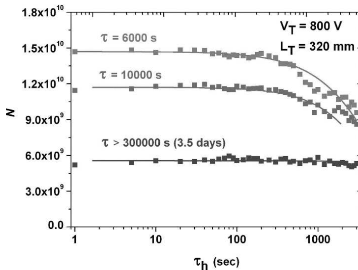
FIGURE 3.3 – Temps de vie des plasmas d'électrons dans le piège du RIKEN. Extrait de [Mohamed et al. 2013].
