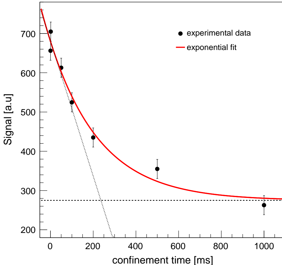
FIGURE 5.25 – Temps de vie des positons constituant le premier pic du signal d'extraction. L'ajustement des points de mesure expérimentaux avec la fonction (5.21) donne un temps de confinement \tau_C = 236 ms.
