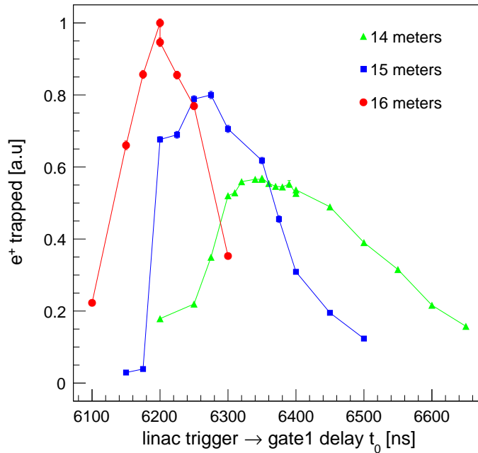
FIGURE 5.16 – Optimisation du délai t_0 entre le déclenchement du linac et la fermeture de gate1 . Les différentes couleurs correspondent à différentes valeurs de d dans la fonction de compression, de respectivement 14, 15 et 16 mètres (voir équation (5.9)).
