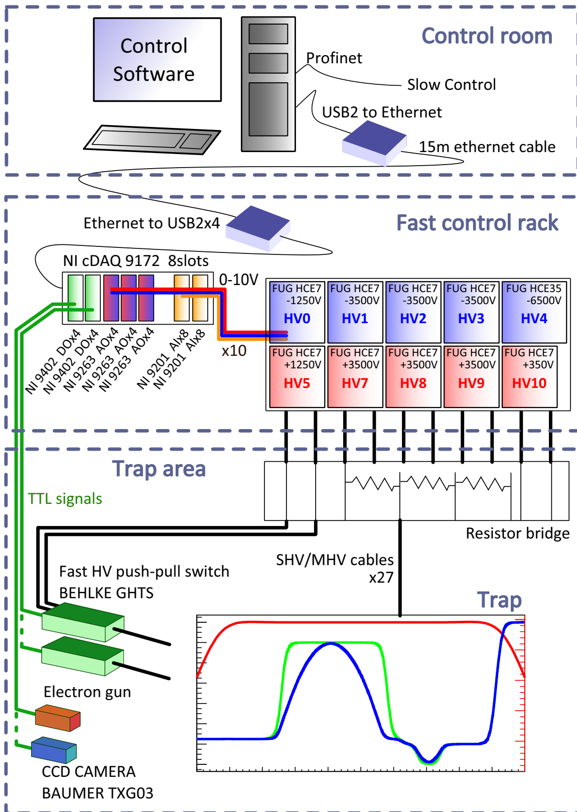
FIGURE 4.17 – Schéma simplifié du système d'acquisition et de contrôle des électrodes du piège ( fast control ).
