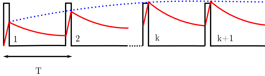
FIGURE 5.20 – Schéma descriptif de la saturation d'accumulation de charges. Un nombre constant de charges est injecté avec une période T , représenté en rouge. Le nombre de charge décroît suivant une loi exponentielle. La saturation du nombre de charge est montrée par la tendance en pointillée bleu.
