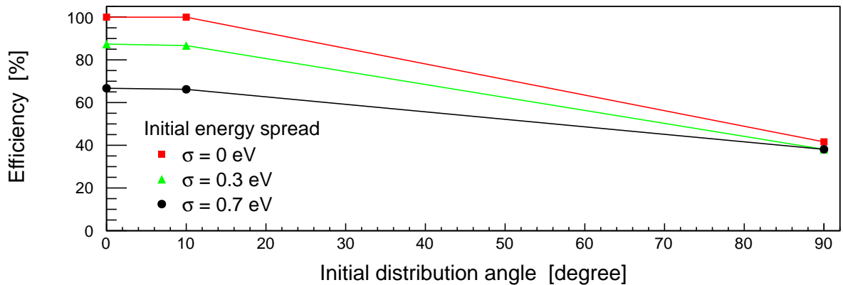
FIGURE 3.8 – Efficacité de compression en fonction de la distribution angulaire initiale. Chaque point correspond à un résultat de simulation, les lignes sont des guides pour les yeux. Pour chaque couleur, les 3 points correspondent à une distribution angulaire nulle, isotrope dans un cône d'angle \theta = 10^\circ , et isotrope (dans le demi espace aval du modérateur, soit \theta = 90^\circ ). La distribution en énergie initiale est une gaussienne d'écart type \sigma . Les différentes valeurs de \sigma simulées sont montrées par les différentes couleurs.
