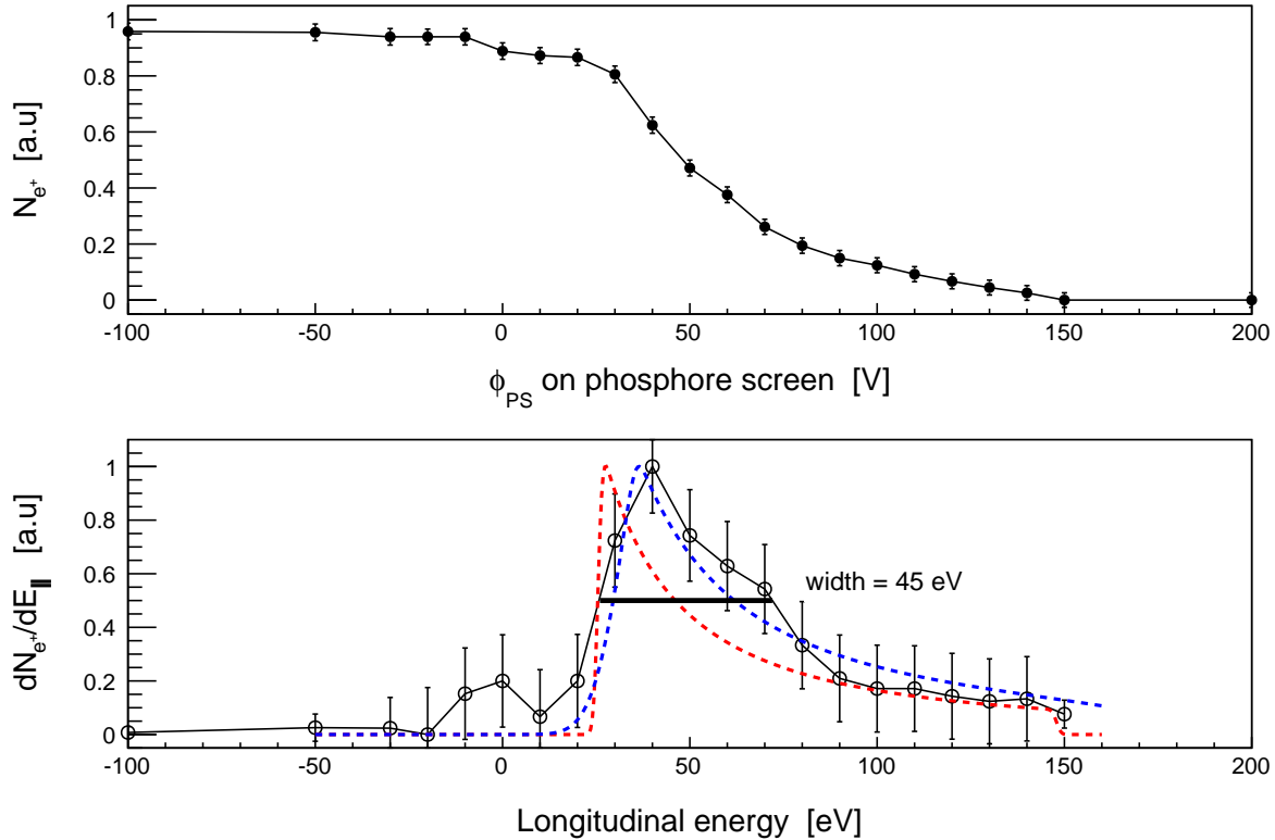
FIGURE 5.9 – Mesure de la distribution en énergie parallèle du faisceau de positons sur l'écran phosphore. La mesure est réalisée avec la méthode décrite dans la partie 5.3. Le graphique du haut présente le flux de positons détecté en fonction du potentiel appliqué sur l'écran phosphore. En dessous, les cercles représentent la distribution en énergie correspondant aux points de mesures. Les lignes pointillées montrent la distribution au modérateur (en rouge) et après transport (en bleu) en intégrant la fonction (5.6) sur la gamme de potentiel appliquée au modérateur. Les paramètres d'intégration \sigma et \alpha sont les paramètres présentés à la figure 5.7 pour la distribution au modérateur, et les modèles linéaires des équations (5.7) et (5.8) sont utilisés pour la distribution après transport. L'élargissement de la distribution mesurée est de 45 eV, compatible avec le modèle prenant en compte l'élargissement pendant le transport.
