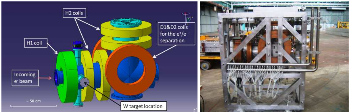
FIGURE 4.5 – Représentation schématique (à gauche) et photographie (à droite) du séparateur e^+/e^- .
