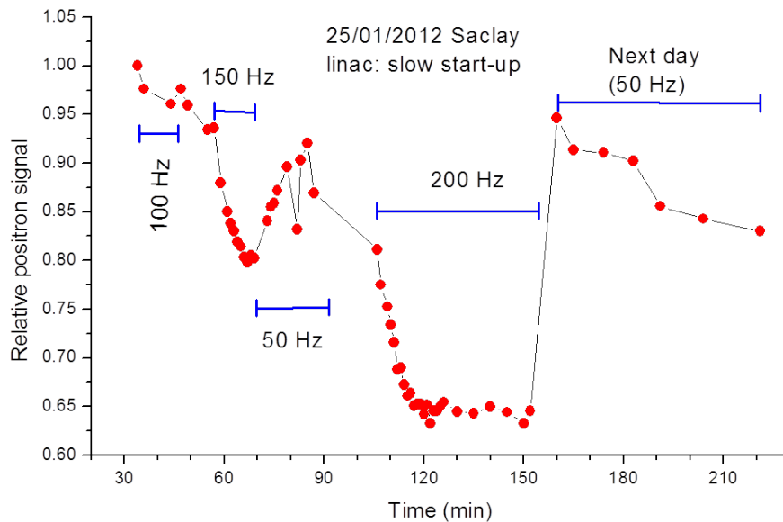
FIGURE 4.9 – Évolution de l'efficacité de modération en fonction du temps. La température du modérateur varie avec le temps d'utilisation et la fréquence du linac.
