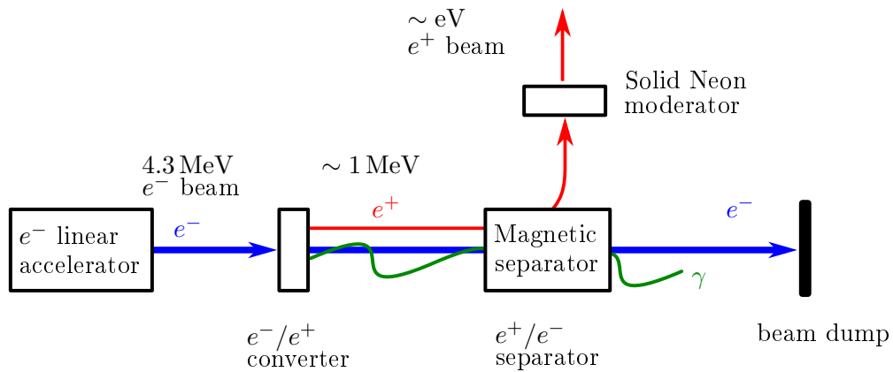
FIGURE 4.2 – Schéma du principe de production de positons lents pour GBAR.
