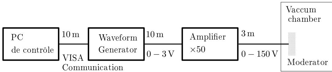
FIGURE 4.10 – Schéma du dispositif expérimental de compression du faisceau.
