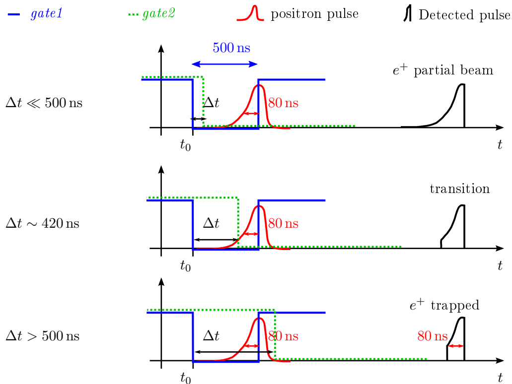
FIGURE 5.14 – Étapes du piégeage des positons pulse par pulse. gate1 est préalablement réglée pour se fermer pendant le passage du pulse, en fixant t_0 et sa durée d'ouverture à 500 ns. On s'assure ainsi de la présence de positons dans le piège, contenus à priori dans une fenêtre de 80 ns précédant la fermeture de gate1 . Le délai \Delta t d'ouverture de gate2 par rapport à gate1 est augmenté depuis 0 jusqu'à \Delta t > 500 ns. Le signal détecté, initialement égal à la fraction de flux transmise avant la fermeture de gate1 , réduit jusqu'au moment où gate2 n'est ouverte qu'après la fermeture de gate1 : le signal détecté correspond alors à des positons piégés.
