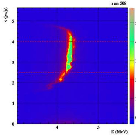
FIGURE 4.4 – Distribution d'énergie du faisceau d'électrons. En ordonnée, le temps en \mu\text{s} . En abscisse, l'énergie du faisceau en MeV. extrait de [Debu et al. 2011].
