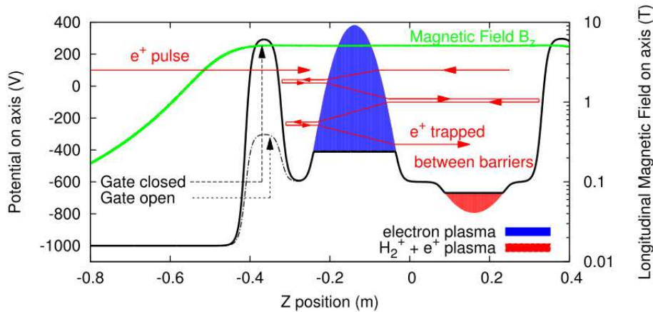
FIGURE 3.13 – Principe d'injection pulsé et de refroidissement des positons dans un plasma d'électrons. Extrait de [Dupré 2013].
