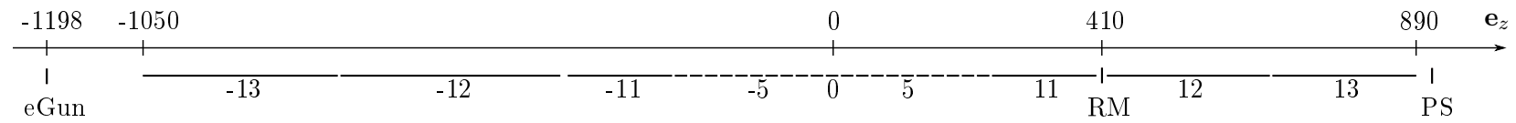
FIGURE 4.24 – Schéma des électrodes du piège à l'échelle. Le canon à électrons est schématisé par eGun, le remodérateur par le sigle RM et l'écran phosphore par PS. Les dimensions sont rapportées en mm. L'écran phosphore se trouve à 24 mm en aval de l'électrode 13.
