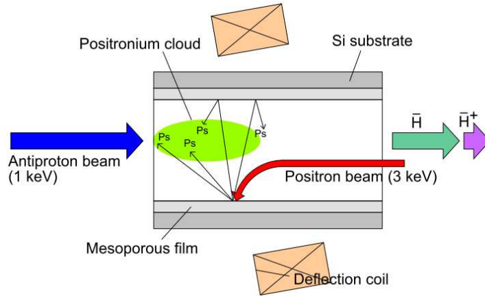
FIGURE 1.2 – Chambre de formation des ions \bar{\text{H}}^+ .
