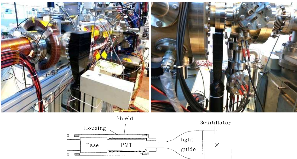
FIGURE 4.22 – En haut : Photo des détecteurs de positons. Assemblage de scintillateurs avec leur guide de lumière et leur photomultiplicateur. Les détecteurs sont recouverts d'un film opaque à la lumière visible. En bas : Schéma du montage.
