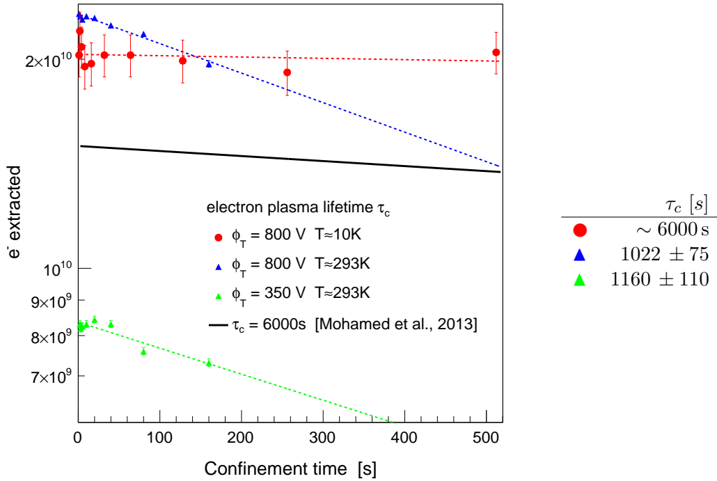
FIGURE 5.3 – Temps de confinement du plasma d'électrons. Les points rouges représentent le temps de vie du plasma dans la configuration 1 : la chambre à vide est refroidie à \sim 11 K, les charges sont détectées par éjection sur l'écran phosphore. Des mesures réalisées sur le remodérateur sont représentées par des triangles, avec la chambre à vide à température ambiante, pour des puits de potentiel de 800 V et 350 V. L'incertitude sur la mesure au niveau de l'écran phosphore est bien plus importante que sur le remodérateur, car il se trouve dans le champ de fuite du piège. Un ajustement avec une fonction exponentielle décroissante (eq. 5.2) est montrée par une ligne en pointillée pour chaque jeu de points de mesure. Le temps de vie obtenu au RIKEN est représenté pour comparaison par la ligne pleine noire [Mohamed et al. 2013].
