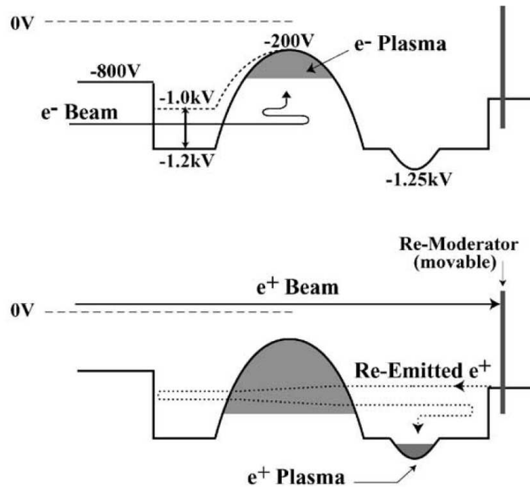
FIGURE 3.2 – Principe d'accumulation de la méthode développée par N. Oshima et ses collaborateurs. En haut, l'étape d'accumulation des électrons. En bas, l'étape d'accumulation des positons. Extrait de [Oshima et al. 2003]
