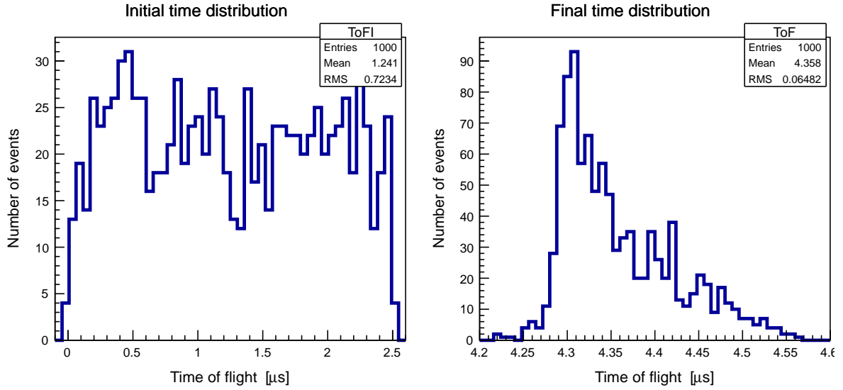
FIGURE 3.7 – Distribution simulée d'un pulse de positons comprimé temporellement au point focal. La distribution en temps initiale est présentée à gauche, la distribution au plan focal à droite. La largeur à mi-hauteur de la distribution finale est de 153 ns. \sim 59\% des positons sont compris dans une fenêtre de 80 ns. La distribution angulaire initiale est isotrope et la dispersion en énergie est de 0.7 eV (voir la figure 3.9).
