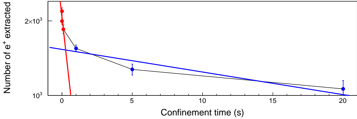
FIGURE 5.21 – Temps de vie des positons après 10 s d’accumulation. Les points correspondent au nombre de charges extraites du piège pour différents temps de confinement, jusqu’à 20 s. La diminution de charges détectée semble dominée par deux processus, un rapide (en rouge) et un lent (en bleu). L’ajustement des points par une fonction exponentielle décroissante donne des constantes de temps respectives de 860 ms et 47 s.
