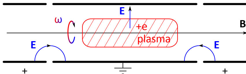
FIGURE 2.1 – Schéma de principe d'un piège de Penning-Malmberg.
