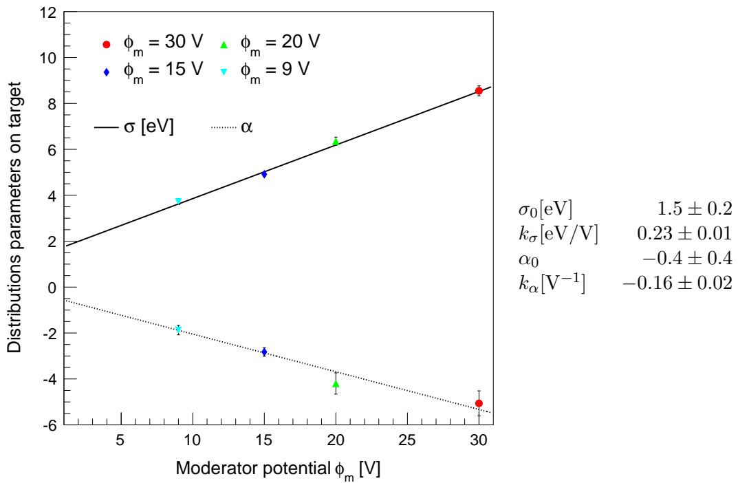
FIGURE 5.8 – Valeurs de \sigma et \alpha obtenues avec l'ajustement de l'équation (5.6) au niveau du détecteur, en fonction du potentiel \phi_m sur le modérateur. Les lignes montrent un ajustement linéaire des fonctions (5.7) et (5.8) dont les valeurs des paramètres sont présentées à droite de la figure.
