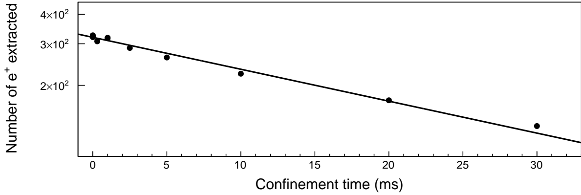
FIGURE 5.17 – Temps de vie des e^+ sans processus de refroidissement. Chaque point représente le nombre de positons détectés en fonction du temps de confinement dans le piège. Les barres d'erreurs sont confondues avec les points. Le délai \Delta t d'ouverture de gate2 est étendu jusqu'à 30 ms. La baisse du flux de positons traduit leur temps de vie dans le piège. La ligne noire correspond à un ajustement des points par une fonction exponentielle décroissante. La constante de temps donnée par l'ajustement est de 32 \pm 4 ms.
