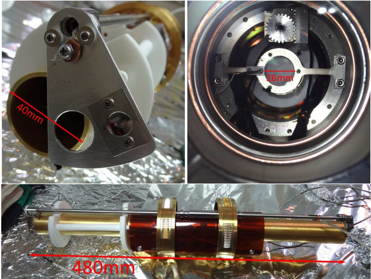
FIGURE 4.21 – Photos du remoderateur et de sa structure mécanique amovible. En haut à gauche, le porte remoderateur. Le remoderateur est vissé sur la structure. A sa gauche, l'orifice permettant le passage des positons. En haut à droite, la roue dentée qui transforme le mouvement du moteur pas à pas en mouvement de rotation de la tige du remoderateur. Sous la roue on peut voir l'écran phosphore. En bas, le bloc d'extraction des électrodes avec la tige de rotation du remoderateur.
