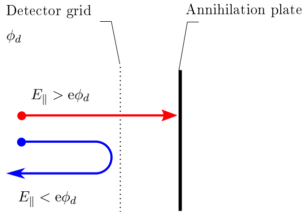
FIGURE 5.5 – Principe de la mesure de la distribution en énergie du faisceau. En augmentant le potentiel \phi_d , on limite le flux sur la cible d'annihilation aux positons ayant une énergie E_{\parallel} > e\phi_d .
