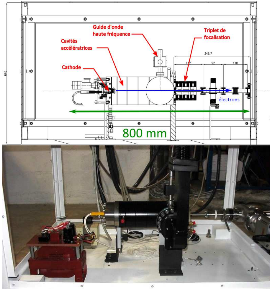
FIGURE 4.3 – Accélérateur linéaire d'électrons. Les dimensions sont données en mm.
