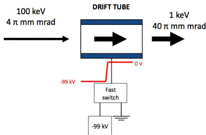
FIGURE 1.1 – Schéma de principe du décélérateur d'antiprotons de GBAR. Il permet d'adapter l'énergie du faisceau délivré par ELENA (100 keV) à la valeur optimale pour la formation d'ions \bar{\text{H}}^+ ( \sim 6 \text{ keV} ).
