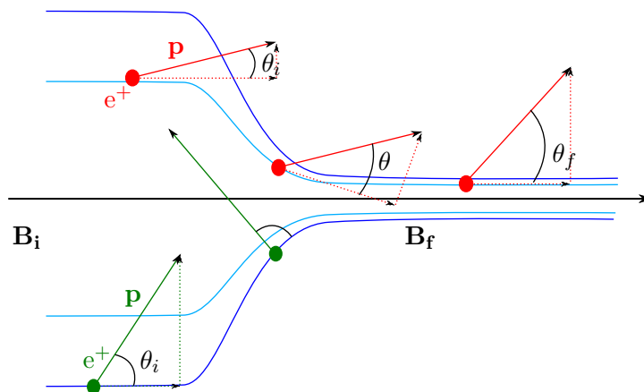
FIGURE 3.11 – Illustration du principe du miroir magnétique. La rotation cyclotron des positons autour des lignes de champ magnétique n’est pas représentée pour plus de visibilité. Dans le cas du positon représenté en rouge, le rapport initial entre impulsion longitudinale et impulsion transverse est assez important pour que le positon franchisse le gradient de champ. Quant au positon représenté en vert, toute son impulsion longitudinale est transférée sur la composante transverse. Le positon n’a d’autre choix que de rebrousser chemin.
