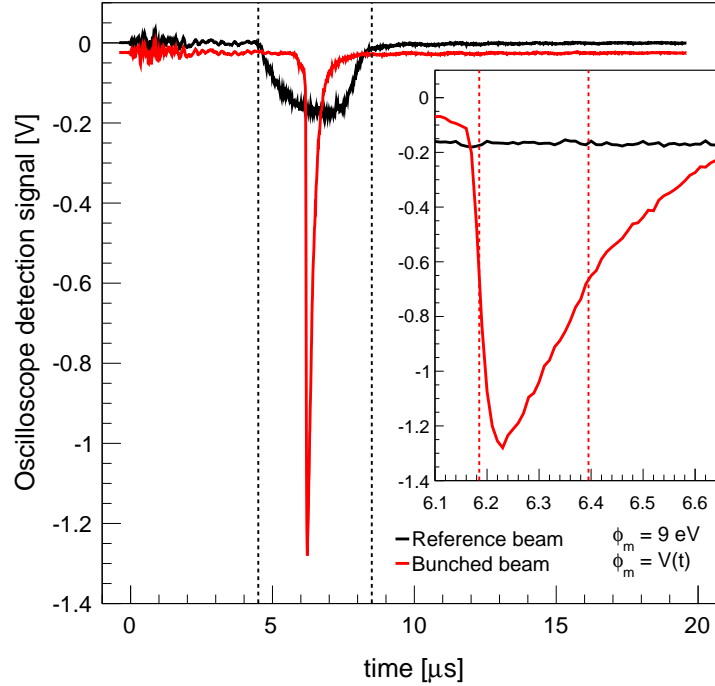
FIGURE 5.10 – Compression temporelle du faisceau de positons sur la cible amont du piège. La courbe noire correspond au signal obtenu en appliquant un potentiel statique de 9 V sur le modérateur (faisceau de référence). La courbe rouge montre le signal obtenu en appliquant le potentiel dynamique sur le modérateur (test 09 dans le tableau 5.4). Un agrandissement sur le pic du faisceau comprimé montre sa largeur à mi-hauteur, de 220 ns. Le résultat de la simulation présentée à la figure 3.7 page 37 montre une largeur de la distribution en temps sur le détecteur de 153 ns. L'élargissement de la distribution en temps peut s'expliquer par l'élargissement de la distribution en énergie pendant le transport.
