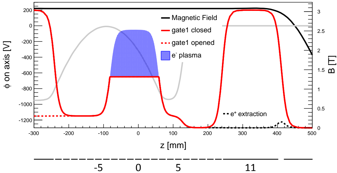
FIGURE 5.18 – Profil de potentiel sur l’axe lors de l’accumulation des positons, appelée configuration 3 . Le champ magnétique est de 3 T. Cette configuration est dégradée pour le confinement des électrons. La configuration 1 , utilisé précédemment pour confiner les électrons, est rappelée en gris clair (le champ magnétique est alors de 5 T).
