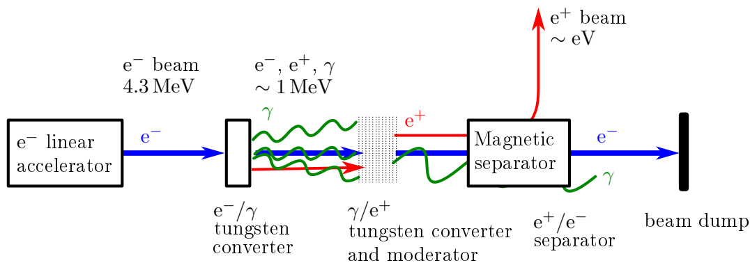
FIGURE 4.7 – Schéma simplifié du processus principal de production de positons lents par modulation avec une multicouche de grilles de tungstène.
