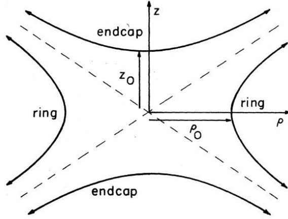
FIGURE 2.2 – Piège de Penning idéal avec deux électrodes hyperboliques (endcap) et une électrode annulaire cylindrique (ring). Le potentiel vaut V(z, \rho) = V_0 \frac{z^2 - \rho^2/2}{2d^2} où V_0 est la différence de potentiel appliquée sur les électrodes et d^2 = \frac{1}{2} (z_0^2 + \rho_0^2/2) [Brown and Gabrielse 1986].
