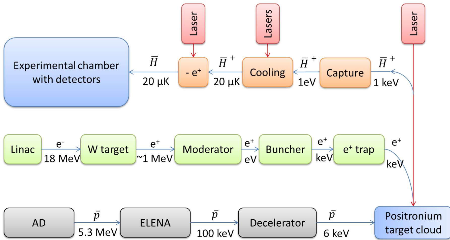
FIGURE 1.6 – Schéma synoptique de l'expérience GBAR.
