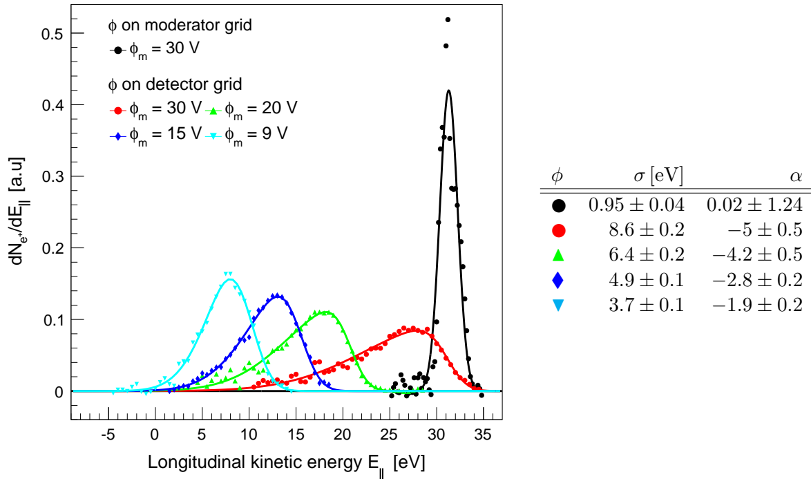
FIGURE 5.7 – Distribution énergétique du faisceau. Les données expérimentales sont représentées par les points, les lignes correspondent à un ajustement avec la fonction (5.6). Les distributions sont centrées sur \phi_m pour plus de visibilité, en fixant \mu = \phi_m pour chaque mesure. On observe une augmentation de la largeur et de l'asymétrie des distributions avec le potentiel initial sur le modérateur. Les paramètres de l'ajustement sont donnés dans le tableau à droite de la figure.
