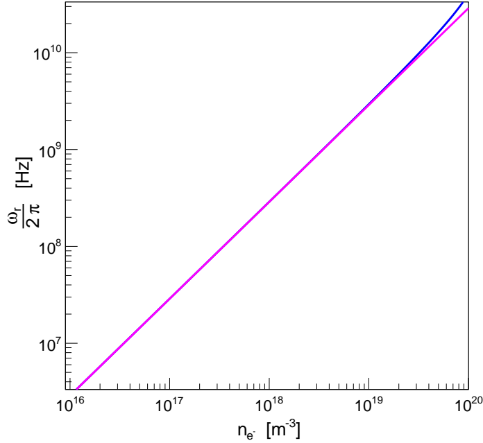
FIGURE 2.5 – Fréquence de rotation \frac{\omega_r}{2\pi} du plasma en fonction de sa densité n sur 4 ordres de grandeurs. La courbe bleue correspond à la solution \omega_- , la courbe rose à la solution approchée \omega_E .
