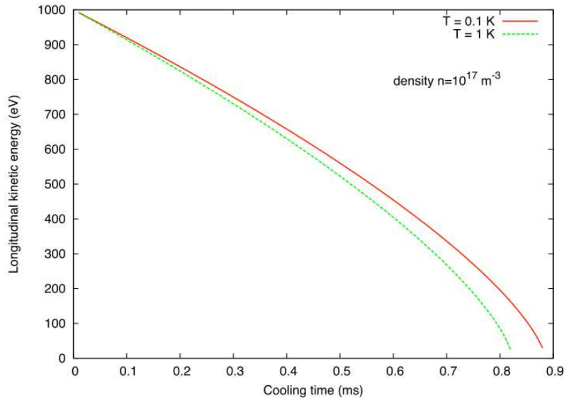
FIGURE 3.4 – Simulation du refroidissement de positons dans un plasma d'électrons de densité n = 10^{17} \text{ m}^{-3} réalisé par P. Dupré. L'énergie longitudinale des positons est tracée en fonction du temps passé dans le plasma d'électrons. Les résultats sont présentés pour un plasma d'électrons avec une température de 1 K et 0.1 K. Extrait de [Dupré 2011].
