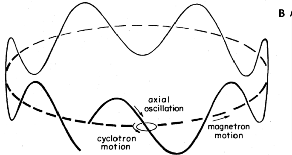
FIGURE 2.3 – Mouvement d'une particule chargée dans un piège de Penning. La ligne pointillée représente le cercle du mouvement magnétron. La ligne pleine couple ce mouvement avec l'oscillation longitudinale. Le mouvement complet prend en compte la rotation cyclotron autour de la ligne pleine [Brown and Gabrielse 1986].
