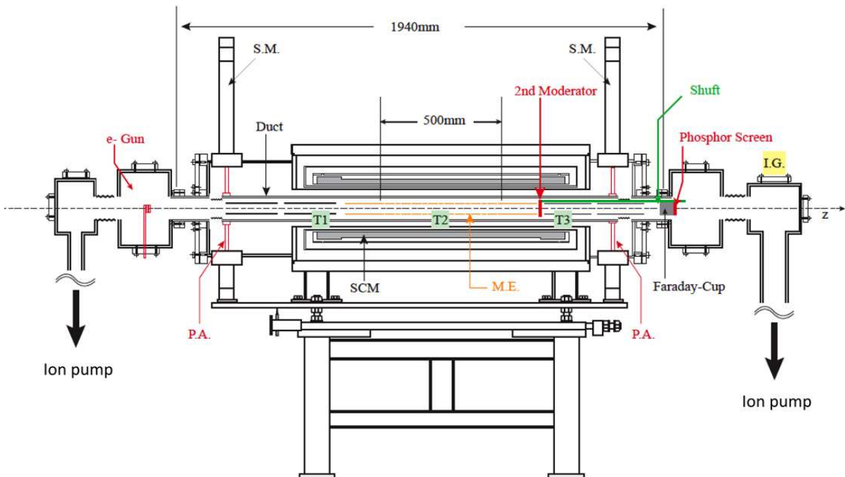
FIGURE 4.13 – Piège du RIKEN. L'axe faisceau correspond à l'axe des z croissant. La bobine supraconductrice est représentée en gris (SCM). Les moteurs pas à pas permettant de bouger le tube faisceau dans le champ magnétique sont désignés par le sigle SM. T1, T2 et T3 montrent l'emplacement des 3 sondes de température de la chambre à vide. Les électrodes sont représentées en orange (ME) et le mécanisme du remoderateur ( 2^{\text{nd}} moderator) est schématisée en vert (shuft). Chaque pompe ionique est équipée d'une jauge de pression (IG). Le canon à électrons est situé côté injection. L'écran phosphore, qui sert à la fois d'écran luminescent, de faraday cup et de cible d'annihilation, est placé dans la zone d'extraction. Le remoderateur et sa mécanique ont aujourd'hui été retiré du piège. Une représentation de l'ensemble des électrodes à l'échelle est présentée à la figure 4.24.
