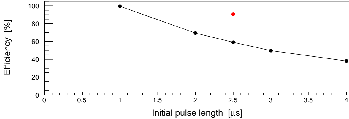
FIGURE 3.9 – Efficacité de compression en fonction de la durée initiale du pulse. La distribution angulaire initiale est isotrope et l'écart type de la distribution en énergie vaut \sigma = 0.7 \text{ eV} . Chaque point correspond à un résultat de simulation, la ligne est un guide pour les yeux. Les points représentés en noir respectent la condition V_{\text{max}} = 150 \text{ V} . Le point rouge ne respecte pas cette condition. Il correspond à une vitesse de rampe maximum atteinte de 2 \text{ kV}/\mu\text{s} .
