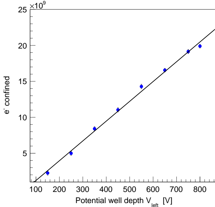
FIGURE 5.2 – Nombre d'électrons confinés en fonction de la profondeur du puits de potentiel. Chaque point correspond au nombre de charges piégées dans une configuration donnée (voir tableau 5.3). La durée d'injection est de 2s, le temps de confinement est de 3s.
