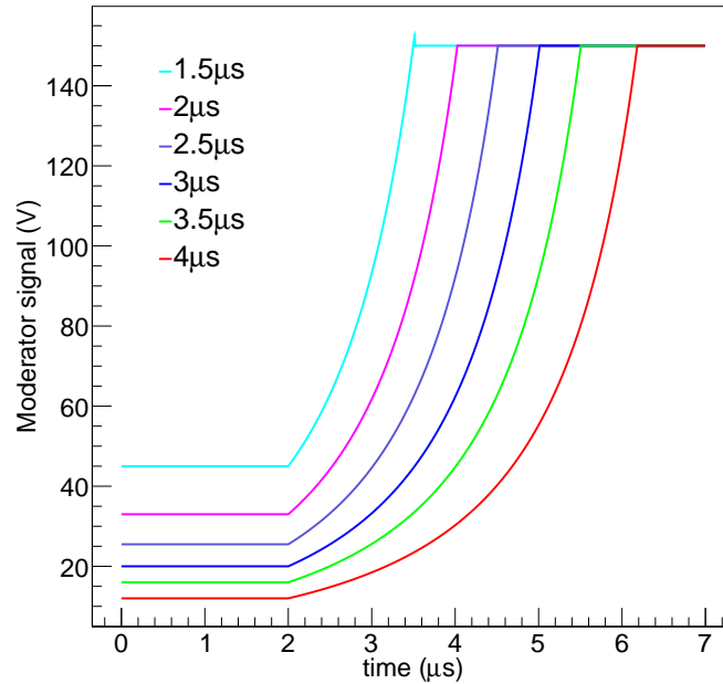
FIGURE 4.11 – Courbes générées par le générateur de fonction arbitraire avec différents \Delta t [\mu s] = \Delta n \times 5000 \mu s . Un plateau de potentiel est appliqué pendant 2 \mu s pour s’assurer que le potentiel initial est bien défini sur le modérateur au moment de la génération du faisceau. Un délai permet de mettre en phase f(n) avec le déclenchement du linac.
