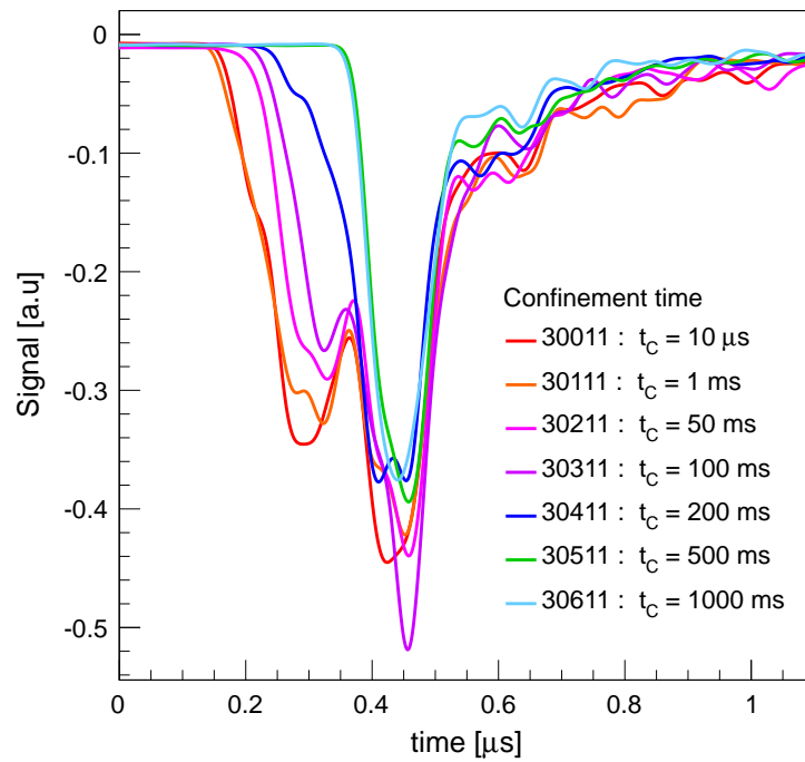
FIGURE 5.22 – Temps de vol des positons éjectés après différents temps de confinement. Les traces sont lissées pour améliorer la visibilité. Le temps d'accumulation est de 3 s.
