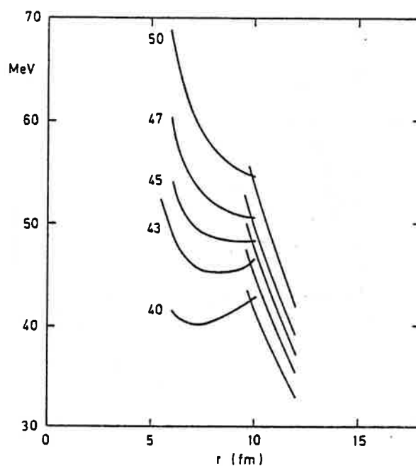
Fig. VI.15. Barrières de fission du noyau ^{52}\text{Cr} pour différentes valeurs du moment angulaire l . Le moment angulaire maximum l_{Bf} est à peu près égal à 45 (d'après Broglia et al, BD 80).
