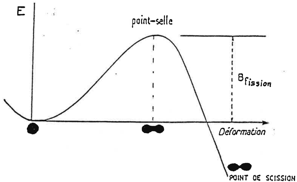
Fig. VI.3. Energie de déformation de la goutte liquide pure (ca 95)
