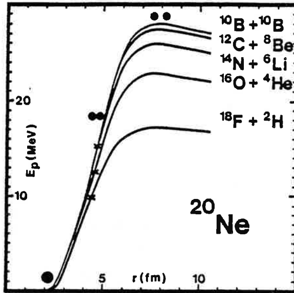
Fig. V.1. Barrières de potentiel pour la fragmentation du noyau ^{20}\text{Ne} dans les cinq voies de sortie suivantes : ^{10}\text{B} + ^{10}\text{B} , ^{12}\text{C} + ^8\text{Be} , ^{14}\text{N} + ^6\text{Li} , ^{16}\text{O} + ^4\text{He} et ^{18}\text{F} + ^2\text{H} . Le paramètre \beta = R_2/R_1 prend respectivement les valeurs 1.00, 0.87, 0.75, 0.63 et 0.48. Le point de contact est indiqué par une croix.
