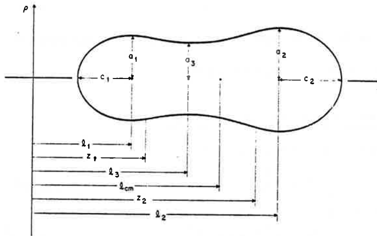
Fig. III.5. Chaque surface est spécifiée par la position l_i de son centre, son demi-axe transverse a_i et sa demi-élongation c_i . Les nappes se joignent en z_1 et z_2 . l_{c.m.} donne la position du centre de masse.
