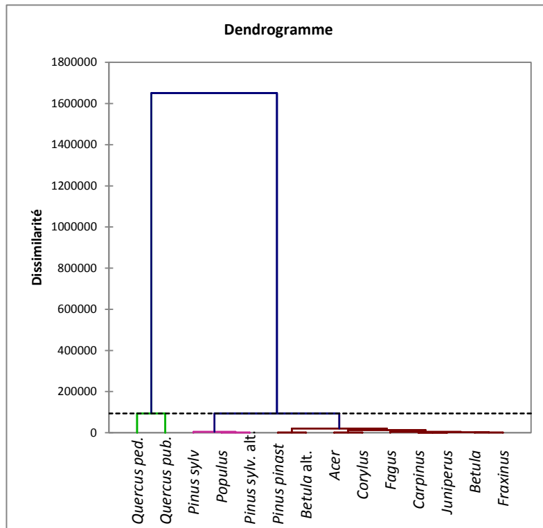
Figure 128 : Dendrogramme issu de la classification ascendante hiérarchique des taxons (toutes espèces, classe de taille de fragments et lots inclus)
