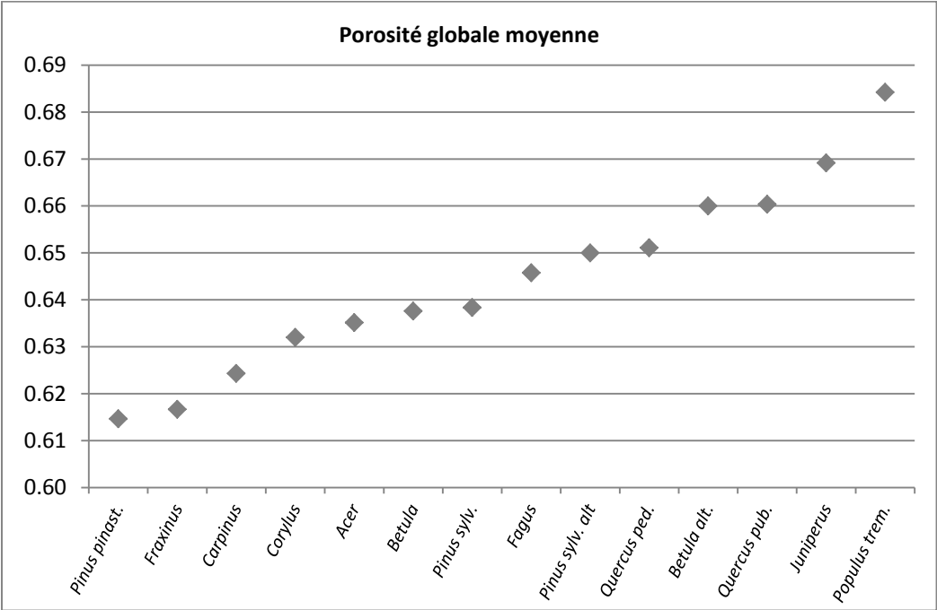
Figure 3 : Indice de porosité globale moyenne des taxons (bois initial et bois final confondus : l'indice mesure les zones de vides à l'échelle globale de l'échantillon)
