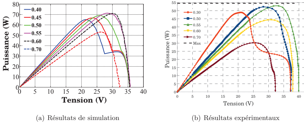
Figure 19: Effet du rapport cyclique dans la courbe P-V
