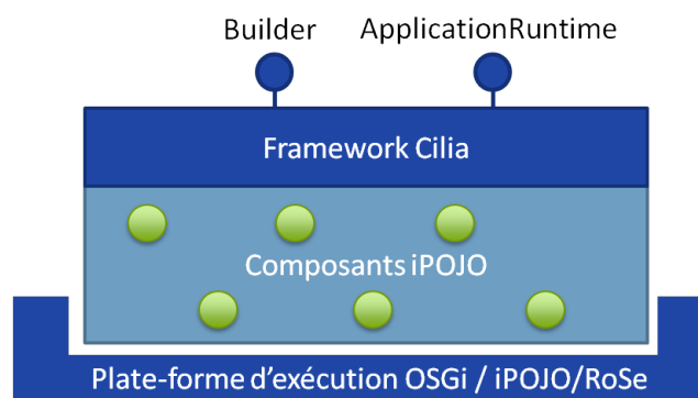
FIGURE 6.5 – L'interface CiliaContext .
