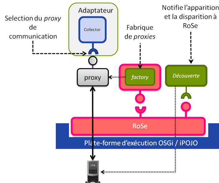
FIGURE 6.4 – Adaptateur avec le framework RoSe.
