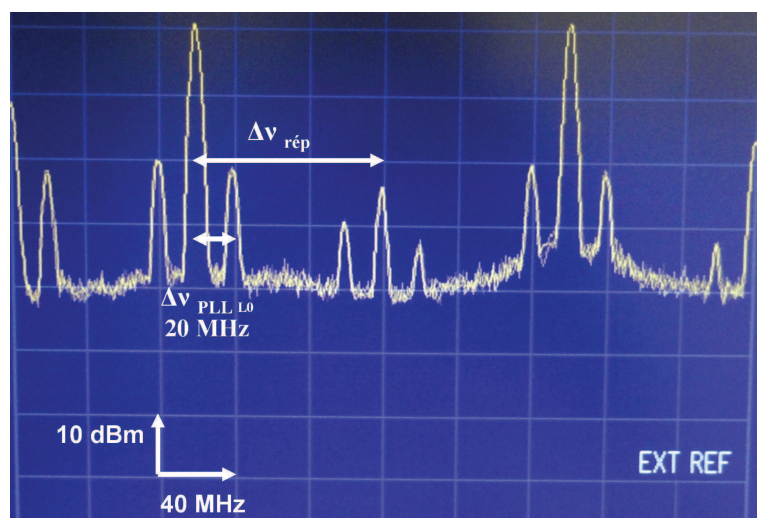
FIGURE 1.11: Photographie de l'écran de l'analyseur de spectre du signal reçu par une photodiode éclairée par le peigne de fréquence et la diode laser L0.
