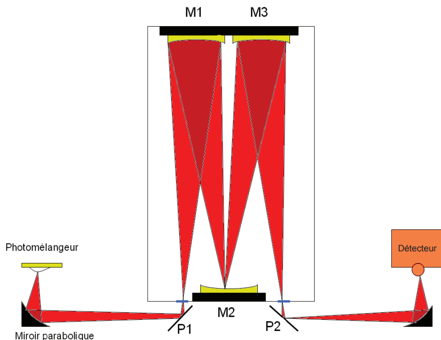
FIGURE 1.12: Schéma d'une cellule multipassage de type White utilisée en expérience de photomélange
