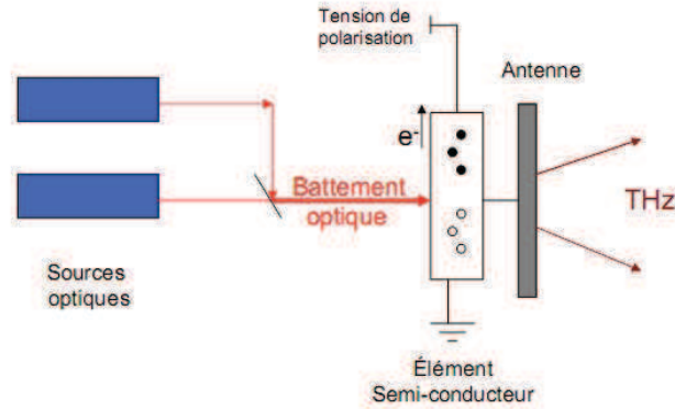
FIGURE 1.4: Schéma de principe de la génération d'ondes THz par technique de photomélange
