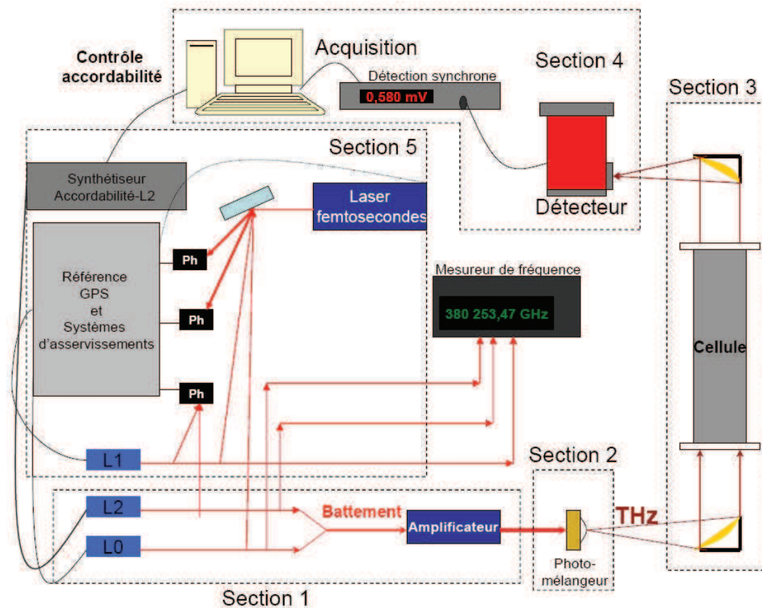
FIGURE 1.3: Représentation schématique du banc de spectroscopie THz à onde continue par photomélangement. Ph est ici l'abréviation utilisée pour photodiode, L1, L2 et L0 sont respectivement les trois diodes laser à cavité étendue utilisées pour cette expérience. Section 1 : sources optiques, Section 2 : Photomélangeur, Section 3 : Environnement échantillon, Section 4 : Détection et acquisition, Section 5 : Métrologie de fréquence
