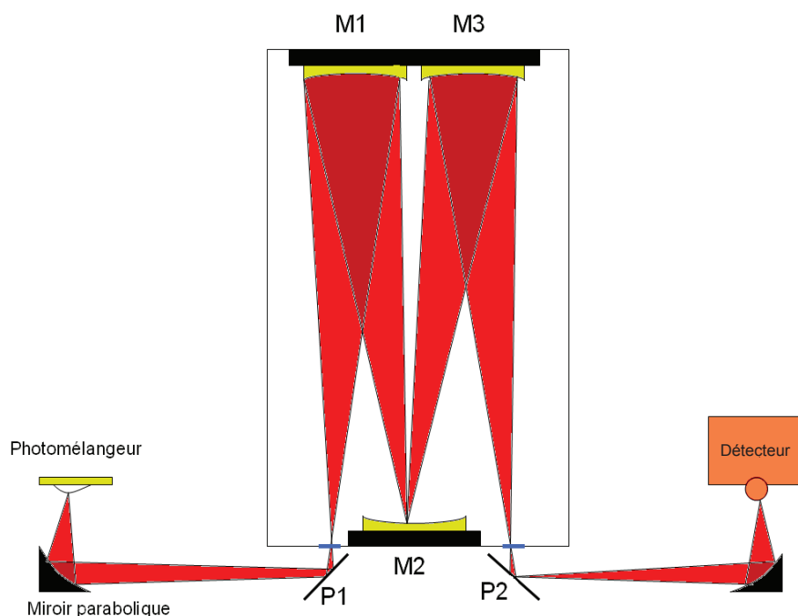
FIGURE 1.12: Schéma d'une cellule multipassage de type White utilisée en expérience de photomélangage
