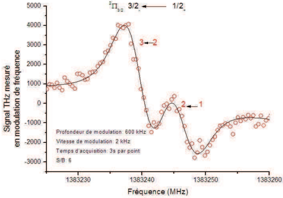
FIGURE 4.8: Structure hyperfine du radical SH partiellement résolue à 1,3 THz, enregistrée sur le banc THz par photomélange du LPCA par détection de la première harmonique du signal modulée en fréquence. Résolution 400 kHz. Les points expérimentaux sont en ronds rouge, l'ajustement est en ligne noire obtenu grâce au programme FitHarmo développé par L. Croizé [18] .
