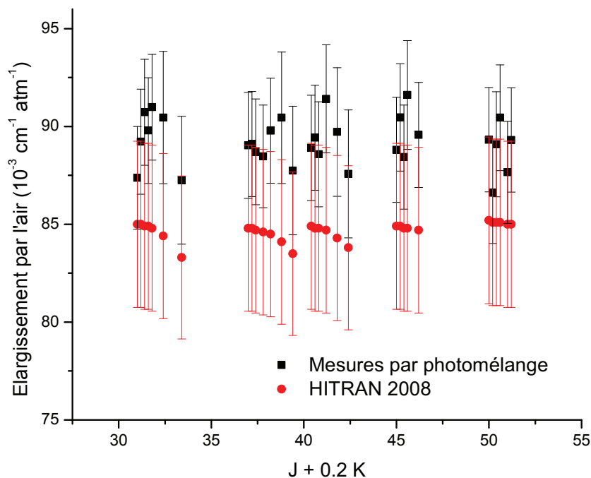
FIGURE 2.8: Dépendance en J du coefficient d'élargissement par l'air pour les hautes valeurs de J . Comparaison des données obtenues par technique de photomélange avec les valeurs estimées par HITRAN 2008.
