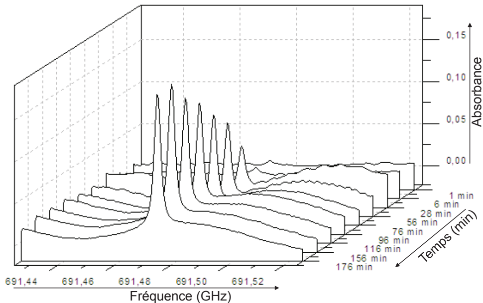
FIGURE 5.6: Enregistrement de la raie complète de CO en fonction du temps, pour des conditions de photolyse du formaldéhyde avec filtre AM 0. Résolution 500 kHz, 300 ms par point.
