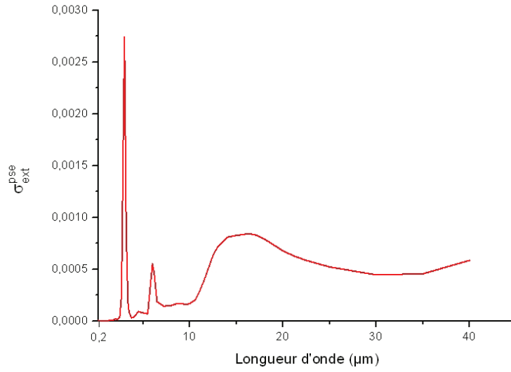
FIGURE 5.19: Section efficace d'extinction de particules solubles dans l'eau pour des aérosols sphériques de 70 nm de diamètre et une concentration estimée à 3 \cdot 10^6 particules/ \text{cm}^3 .
