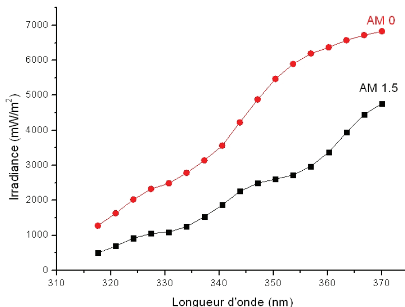
FIGURE 5.5: Spectres, entre 317 et 370 nm, du simulateur solaire obtenus par un spectroradiomètre placé à 12 cm de la source de lumière. En ronds rouges, en présence du filtre AM 0 seulement. En carrés noirs, en présence du filtre AM 1.5.
