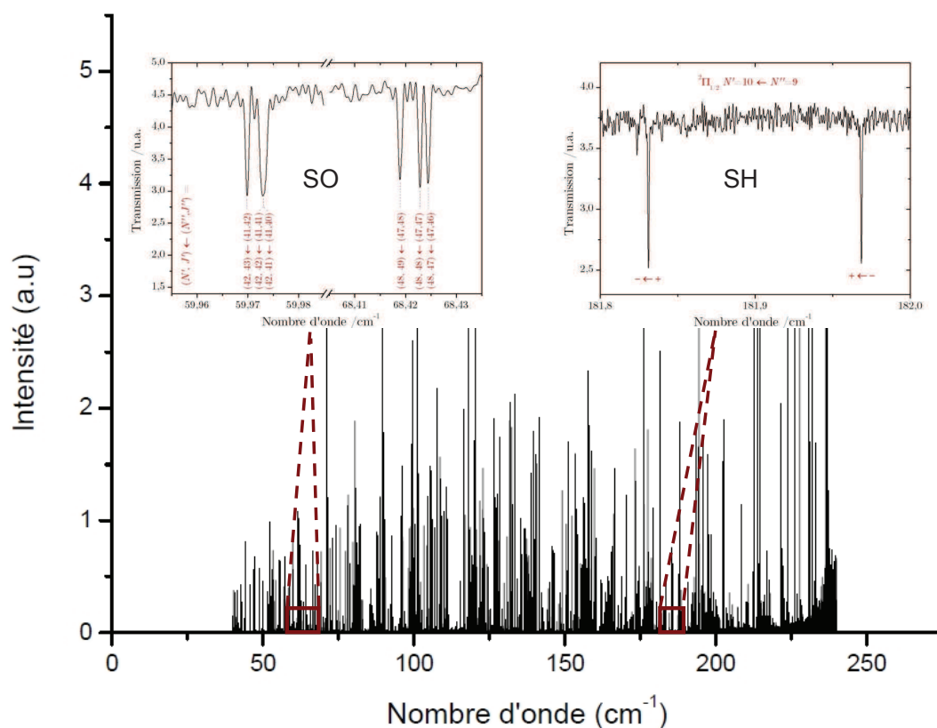
FIGURE 4.11: Spectre obtenu sur la ligne AILES par décharge DC (980 W) dans un flux d'un mélange H 2 S, He, H 2 , air. En encart, un agrandissement sur les transitions des radicaux SO et SH. Des raies du précurseur H 2 S et de l'eau sont également présentes sur le spectre. Résolution 0,00102 cm -1 (30 MHz), spectre résultant de l'accumulation de 98 spectres.
