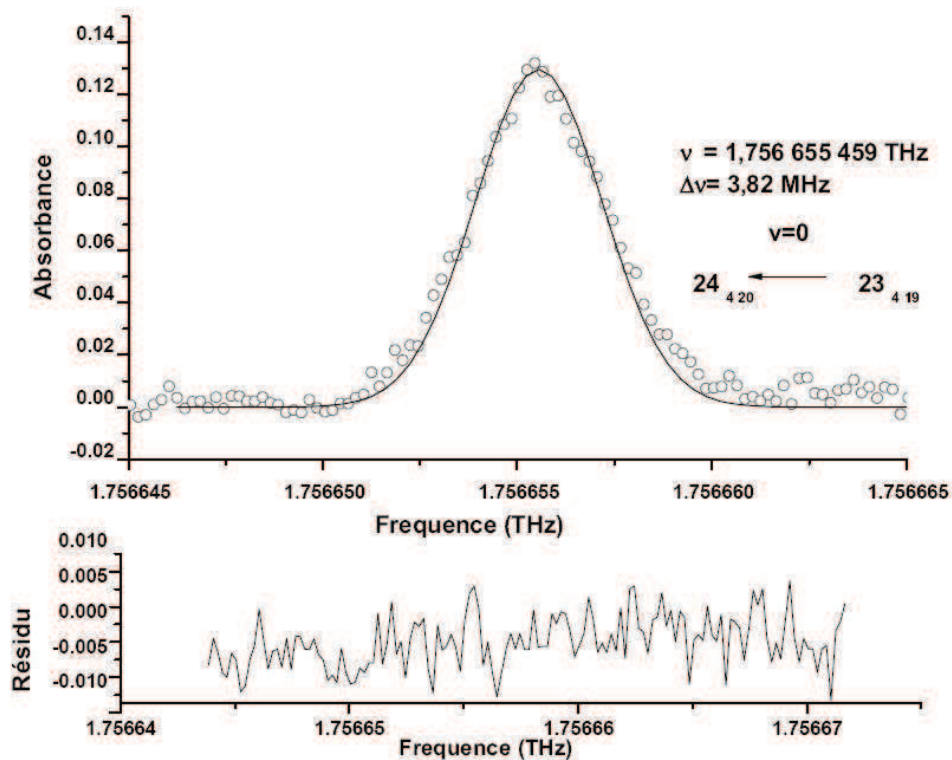
FIGURE 1.14: Transition de rotation pure dans l'état vibrationnel fondamental du formaldéhyde enregistrée sur le spectromètre à onde continue THz par photomé-lange à 1.7 THz à une pression de 80 \mu bar et dans une cellule de 60 cm de trajet optique. La courbe noire représente la modélisation de la transition, les ronds vides représentent les points expérimentaux.
