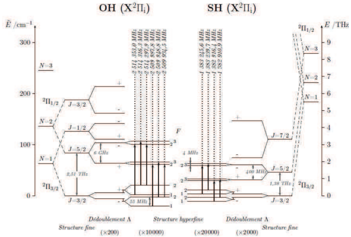
FIGURE 3.1: Diagramme des niveaux d'énergie des radicaux OH et SH [1]. Par souci de clarté, ce diagramme n'est pas à l'échelle.
