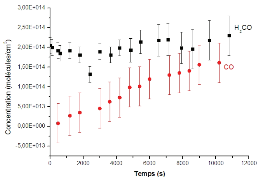
FIGURE 5.9: Concentrations de monoxyde de carbone et de formaldéhyde en fonction du temps, enregistrées lors de la même expérience avec utilisation du filtre AM 1.5.
