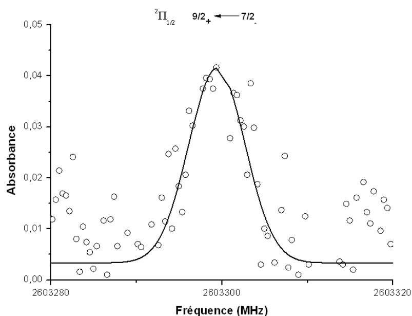
FIGURE 4.10: Composante de dédoublement- \Lambda du radical SH enregistrée à 2,6 THz sur le banc par photomélange du LPCA. Résolution 400 kHz. Ici les composantes hyperfines ne sont pas résolubles car séparées seulement de 200 kHz l'une de l'autre [39].
