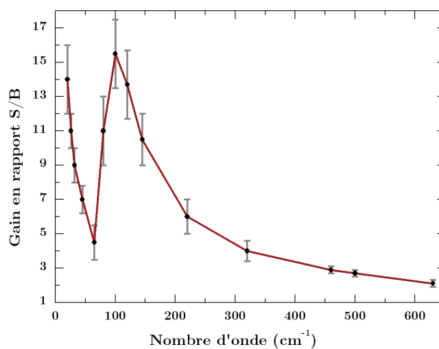
FIGURE 4.1: Rapport signal-sur-bruit obtenu avec rayonnement synchrotron divisé par celui obtenu en source interne (global), valeurs obtenues pour une résolution (maximale) de l'interféromètre (30 MHz-0.00102 cm -1 ). D'après [45]
