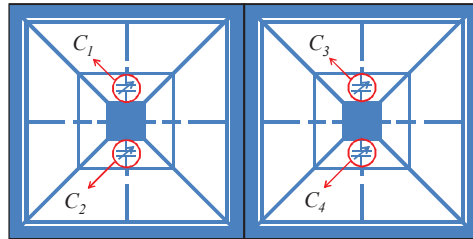
Fig. 5.21 : Deux cellules dans le guide d'onde, chargées par des capacités dissymétriques.
