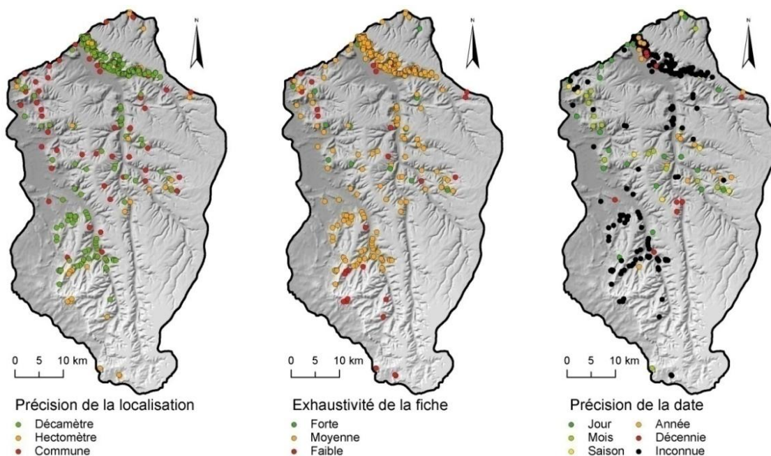
Figure 4.1 : Cartes de la distribution régionale de la catégorie "glissement" de la BDMvt, affichée selon des différents indicateurs de qualité disponibles pour la partie continentale du Pays d'Auge
