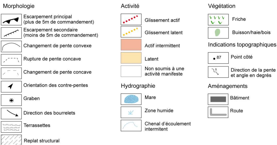
Figure 3.38 : Carte morphodynamique du secteur des Bottentuits (Saint-André-d’Hébertôt, Calvados)
