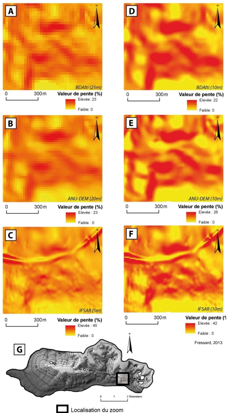
(A) MNT brut BDAlti, (B) MNT brut ANUDEM, (C) MNT brut IFSAR, (D) BDAlti rééchantillonnée à 10m, (E) ANUDEM rééchantillonné à 10m et (F) MNT IFSAR rééchantillonné à 10m, (G) localisation du zoom proposé
