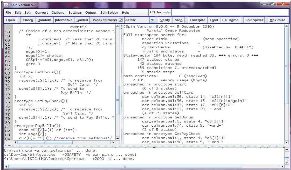
Figure 3.7 Vérification de la cohérence du processus de vente de voitures en jSpin
