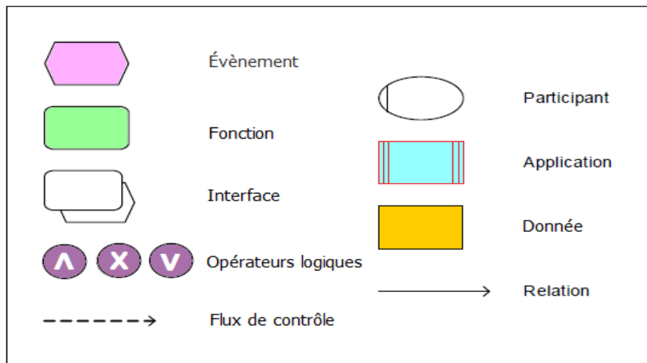
Figure 1.13 Éléments de base d'un diagramme EPC.
