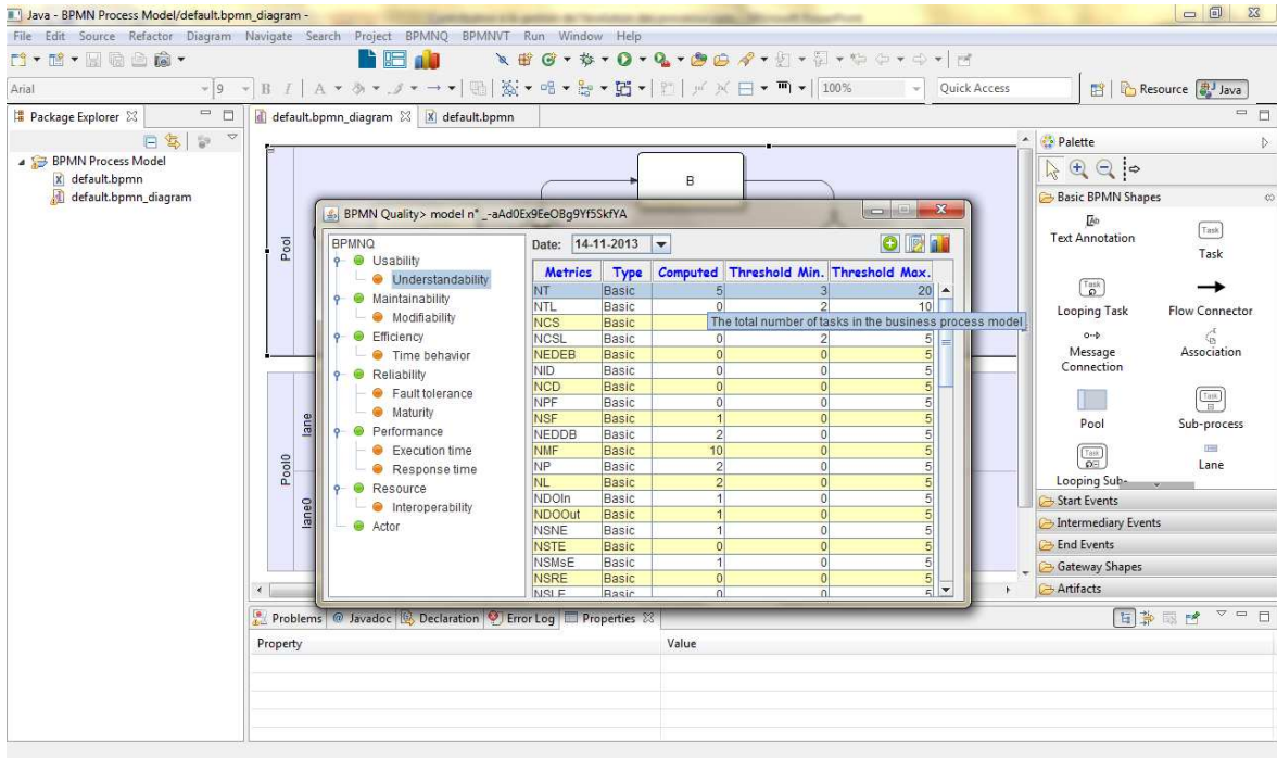
Figure 6.11 Évaluation des métriques d'un modèle BPMN par plug-in BPMNQ.
