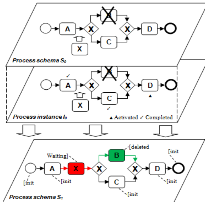
Figure 4.6 L'ajout de l'activité «X» et la suppression de l'activité «B»
