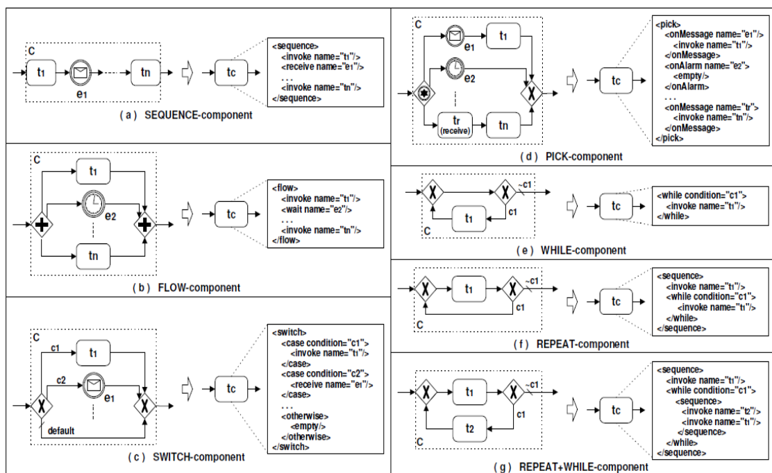
Figure 1.16 Transformation de BPMN à BPEL
