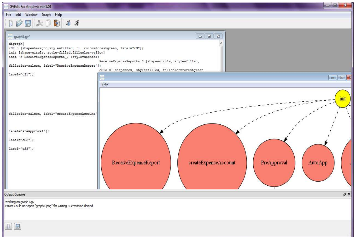
Figure 6.17 Visualisation du fichier Expense_reimbursement_process.dot avec Graphviz.
