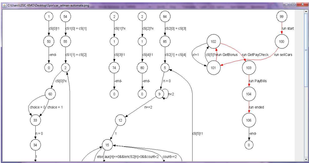
Figure 3.8 La structure de kripke générée par jSpin
