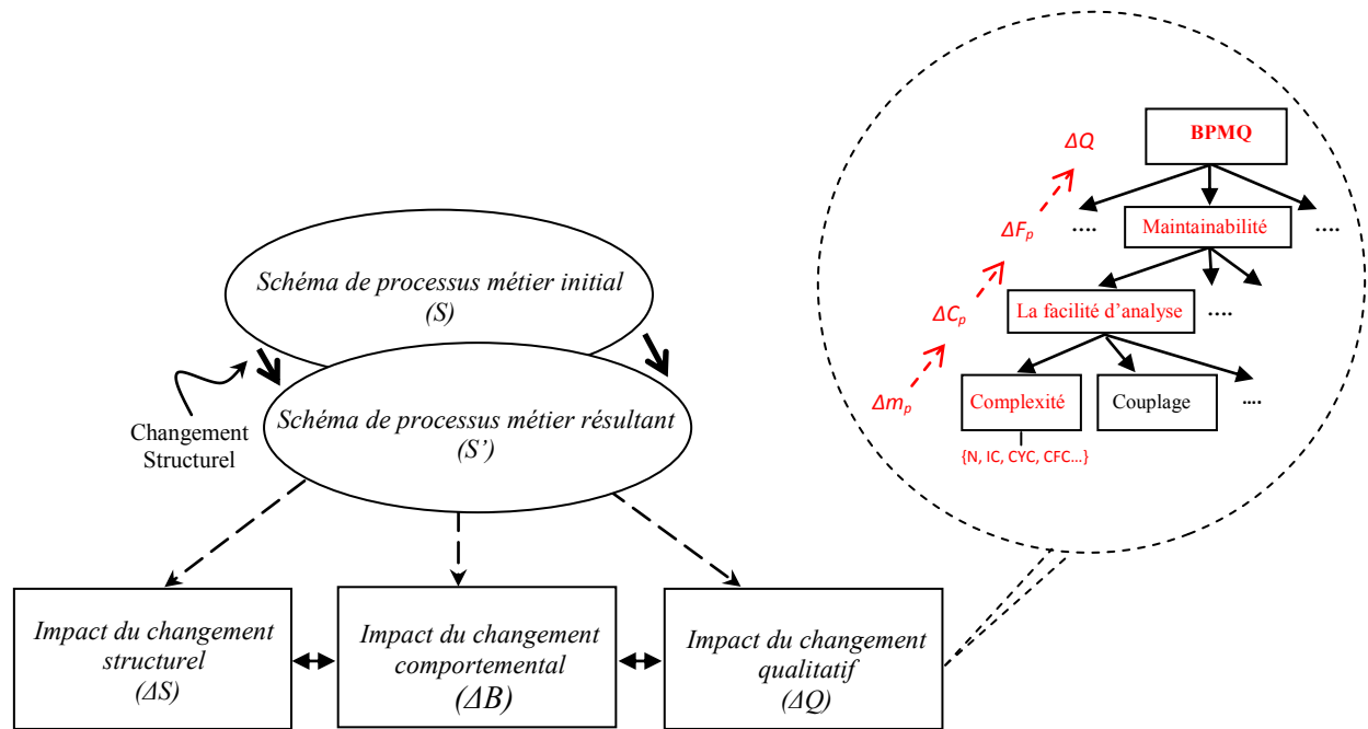
Figure 5.2 Relations entre l'impact structurel, comportemental et qualitatif du changement.
