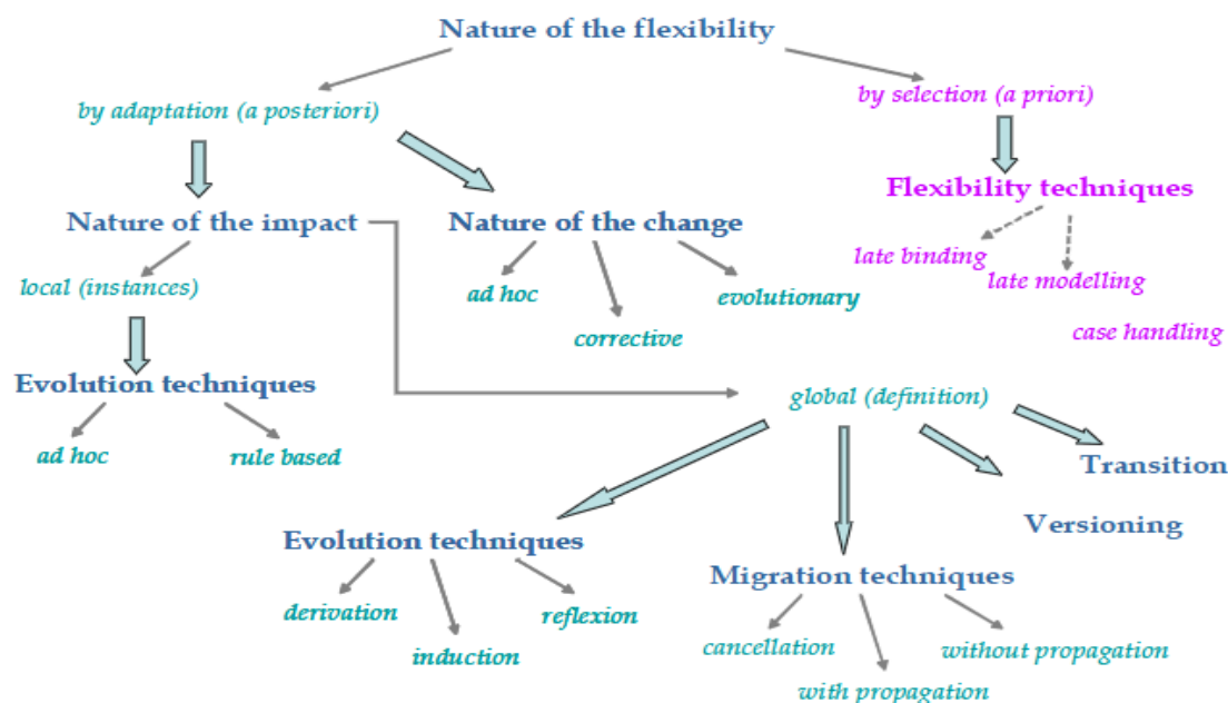
Figure 1.18 Les notions de changement selon la classification de Nurcan
