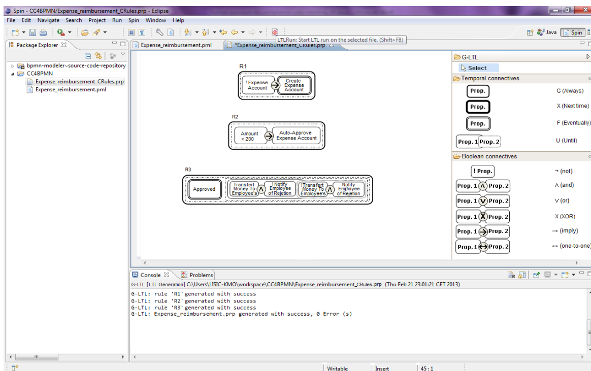
Figure 6.8 Le module CR2LTL.
