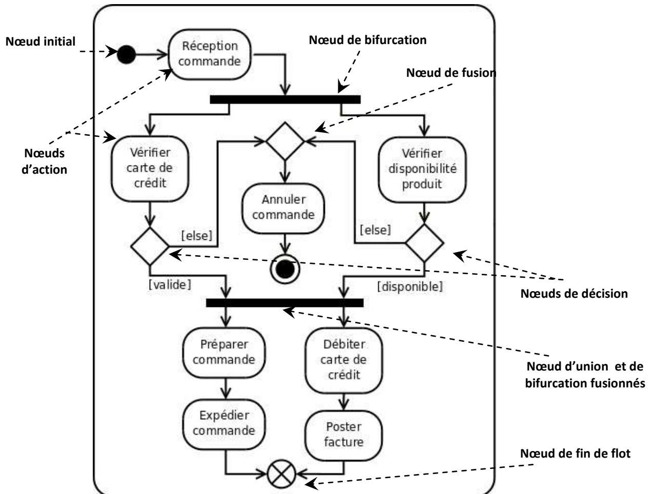
Figure 1.11 Processus de commande modélisé par le diagramme d'activités
