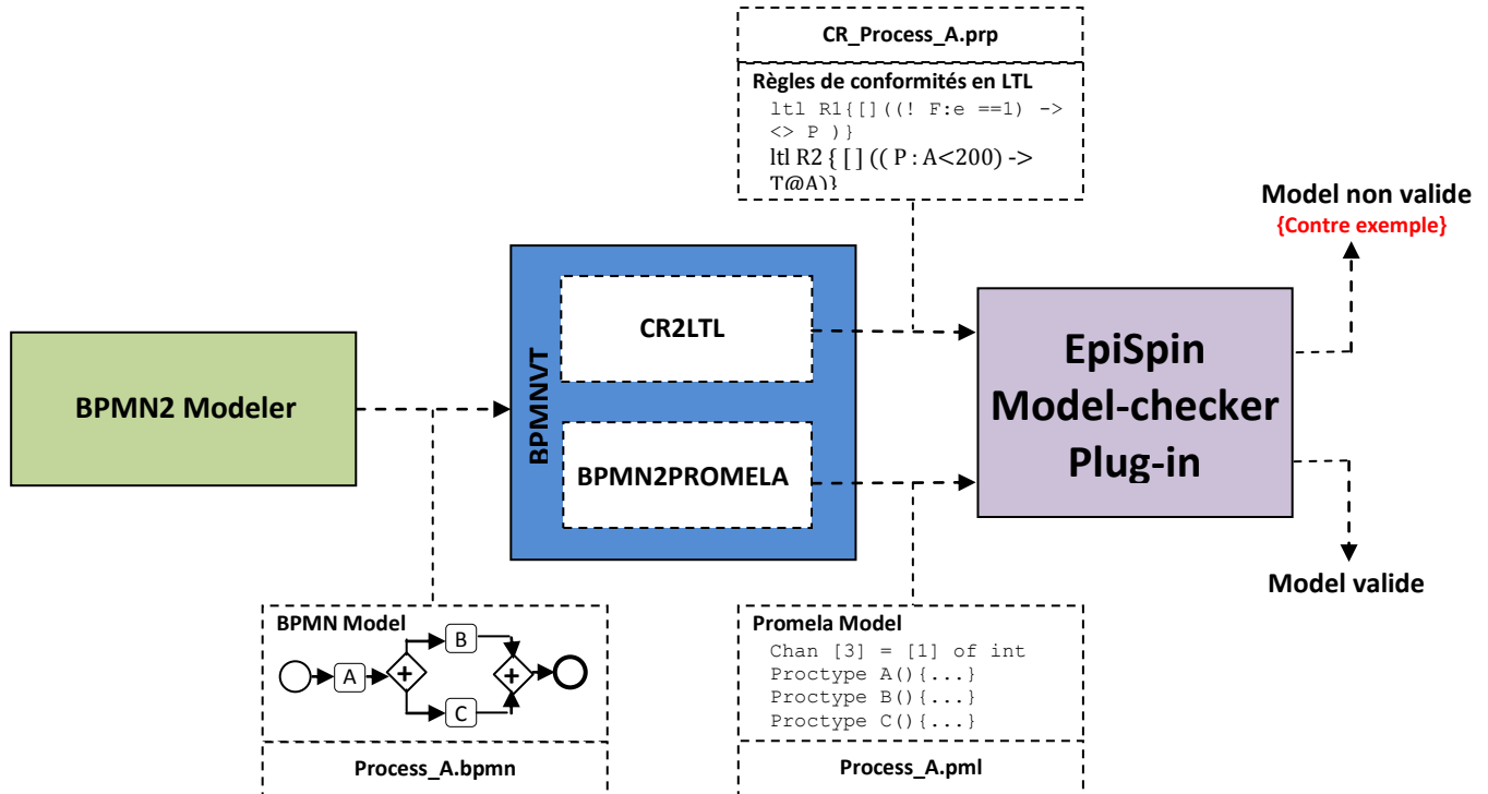
Figure 6.5 L'architecture du plug-in BPMNVT.
