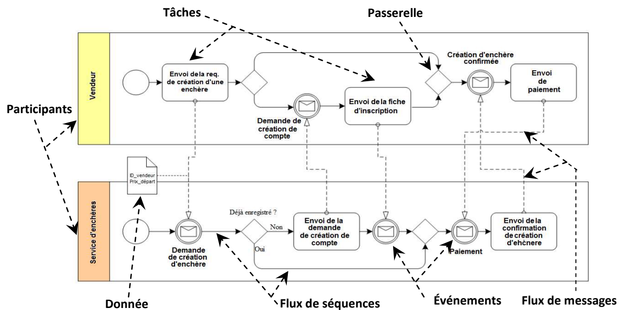
Figure 1.9 Processus de vente aux enchères modélisé par la notation BPMN
