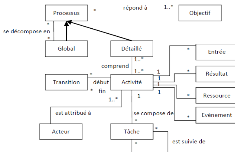
Figure 1.4 Méta modèle du processus métier selon (Morley, Hughes, Leblanc, & Hugues, 2007)
