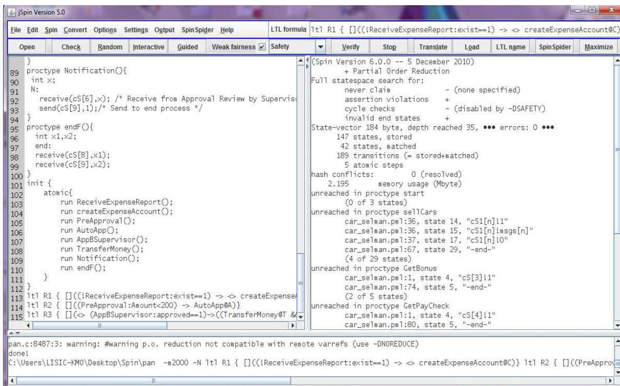
Figure 3.13 Résultats de la vérification de conformités du processus en jSpin
