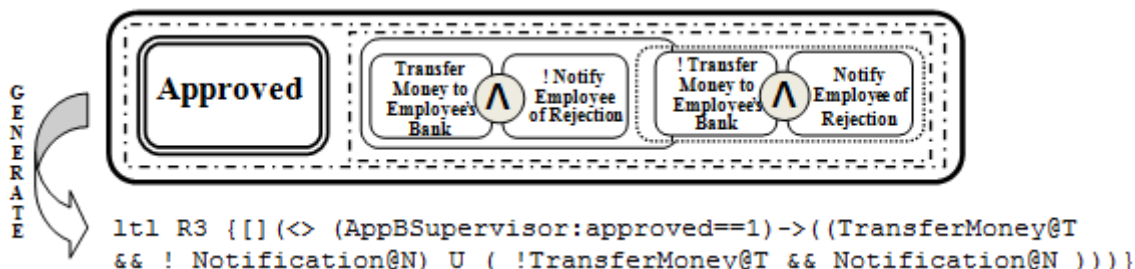
Figure 3.12 La représentation graphique de la règle «R3»
