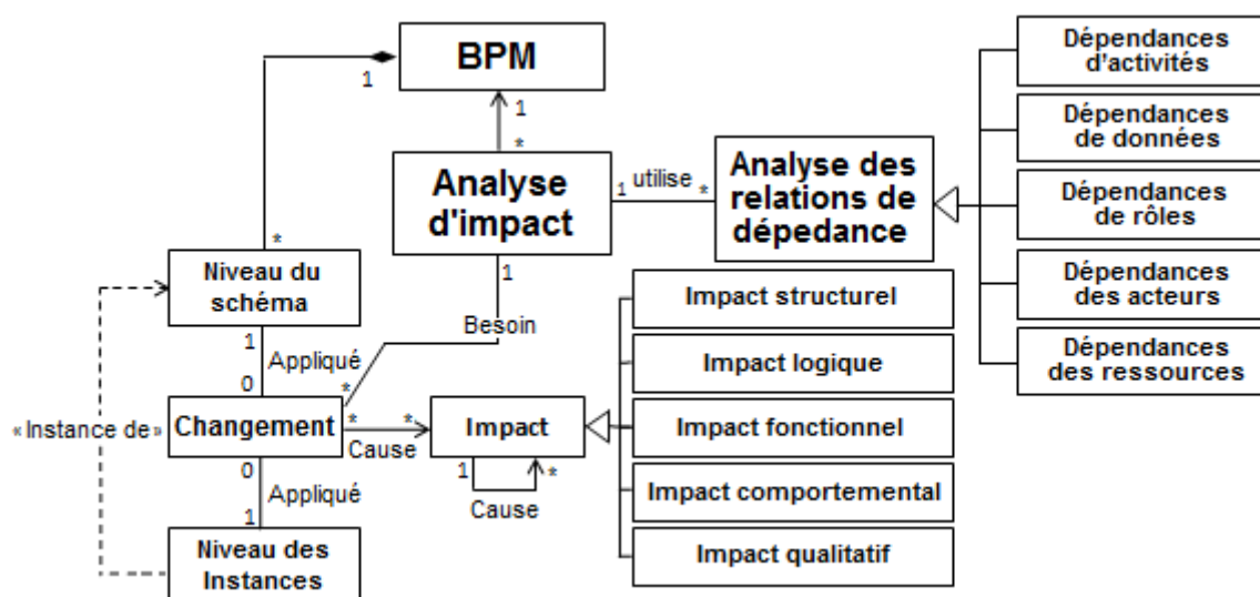
Figure 4.1 Analyse de l'impact du changement des processus métier
