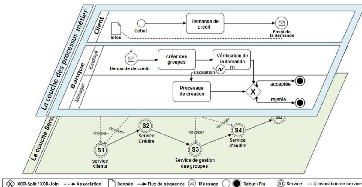
Figure 4.2 Dépendances multicouches dans les processus métier
