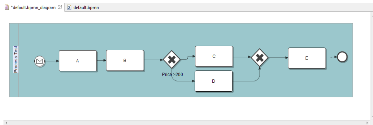
Figure 6.4 Extrait du fichier d'entrée « Description graphique ».
