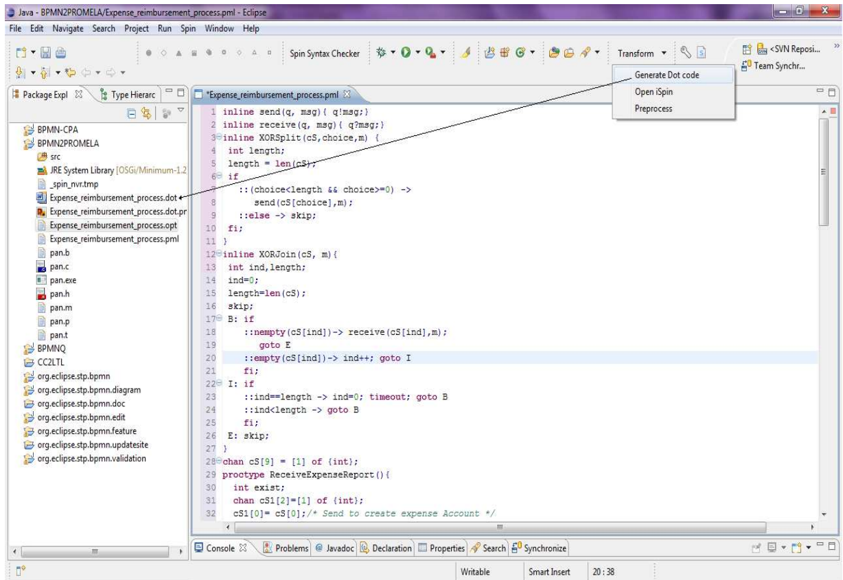
Figure 6.16 Génération du fichier Expense_reimbursement_process.dot .
