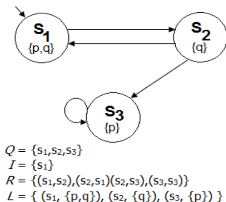
Figure 3.2 Un exemple de structure de kripke.
