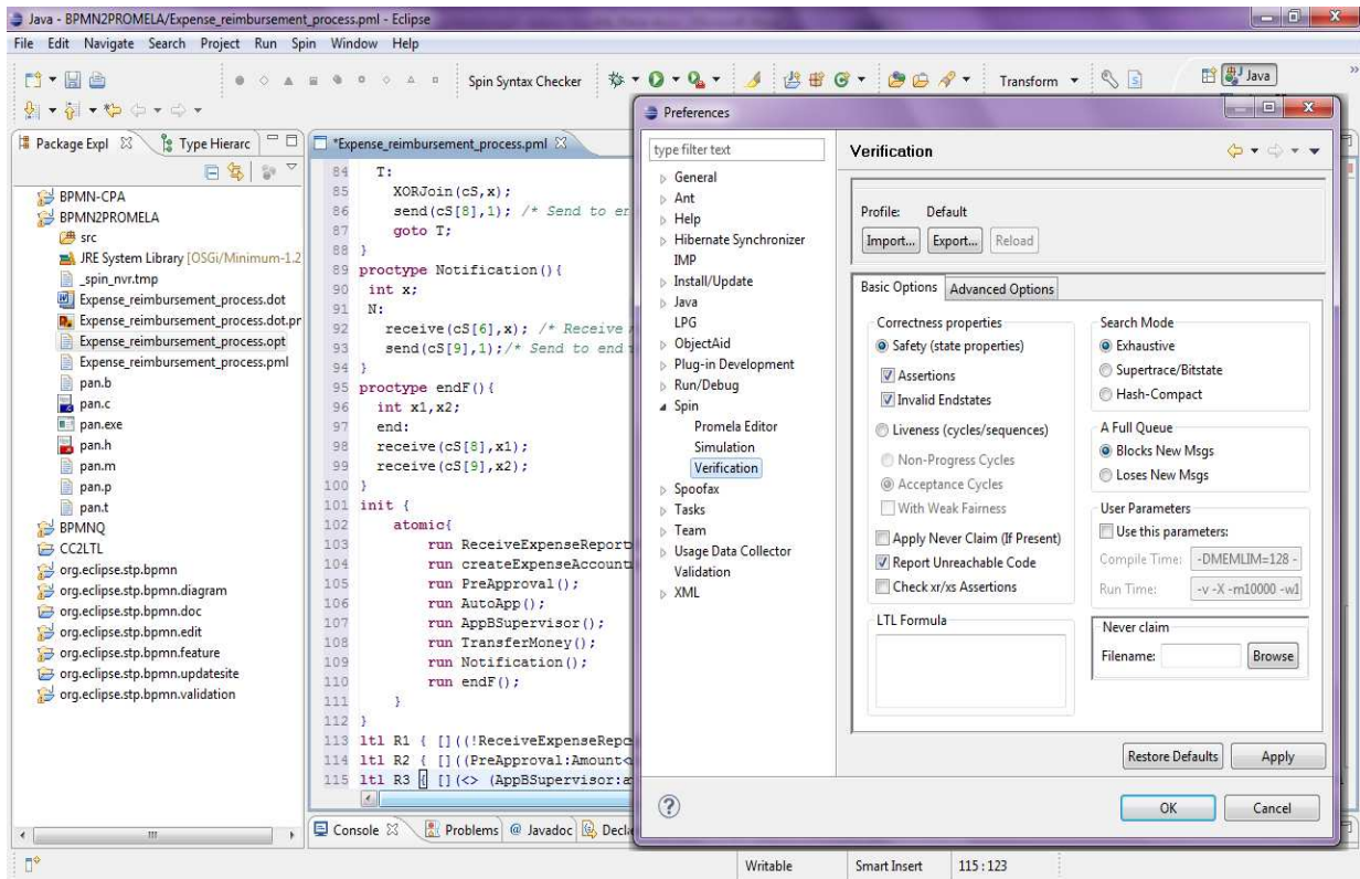
Figure 6.14 Modèle Promela généré par BPMN2PROMELA.
