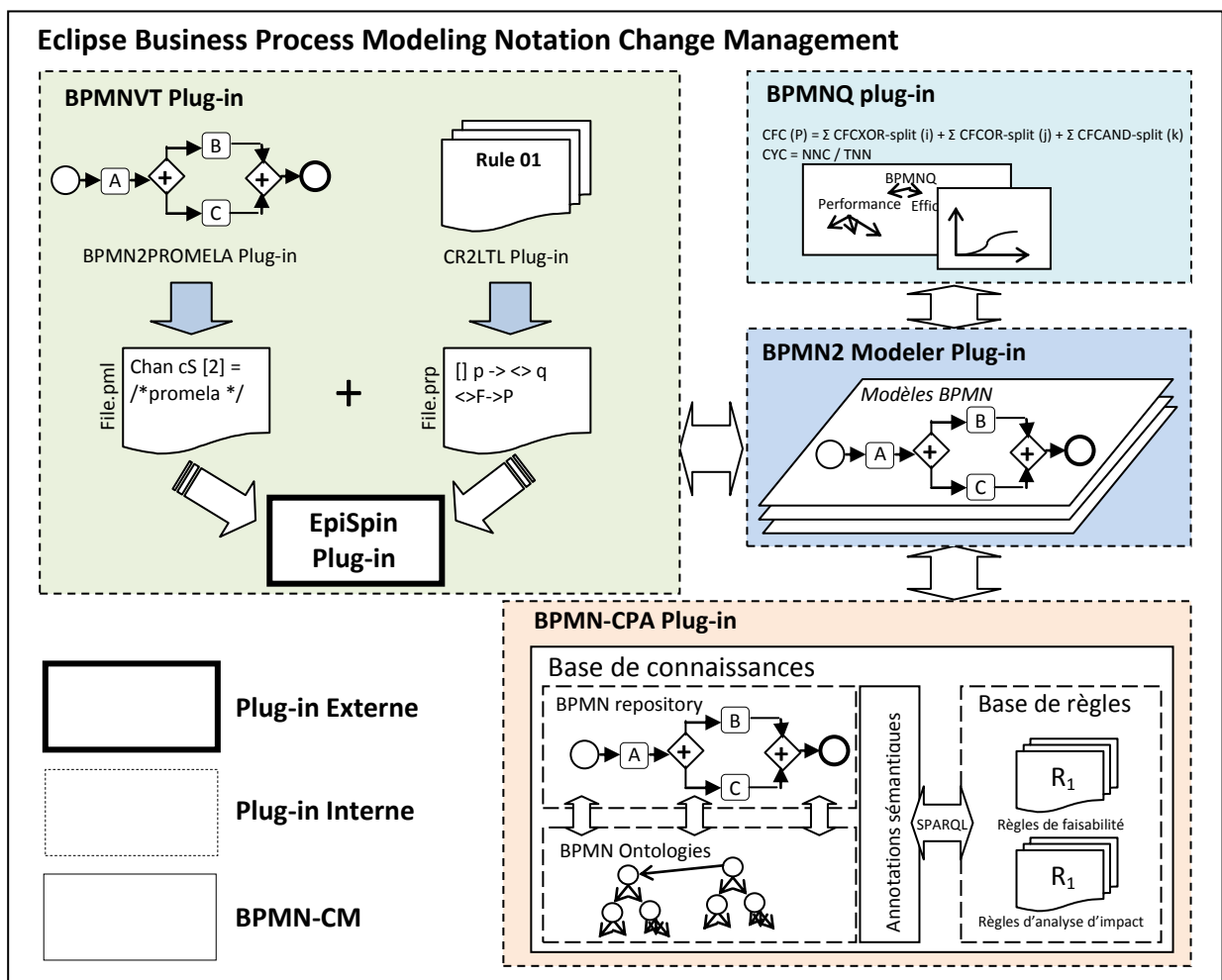
Figure 6.2 L'architecture générale de la plate-forme BPMN-CM.
