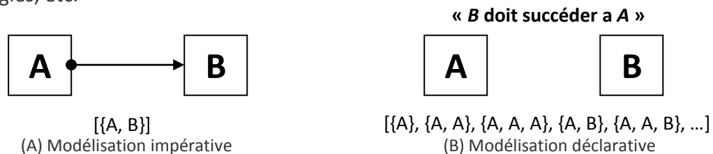
Figure 1.7 Modélisation impérative et modélisation déclarative
