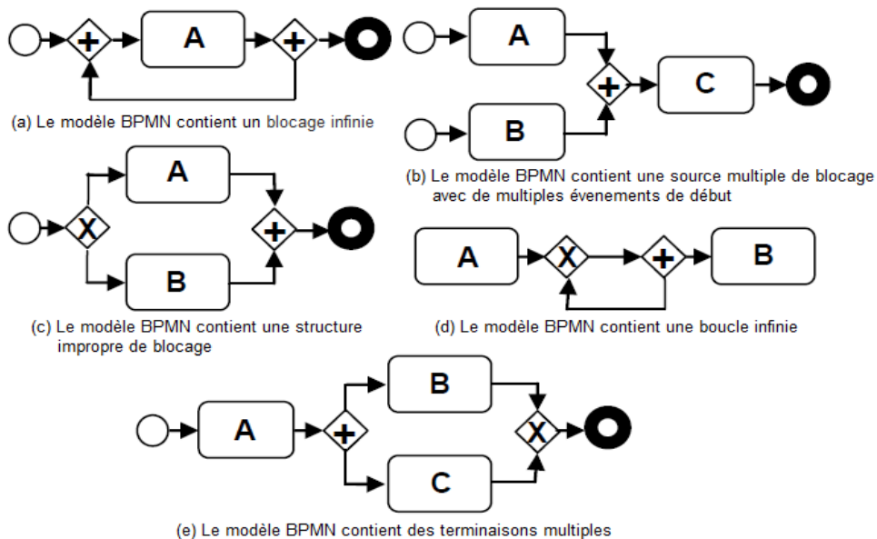
Figure 3.4 Les erreurs structurelles dans les modèles BPMN.
