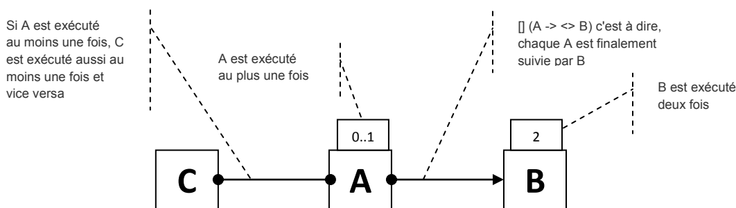
Figure 1.12 Un exemple simple d'un modèle CONDEC.
