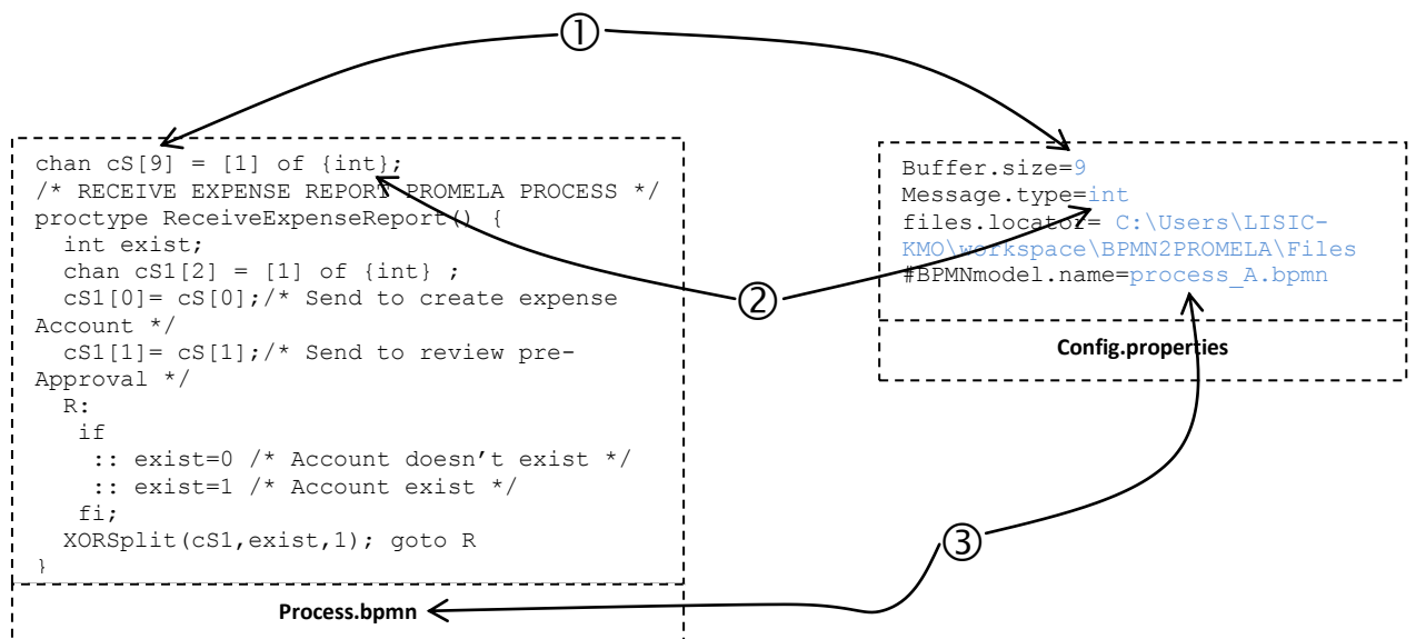
Figure 6.7 Fichier de configuration de BPMNVT.
