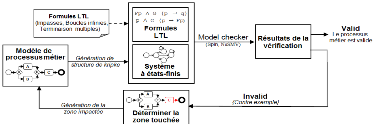
Figure 3.5 Vérification des modèles de processus métier basée sur le model-checking.
