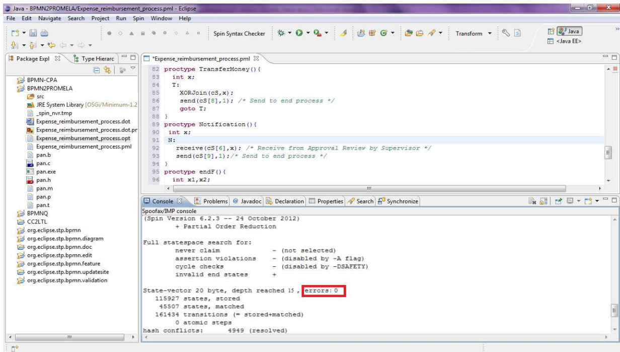
Figure 6.15 Vérification de la cohérence du processus de remboursement des frais par EpiSpin.
