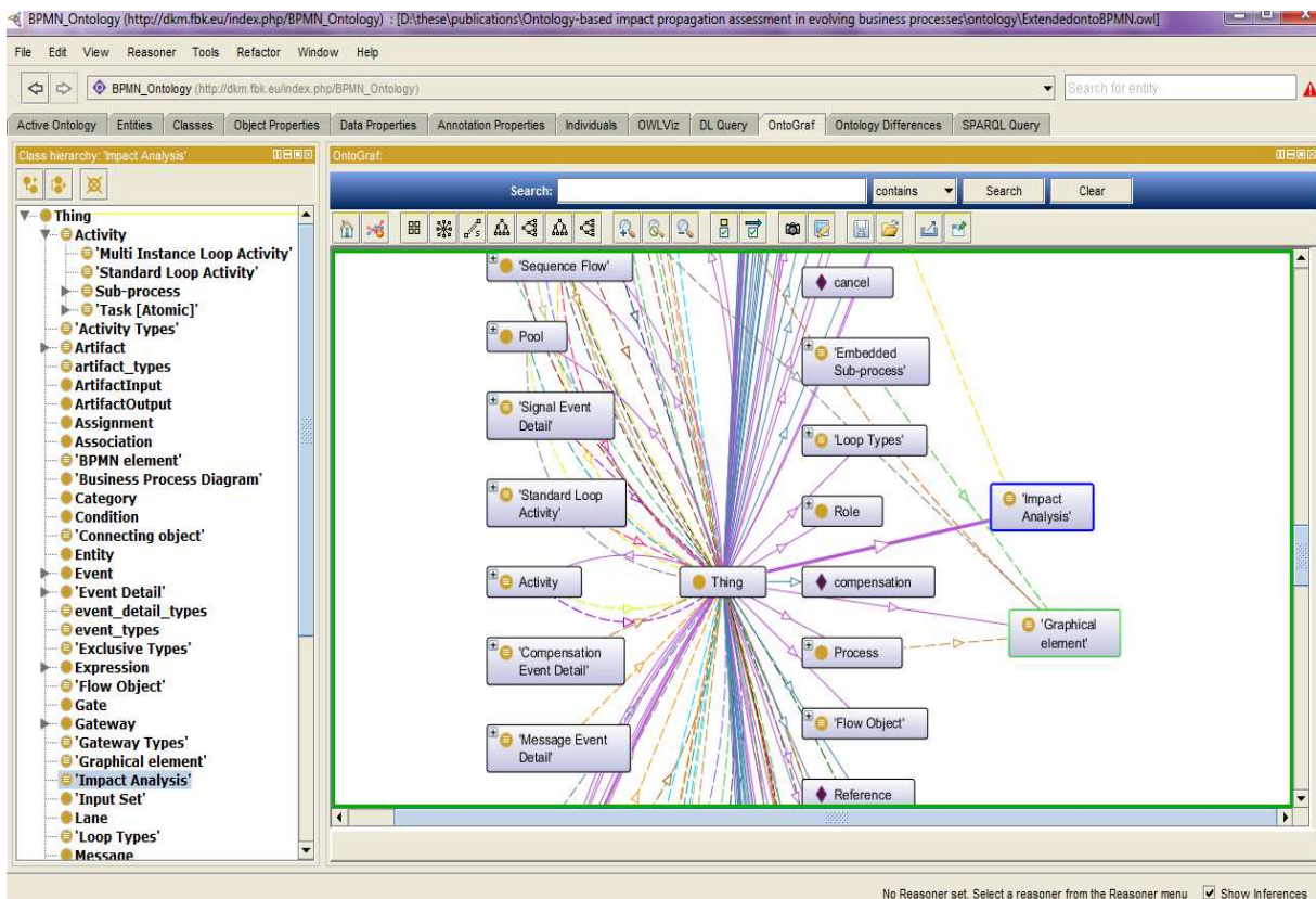
Figure 4.4 Hiérarchie des classes de extended BPMN 2 Ontology
