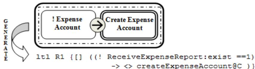
Figure 3.10 La représentation graphique de la règle «R1»
