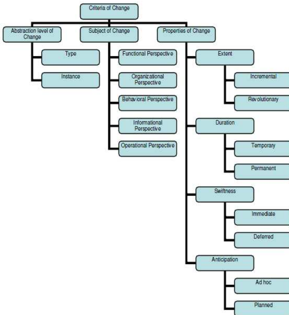
Figure 1. 17 Les notions de changement selon la classification de Regev et al.
