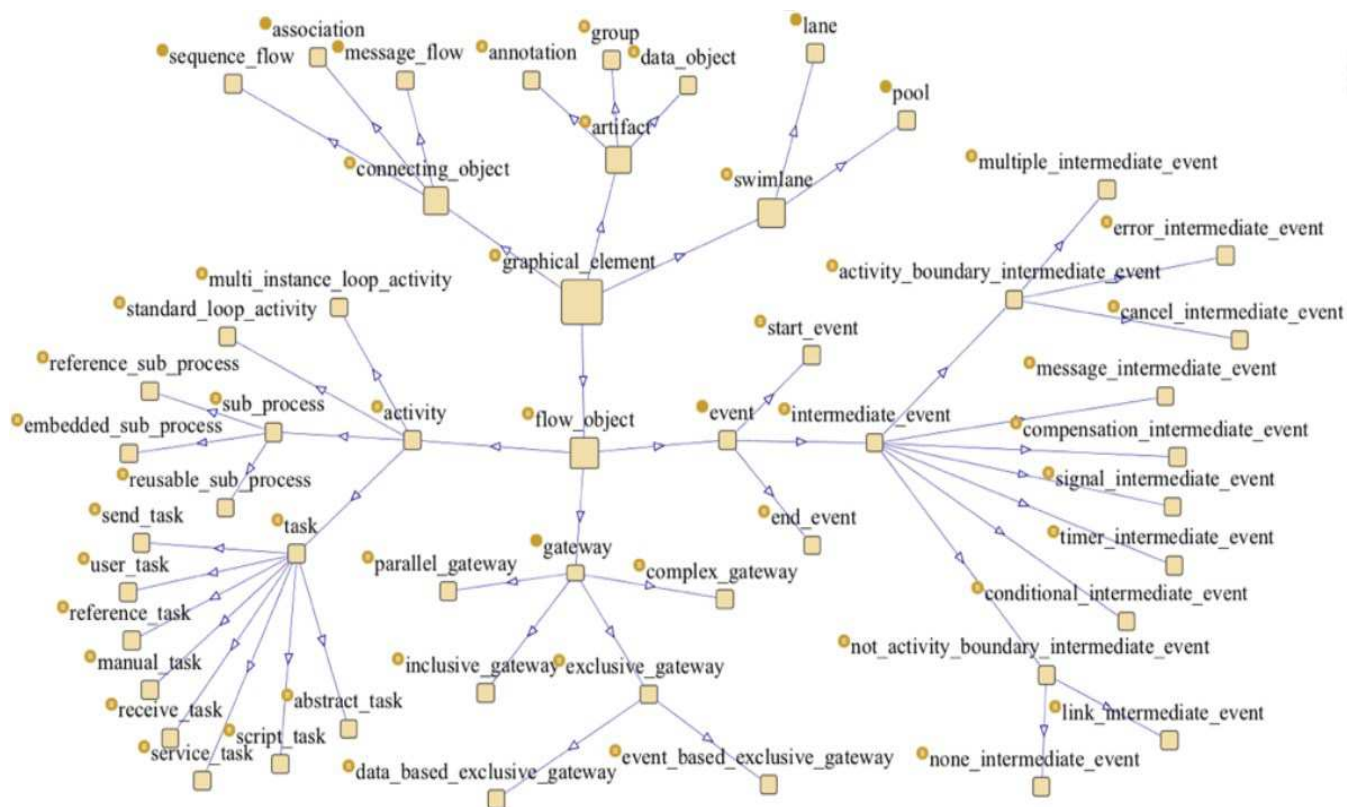
Figure 4.3 Hiérarchie des classes de BPMN 2 Ontology
