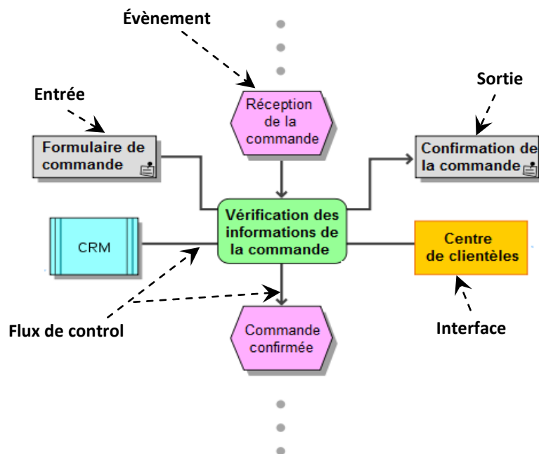
Figure 1.14 Processus de traitement des commandes modélisé en EPC.
