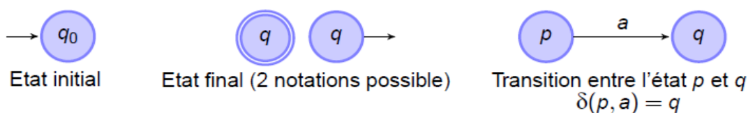
Figure 2.1 Les éléments constituant un automate
