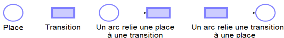
Figure 2.2 Les éléments constituant un réseau de Petri
