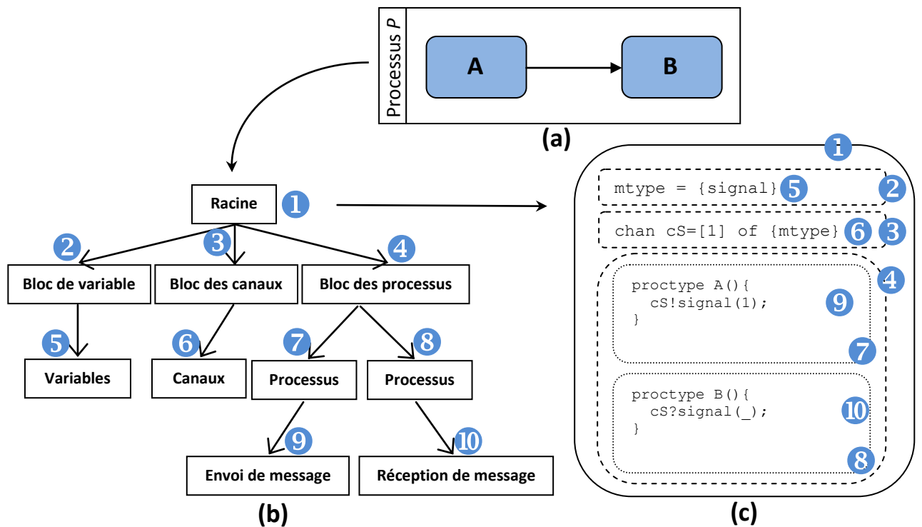
Figure 6.6 Exemple de l'arbre syntaxique.
