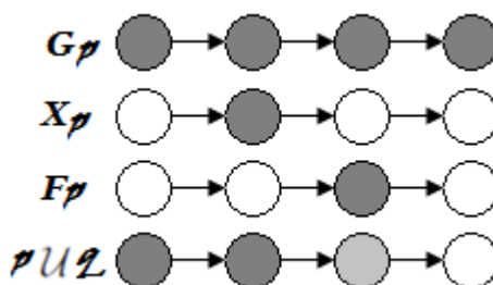
Figure 3.3 Les connecteurs temporels LTL.
