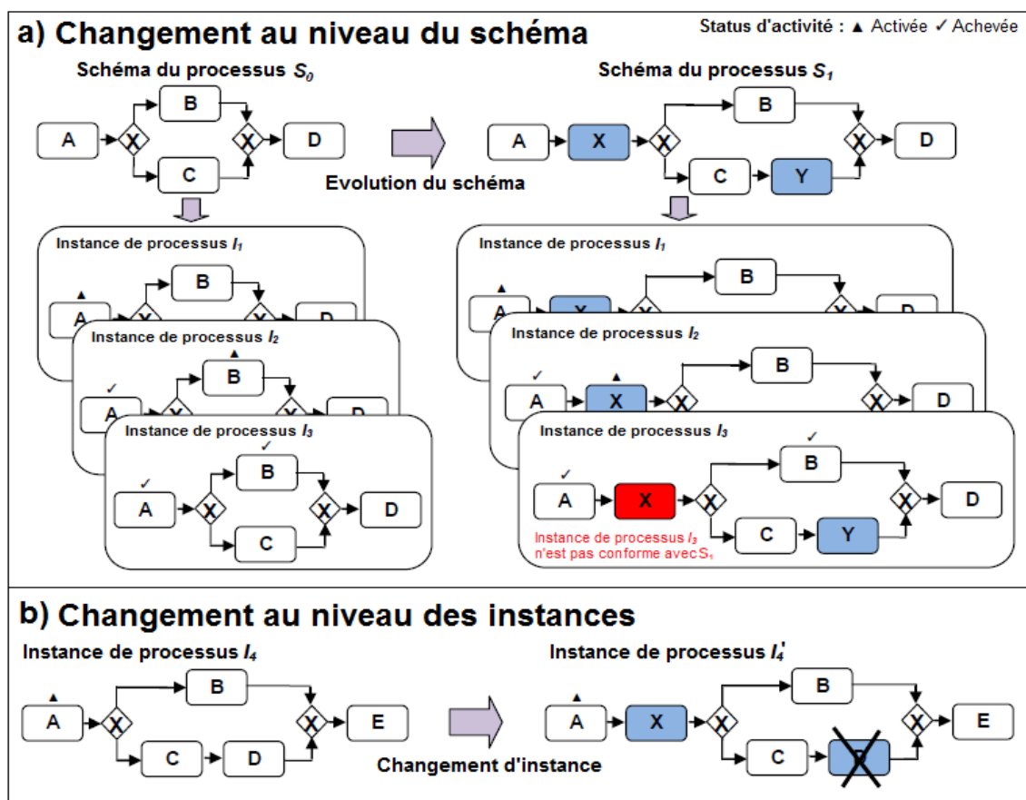
Figure 2.4 Niveaux de changement de processus
