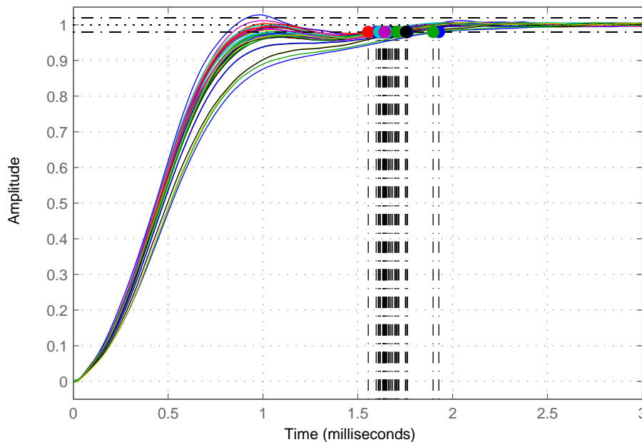
Figure 5.20 – Réponses indicielles des boucles fermées G_i K (1 + G_i K)^{-1} pour i \in [1, \dots, 35]
