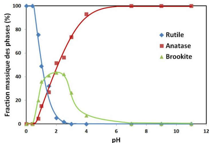
Figure 3.4 : fraction massique des phases de \text{TiO}_2 cristallisées en fonction du pH au cours du traitement hydrothermal ( \text{K/Ti} = 2 , T = 180^\circ\text{C} et t = 48 h)
