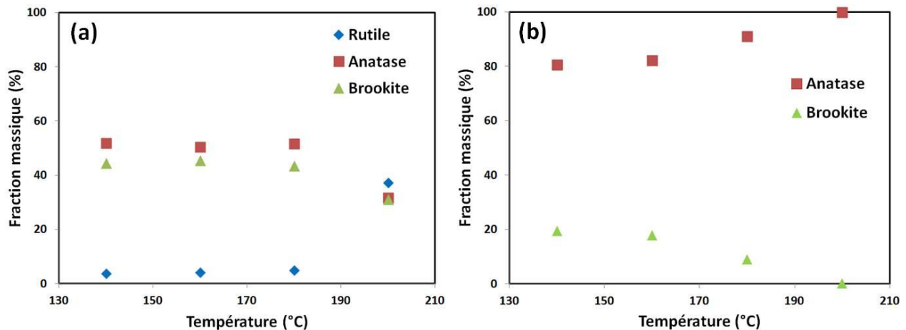
Figure 3.9 : fraction massique des phases en fonction de la température du traitement à pH = 2,0 (a) et pH = 4,0 (b) ( K/Ti = 2 et t = 48 h)
