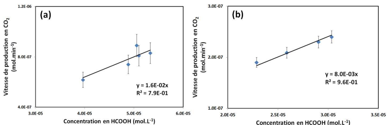
Figure 4.14 : vitesse de production en \text{CO}_2 en fonction de la concentration en acide formique, pour le P25 (a) et l'O39 (b) (0,4 vol. % méthanol, 1,0 \text{ g}\cdot\text{L}^{-1} en \text{TiO}_2 , 1,0 pds. % en Pt, photodépôt)
