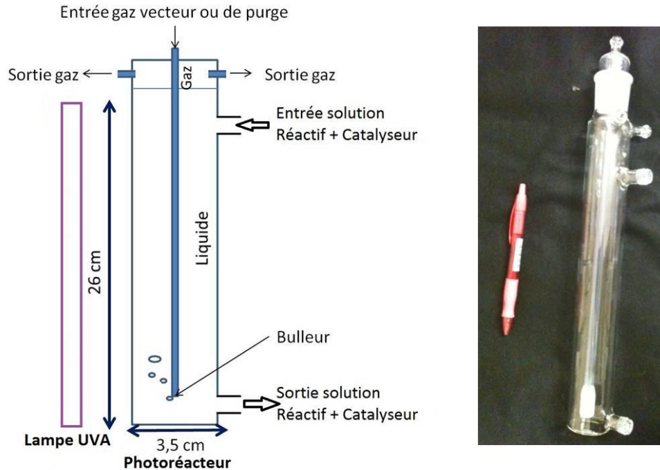
Figure 5.1 : Dimension d'un photoréacteur pour le couplage
