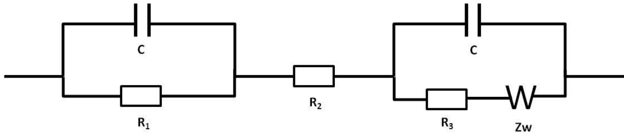
Figure 2.13 : Circuit équivalent 46
