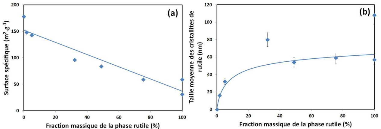
Figure 3.8 : Surface spécifique (a) et taille moyenne des cristallites de la phase rutile (b) en fonction de fraction massique de la phase rutile ( 0,0 \leq \text{pH} \leq 3,0 , \text{K}/\text{Ti} = 2 , \text{T} = 180^\circ\text{C} et t = 48 \text{ h} )
