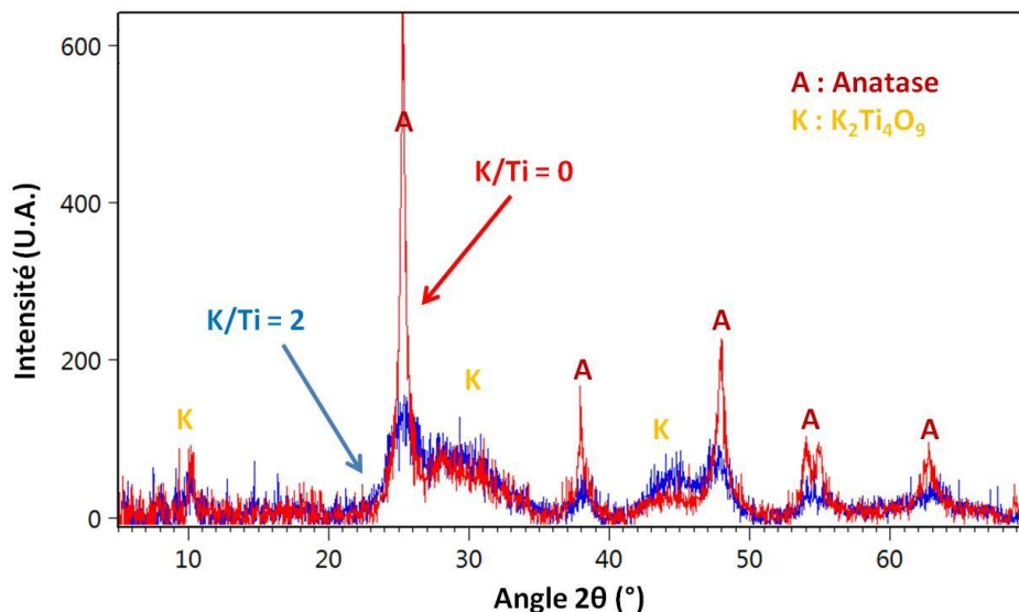
Figure 3.5 : Diffractogrammes des rayons X obtenus pour différents rapports molaires K/Ti (pH = 11,0, T = 180°C et t = 48 h)
