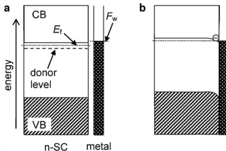
Figure 1.16 : Représentation d'un semiconducteur de type n et d'un métal (a) et du contact ohmique entre eux (b) 157
