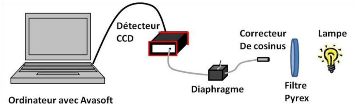
Figure 2.6 : Dispositif expérimental pour les mesures d'irradiance des lampes
