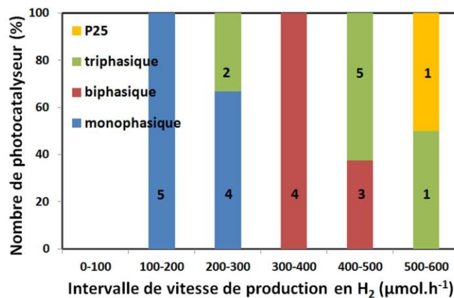
Figure 4.23 : Nombre de photocatalyseur en fonction de la vitesse de production en H 2 (100 vol. % méthanol, 1,0 g.L -1 en TiO 2 , 0,35 pds. % en Pt, imprégnation à échange d'ions)
