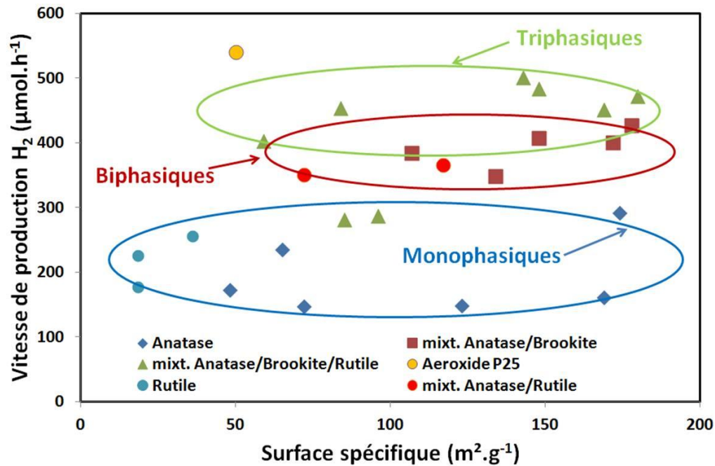
Figure 4.22 : Activité photocatalytique des différents types de photocatalyseur en fonction de la surface spécifique (100 vol. % méthanol, 1,0 g.L -1 en TiO 2 , 0,35 pds. % en Pt, impr. à échange d'ions)
