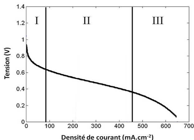
Figure 1.6 : Courbe de polarisation classique d'une pile à combustible 48
