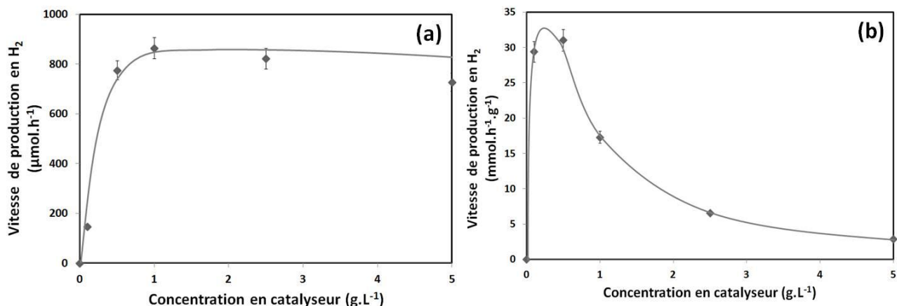
Figure 4.2 : vitesse de production en hydrogène (a) et vitesse de production spécifique (b) en fonction de la concentration en catalyseur (100 vol. % en méthanol, 1,0 pds. % en Pt, photodépôt)
