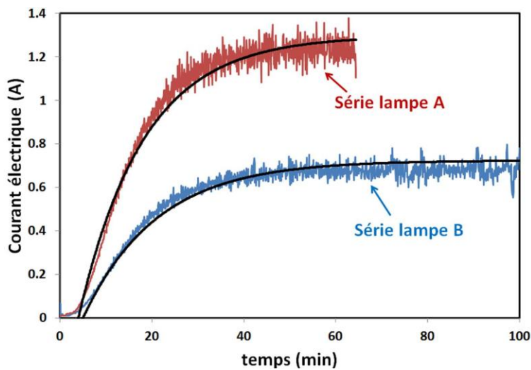
Figure 5.9 : Courants limites obtenus à 220 mV pour deux flux de photons, déshydrogénation du méthanol, 1 \text{ g}\cdot\text{L}^{-1} en Pt/TiO 2 à 1,0 pds. % Pt, PEMFC avec Pt à l'anode, système photocatalytique B
