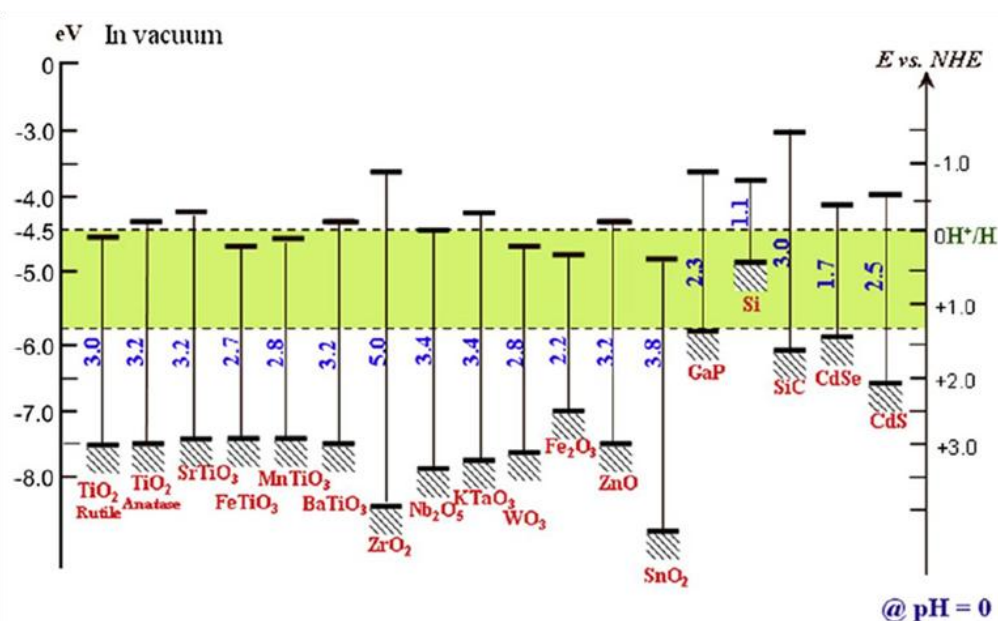
Figure 1.19 : Position des bandes de valence et de conduction, et largeur de la bande interdite pour différents semiconducteurs étudiés en photocatalyse, par rapport au potentiel de l'eau 187
