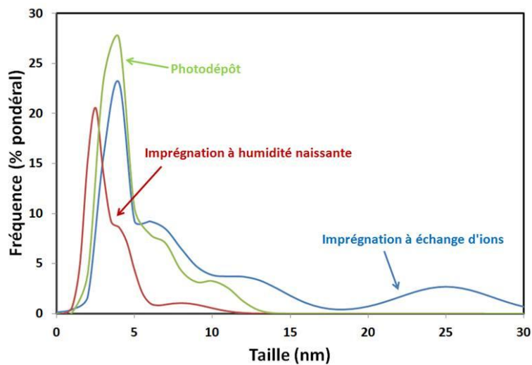
Figure 3.26 : Distribution en taille des particules de platine pour les différentes méthodes de dépôt sur le P25 ( 0,38 \pm 0,03 pds. % en Pt)
