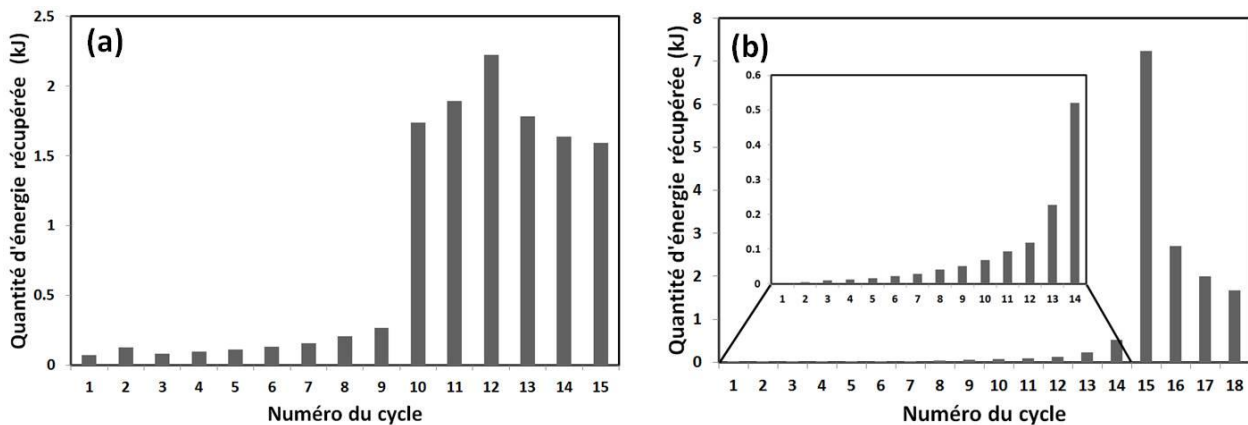
Figure 5.13 : Quantité d'énergie récupérée en fonction du cycle (pour P \geq 0,12 W) pour la déshydrogénation du méthanol (a) et le reformage du méthanol à 50 vol.% (b), PEMFC avec Pt à l'anode sous 1,1 bar
