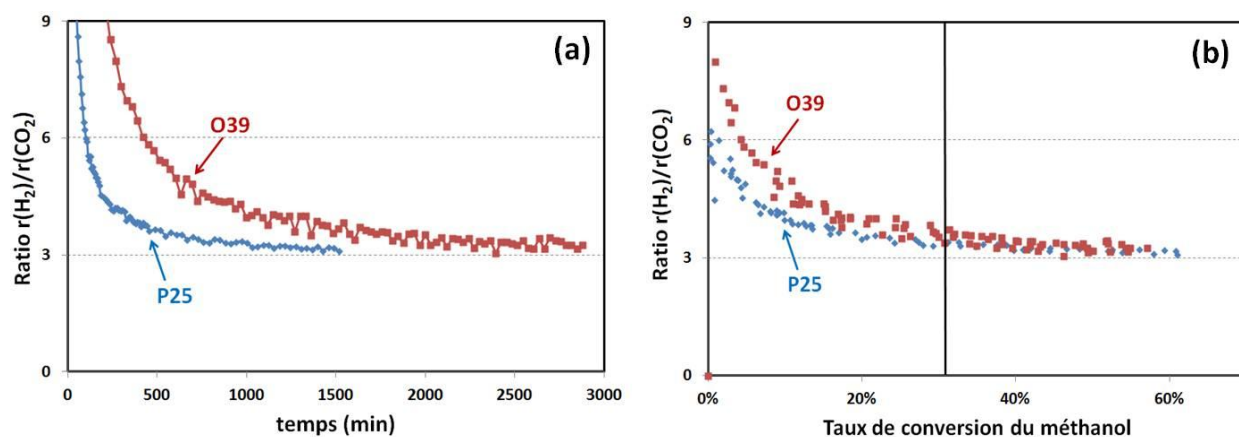
Figure 4.10 : Ratio des vitesses de production r(\text{H}_2)/r(\text{CO}_2) en fonction du temps (a) et du taux de conversion du méthanol (b) (0,4 vol. % méthanol, 1,0 g.L -1 en TiO 2 , 1,0 pds. % en Pt, photodépôt)
