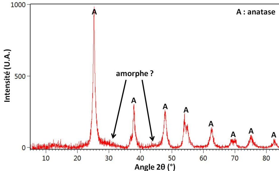
Figure 3.13 : Diffractogramme des rayons X de l'échantillon initial d'anatase (pH = 9,0, K/Ti = 2, T = 180°C et t = 48 h)
