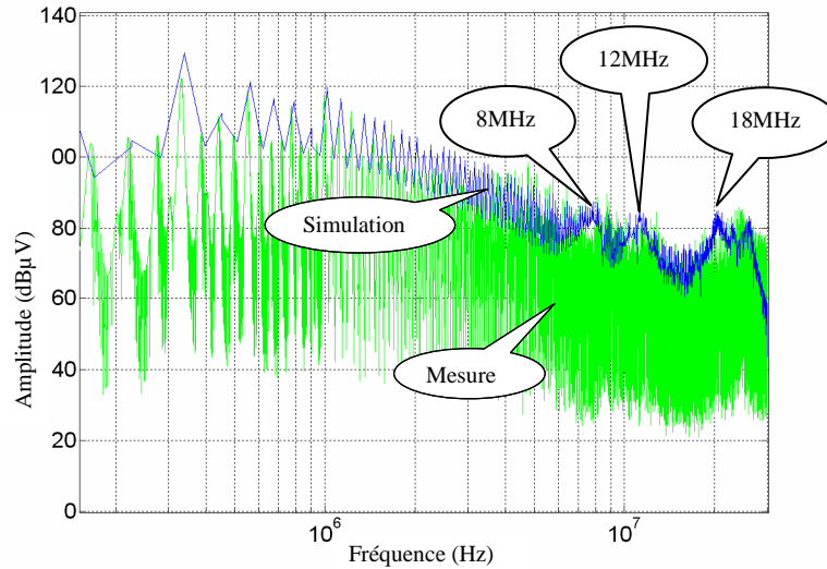
Figure 86 : Comparaison entre la simulation et la mesure du spectre électromagnétique du convertisseur complet sans filtre
