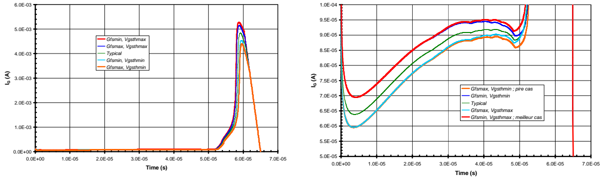
Figure 66 : Influence des paramètres électriques de MBS sur la commande optimisée
