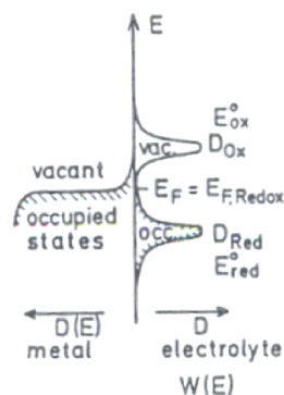
Figure A.3.5 : Schéma du transfert de charge à une électrode métallique en équilibre avec un couple rédox, d'après Gerischer [Ger85] .
