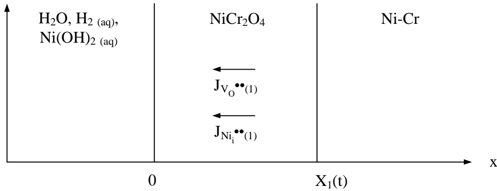
Figure 5.2 : Schéma du sous-système Ni-Cr / \text{NiCr}_2\text{O}_4 / \text{H}_2\text{O} , \text{H}_2 (aq), \text{Ni(OH)}_2 (aq) tel que modélisé au paragraphe 2.1.
