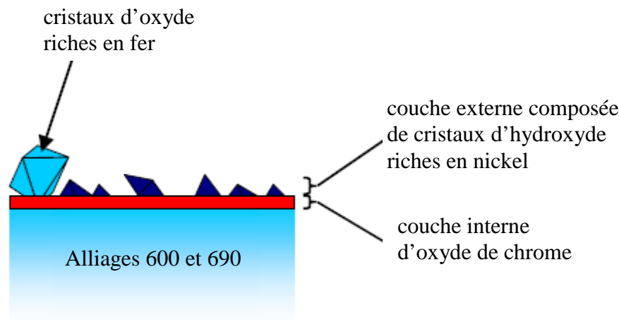
Figure 1.1 : Schématisation de la couche d'oxyde formée sur les alliages 600 et 690 corrodés en milieu aqueux (composition indiquée dans le tableau A.1.1 figurant en annexe 1) à 325^{\circ}C , d'après Machet [Mac04a] .
