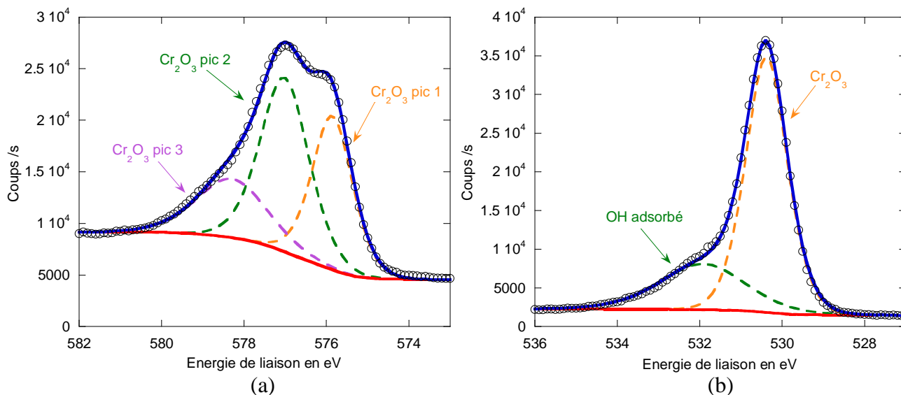
Figure 3.29 : Spectres des niveaux de cœur 2p_{3/2} du chrome (a) et 1s de l'oxygène (b), obtenus sur une couche de \text{Cr}_2\text{O}_3 , sans correction des effets de charge ( E_{C1s} = 285,1 eV).
