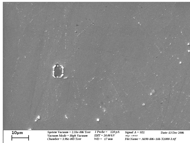
Figure 4.11 : Observations par MEB, en électrons secondaires, de la surface de la couche d'oxyde se formant sur l'alliage 690 exposé en milieu de type primaire à 325 °C, durant 406 heures en boucle à recirculation en conditions optimales de fonctionnement des résines échangeuses d'ions puis pendant 144 heures en autoclave en TA6V.
