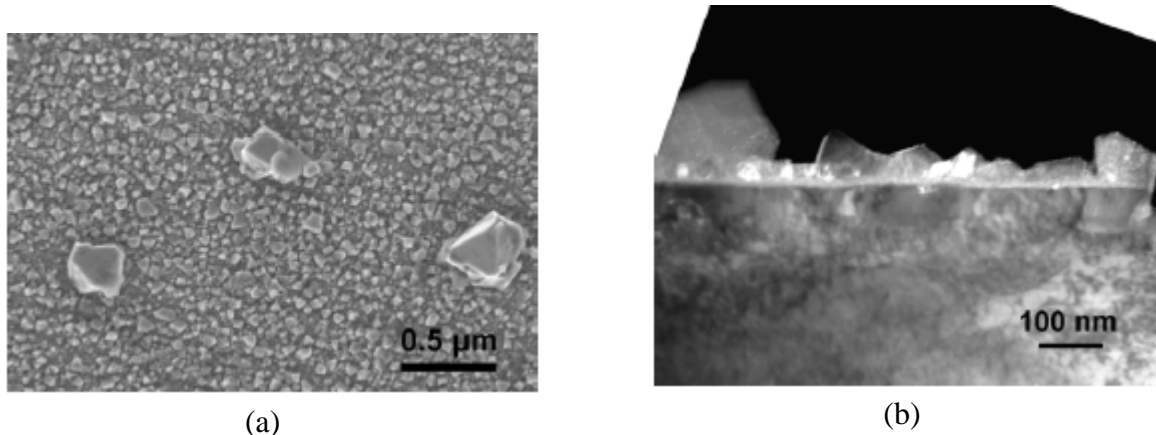
Figure 1.2 : Observations des couches d'oxyde se formant sur l'alliage 600 exposé 300 heures en milieu de type primaire (composition exacte indiquée dans le tableau A.1.2) à 360 °C, (a) vue de surface observée par MEB-FEG et (b) coupe transverse observée au MET, d'après Panter [Pan02] .
