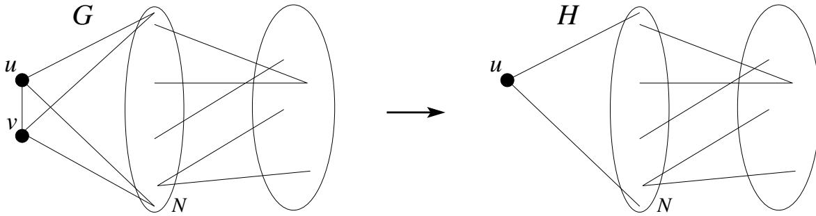
FIGURE 5.7: Identification de deux sommets (u, v) simpliciaux et vrais jumeaux. N est le voisinage des sommets u et v .
