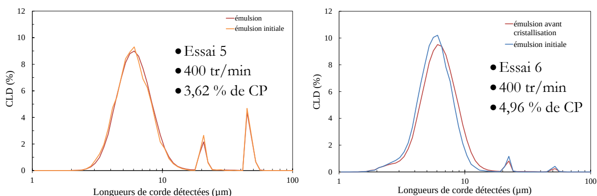
Figure V.24 Essais 5 et 6 : Evolution de la CLD de l'émulsion CP + eau avant cristallisation
