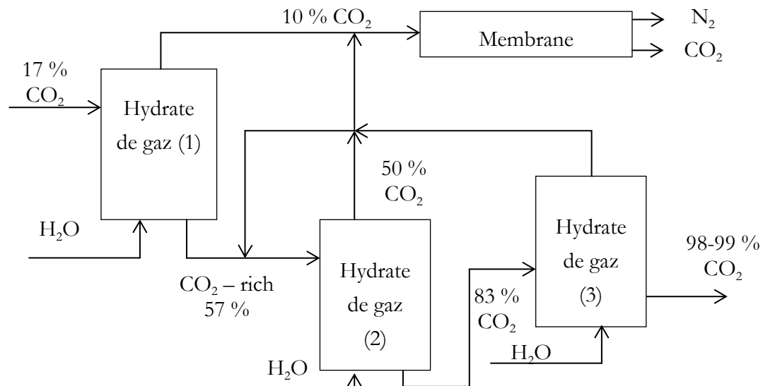
Figure I.8 Procédé de séparation hybride pour le captage en postcombustion proposé par Linga et al. (2007b)
