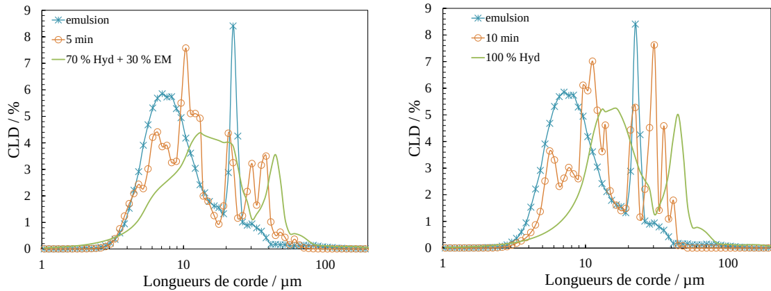
Figure V.39 Essai 13 : Comparaison entre les CLDs simulées et expérimentales
