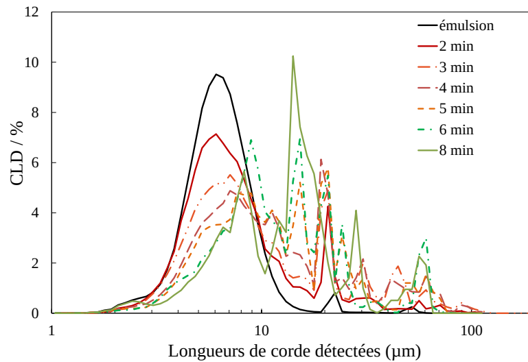
Figure V.29 CLDs de l'essai 5 à différents temps t de cristallisation
