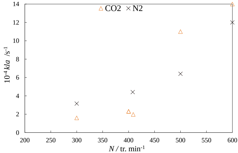
Figure IV.5 Evolution de la constante de transfert gaz/liquide k_{Lw} a du CO_2 ou de N_2 en fonction de la vitesse d'agitation N dans l'eau pure
