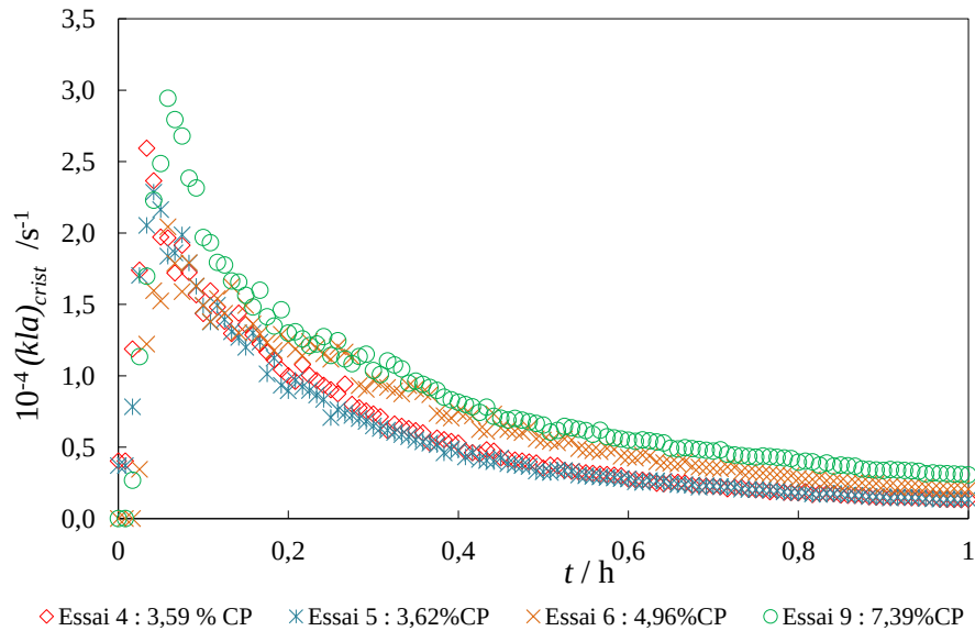
Figure IV.16 Evolution de la constante globale de transfert (k_{Lw}a)_{crist} en fonction du temps durant la cristallisation, essais 4, 5, 6, 9 où t_{ind} > 1 h et N=400 \text{ tr.min}^{-1}
