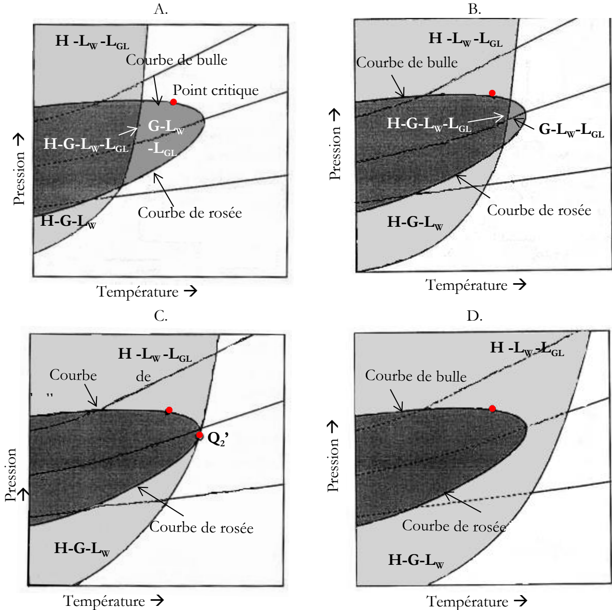
Figure I.7 Diagrammes de phases modifiés d'après Diamond (1994) 4 fractions molaires en azote dans la phase gazeuse (de A à D, y_{N_2} augmente)
