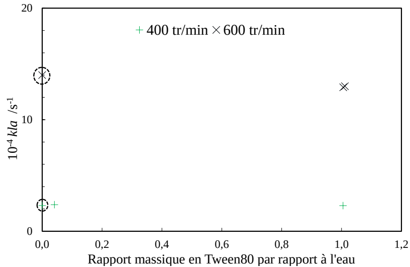
Figure IV.6 Evolution de la constante de transfert gaz/liquide du CO_2 en fonction de la vitesse d'agitation N et du rapport massique en Tween80®, émulsion CP/eau à w_{CP,0}^{EM} = 3,6 \% .
