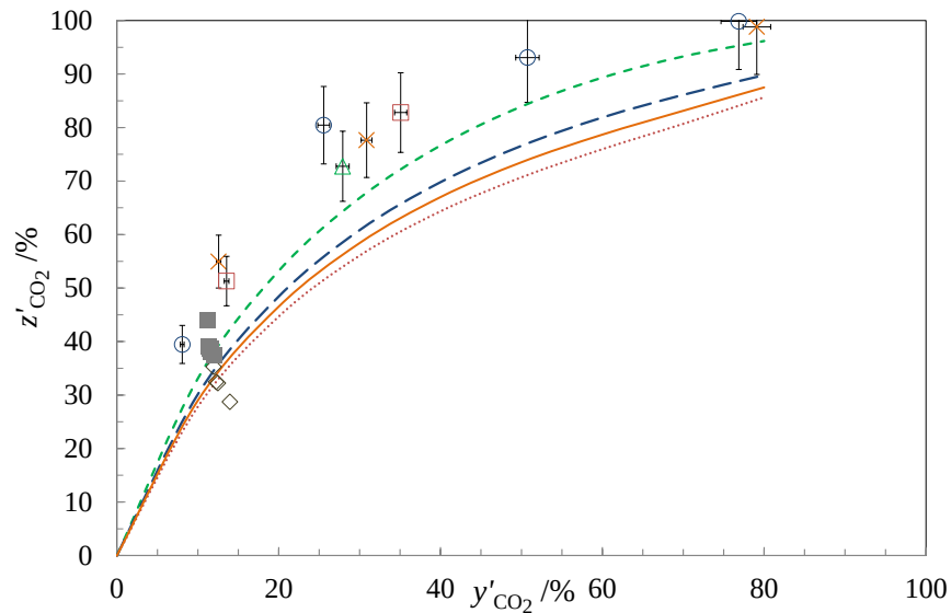
Figure III.8 Fraction molaire en CO 2 dans l'hydrate z'_{CO_2} en fonction de la fraction molaire en CO 2 y'_{CO_2} dans le gaz à l'équilibre à différentes températures.
