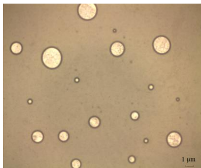
Figure II.12 Gouttelettes de CP dispersées dans l'eau : cas de l'émulsion en présence d'IPE
