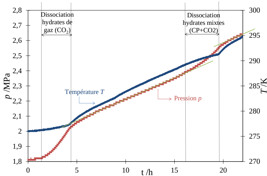
Figure II.18 Dissociation des hydrates : évolutions de la pression et de la température en fonction du temps (CO 2 pur, émulsion CP/eau avec w_{CP,0}^{EM}=1,84\% )
