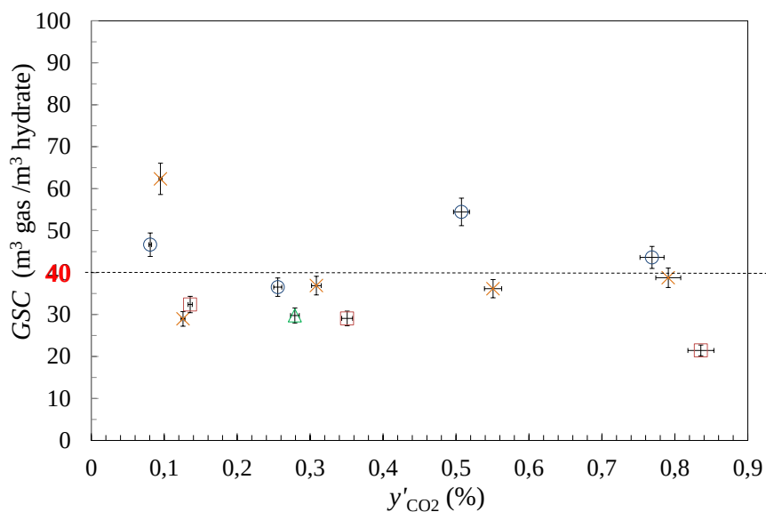
Figure III.11. Volume de gaz stocké GSC dans les hydrates mixtes de CO_2 + N_2 + CP à différentes températures T et compositions de la phase gazeuse à l'équilibre y'_{CO_2} .
