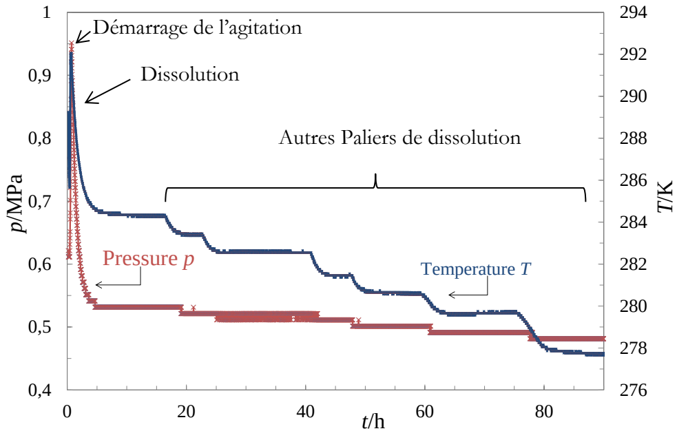
Figure II.16 Evolution de la pression et de la température de la phase liquide au cours de la dissolution du \text{CO}_2 dans une émulsion CP/eau avec w_{\text{CP},0}^{\text{EM}} = 27,80\%
