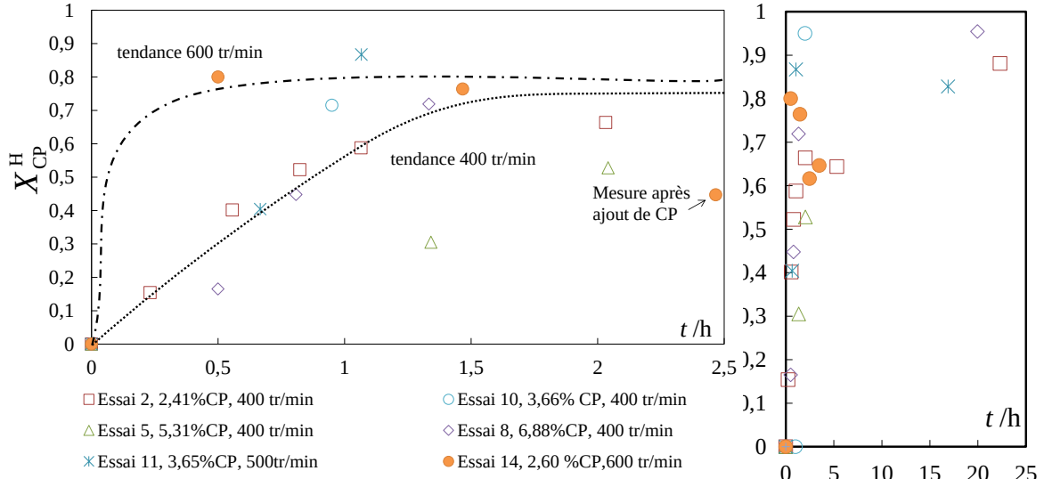
Figure IV.13 Evolution du taux de conversion du CP X_{CP}^H à différents temps t de cristallisation (essais 2, 7, 8, 10, 11 et 14)
