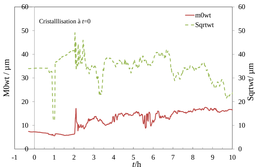
Figure VI.38 Essai 10 : Evolution de la longueur de corde moyenne pondérée en nombre (mean No wt) et en surface (mean No sqrt) en fonction du temps t
