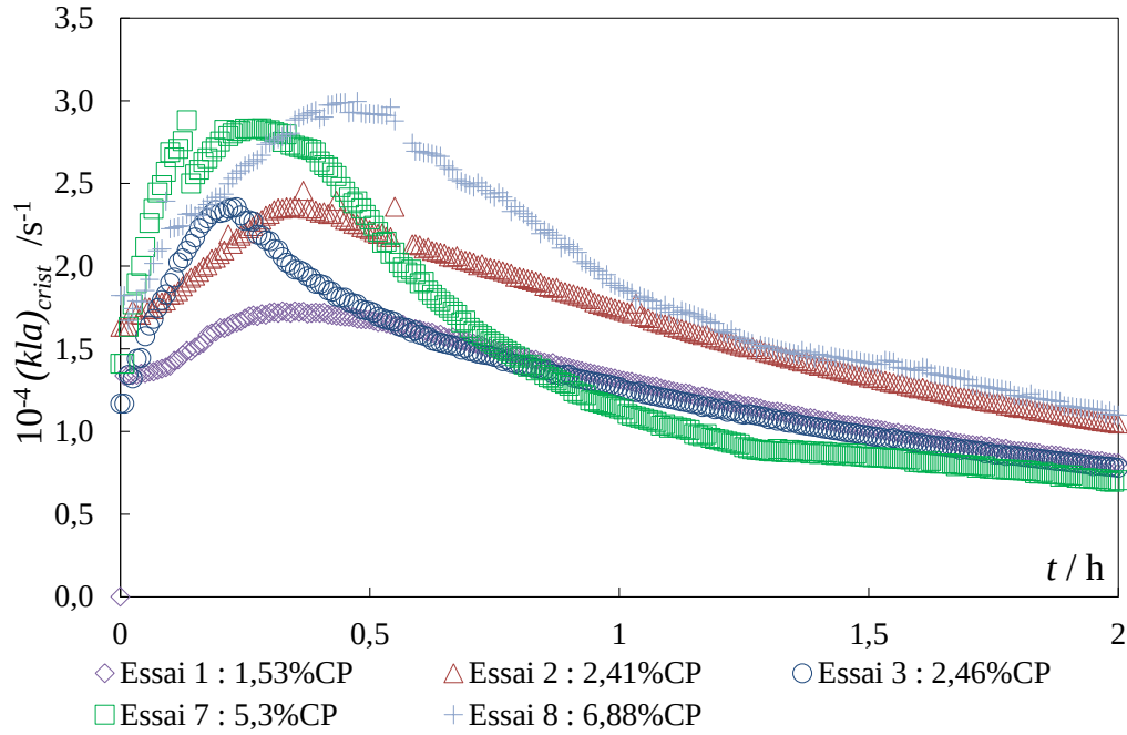
Figure IV.14 Evolution de la constante globale de transfert (k_{Lw}a)_{crist} en fonction du temps de cristallisation, essais 1, 2, 3, 7, 8 où t_{ind} < 1 h et N=400 tr.min -1
