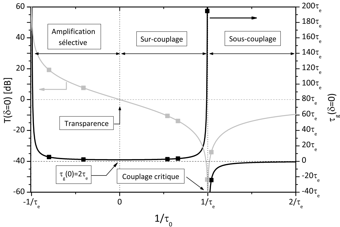
FIGURE 4.13 – Transmission T(0) et le retard de groupe \tau_g(0) à résonance en fonction 1/\tau_0 pour une microsphère de diamètre 145 \mu\text{m} dopée Erbium à 0,1\% molaire. Les résultats en amplification sélectives viennent de la partie 3.9.1.
