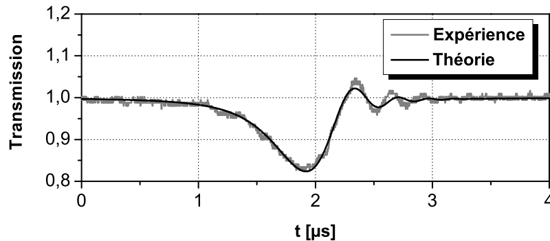
FIGURE 2.16 – Mesure CRDM d'une résonance du résonateur n° 1 dans un cas de sous-couplage. En bleu la mesure expérimentale, en rouge l'ajustement théorique.
