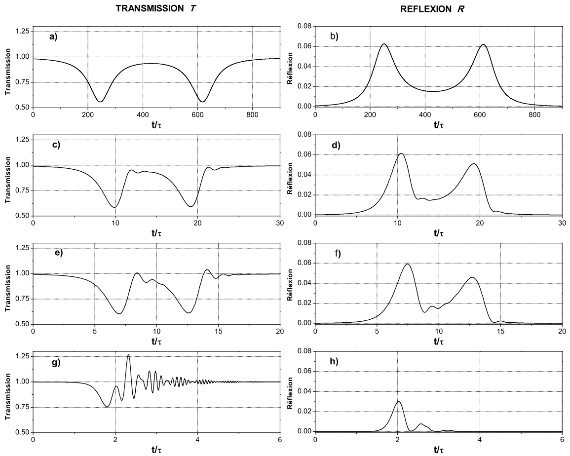
FIGURE 5.3 – Simulation de la transmission T(t) et de la réflexion R(t) en régime de couplage modal dans le cas où \gamma = \tau/10 et \tau_0 = \tau_e/3 pour différentes vitesses de balayage. (a)-(b) \tilde{V}_s = 0.015\tilde{V}_0 , (c)-(d) \tilde{V}_s = 0.6\tilde{V}_0 , (e)-(f) \tilde{V}_s = \tilde{V}_0 , (g)-(h) \tilde{V}_s = 20\tilde{V}_0 . L'axe des abscisses est normalisé par rapport au temps de vie globale \tau .
