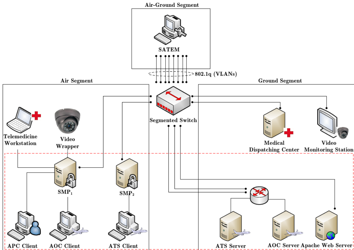
Figure 13 : environnement aéronautique émulé
