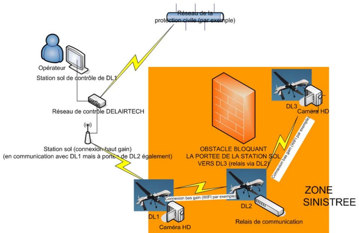
Figure 37 : scénario d'application (télésurveillance distribuée)
