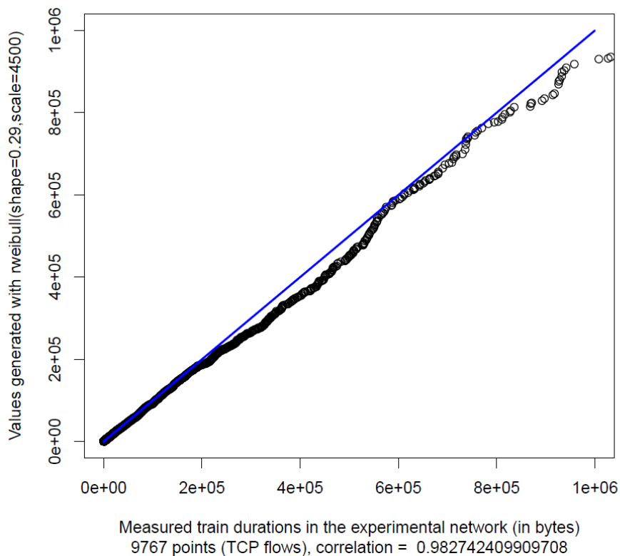
Figure 6 : QQPlot pour la série des Don (trafic réel vs trafic généré)
