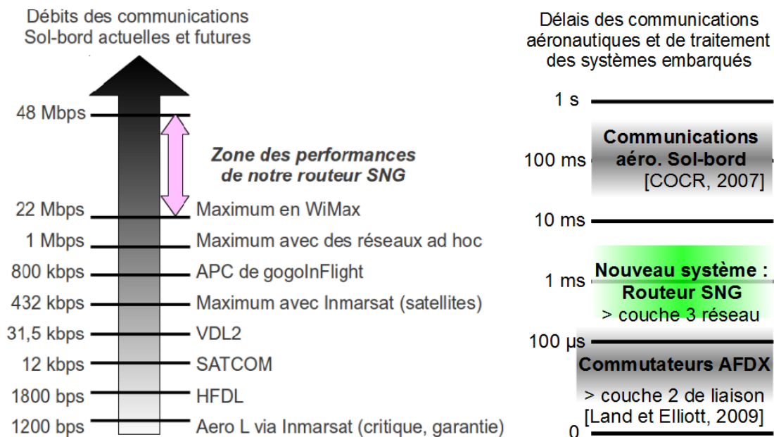
Figure 25 : performances globales du système SNG
