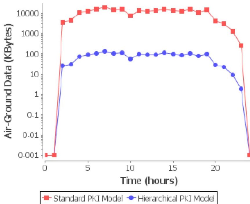
Figure 19 : utilisation des ressources du lien sol-bord
