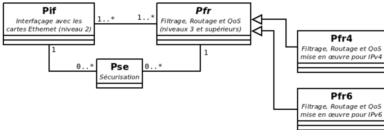
Figure 22 : diagramme de classes du routeur SNG
