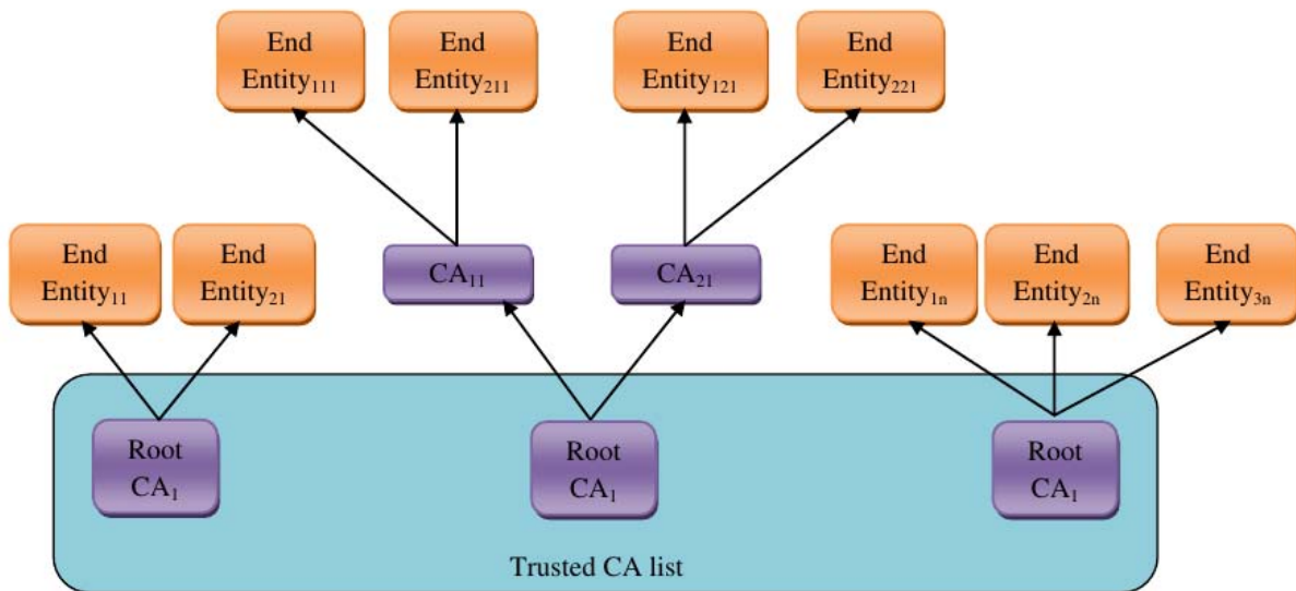
Figure 15 : modèle générique de PKI hiérarchique comportant plusieurs racines
