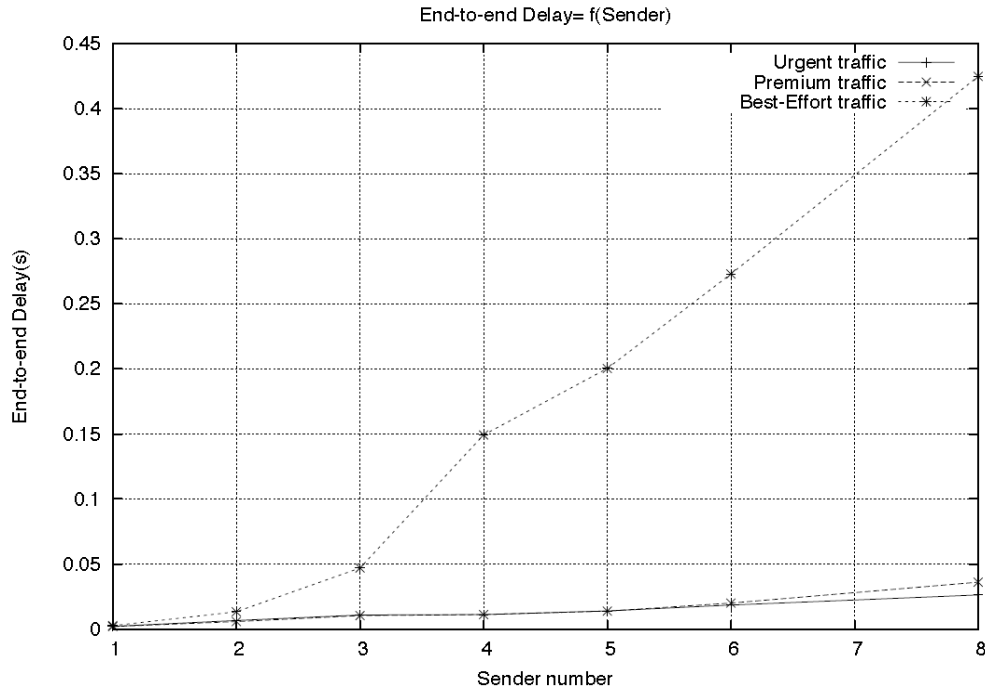
Figure 35 : délai de bout en bout en fonction du nombre d'émetteurs par type de service
