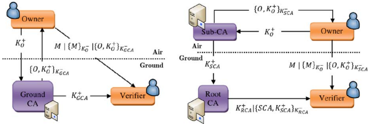
Figure 16 : architectures de PKI: référence Internet (à gauche) vs. PKI aéronautique hiérarchique (à droite)
