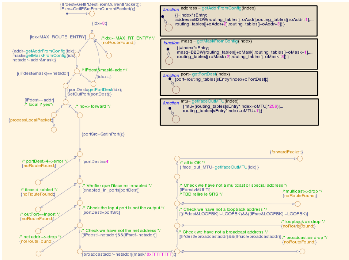
Figure 24 : diagramme à états-transitions de routage des paquets IPv4
