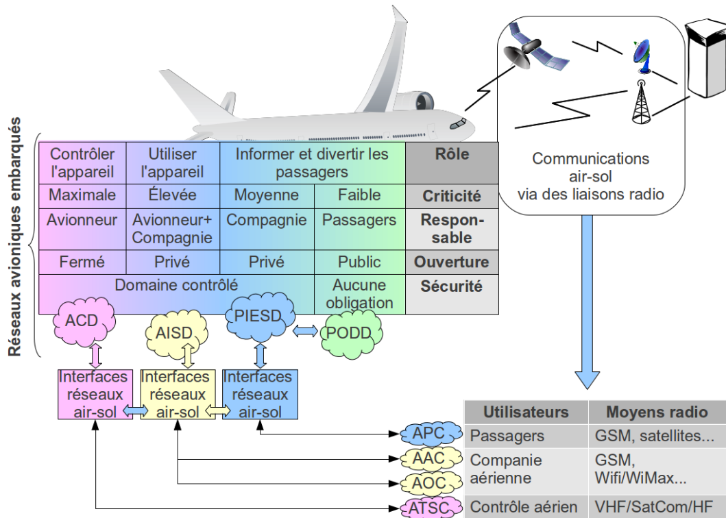
Figure 1 : réseaux avioniques et aéronautiques
