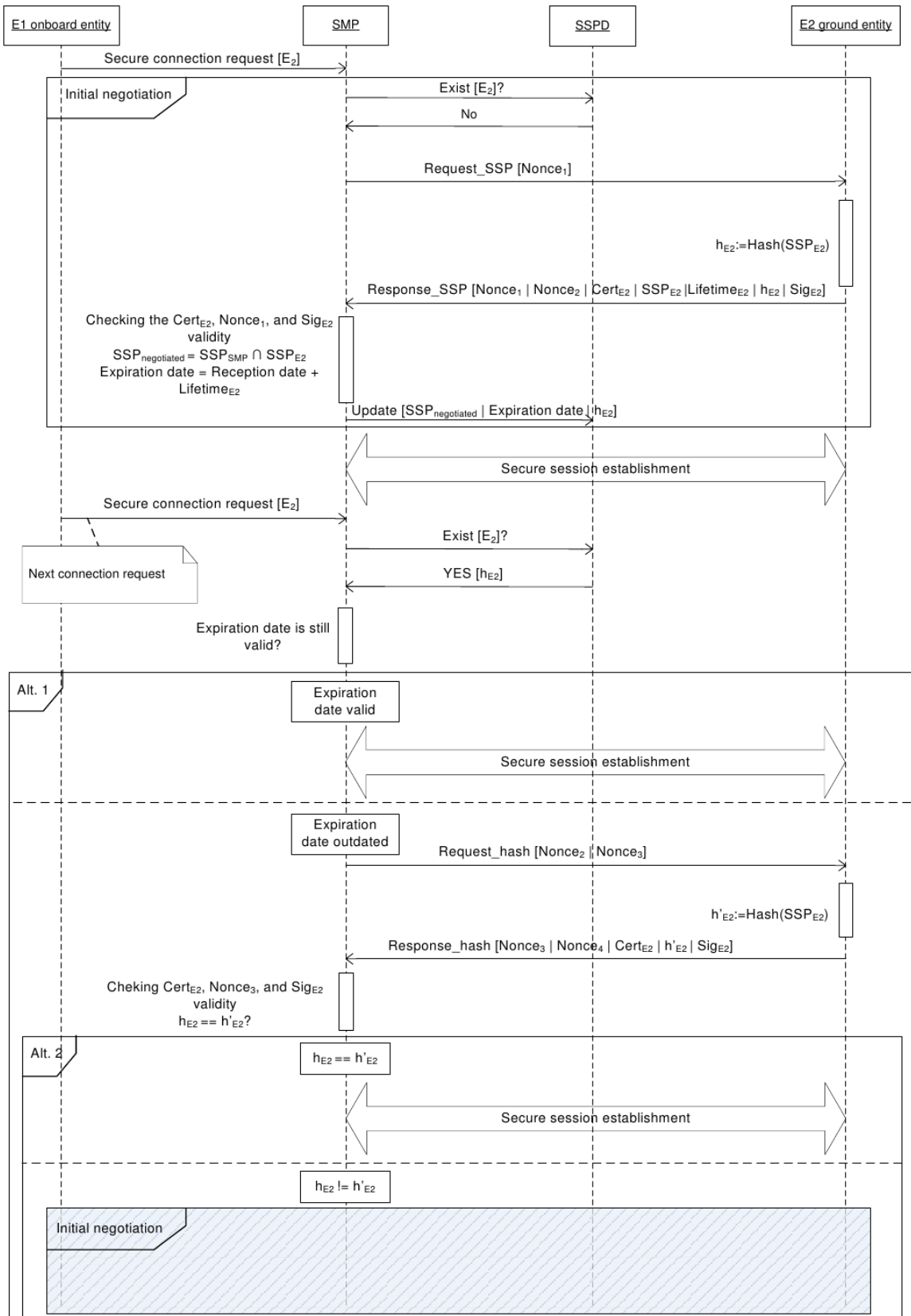
Figure 12 : fonctionnement du protocole SSP
