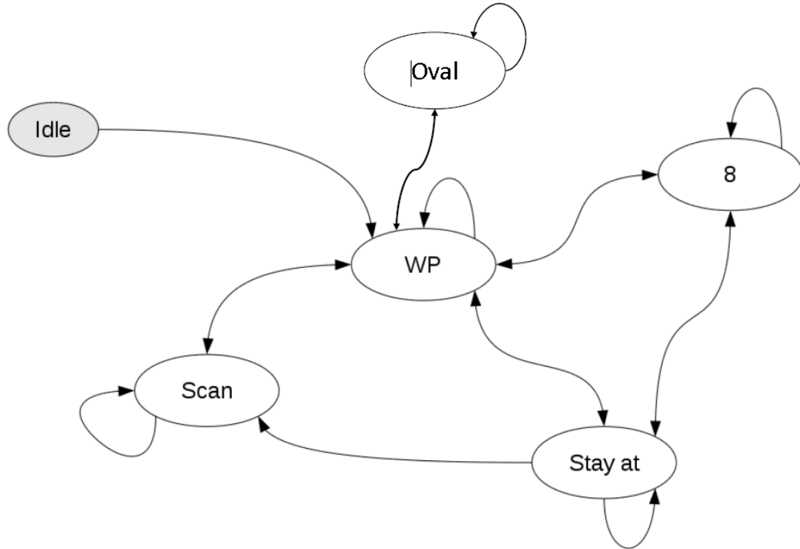
Figure 33 : principes de déplacement pour le modèle Paparazzi (PPRZM)
