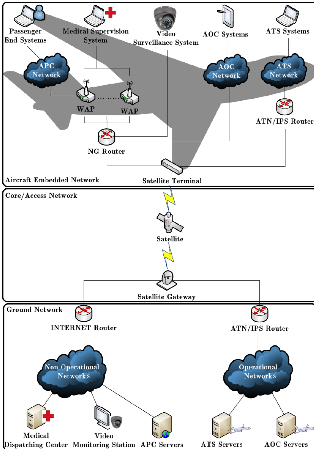
Figure 2 : exemple de mutualisation des communications au travers d'un lien satellite unique
