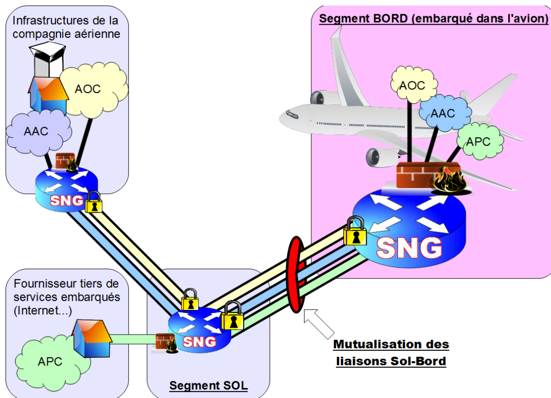
Figure 21 : exemple de déploiement du routeur SNG dans le contexte aéronautique
