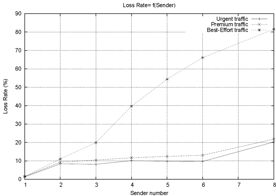
Figure 36 : taux de perte en fonction du nombre d'émetteurs par type de service
