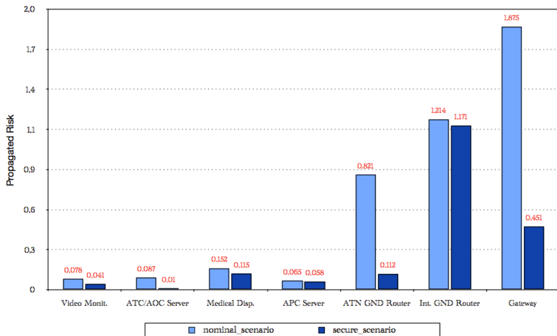
Figure 30 : niveau de risque des différentes entités présentes dans le réseau AeroMACS : topologie initiale #1 vs. topologie évoluée et plus sécurisée #2
