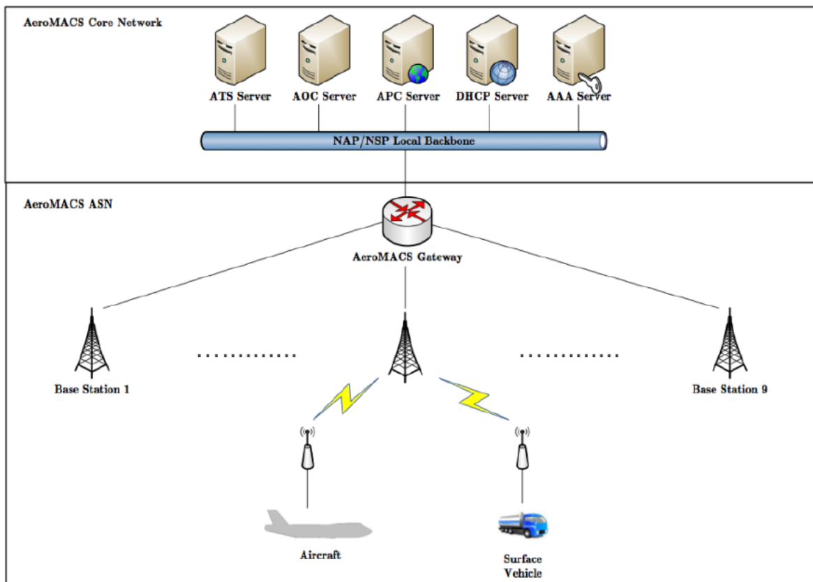
Figure 28: topologie du réseau AeroMACS (topologie #1)
