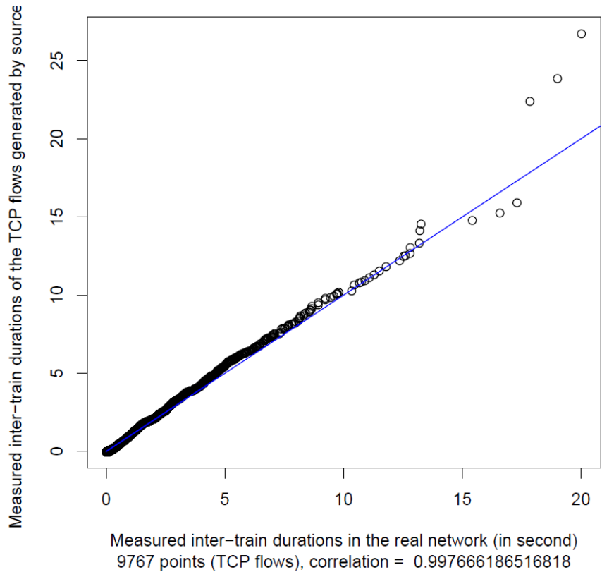
Figure 5 : QQPlot pour la série des Doff (trafic réel vs trafic généré)
