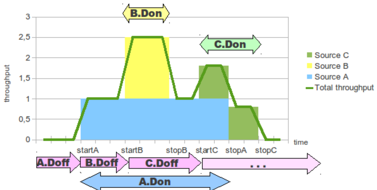
Figure 4 : principes de génération des flux APC à l'aide de sources ON-OFF
