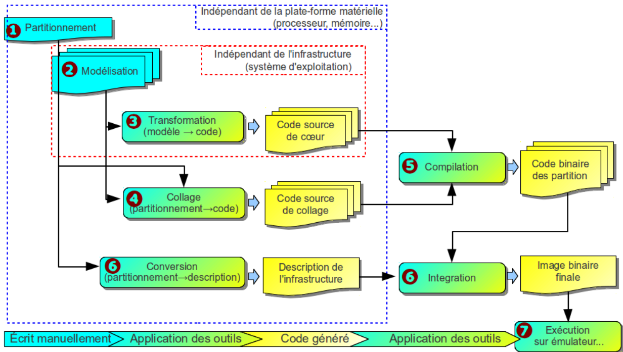
Figure 20 : méthodologie de développement orientée modèle pour les systèmes embarqués complexes
