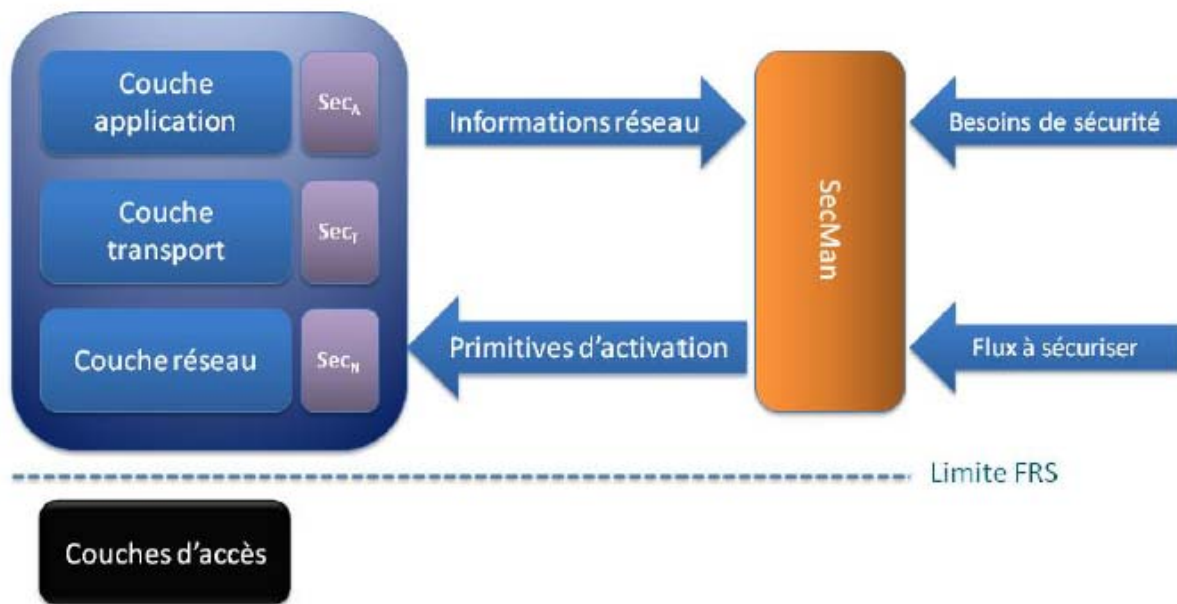
Figure 9 : principes de fonctionnement de SecMan
