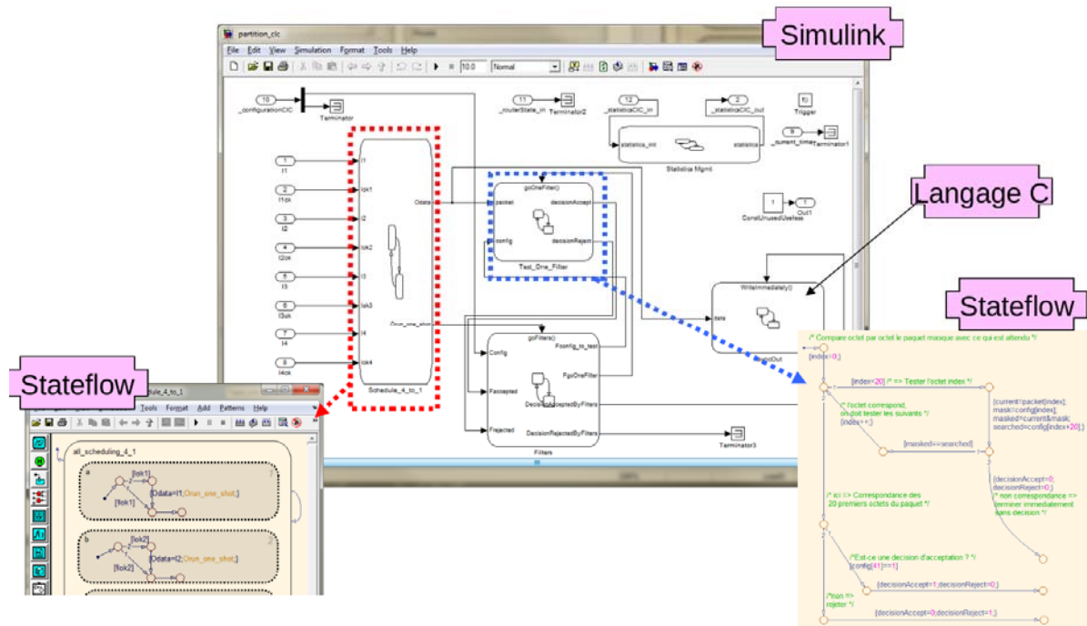
Figure 23 : modélisation de la classe Pfr4 du routeur SNG à l'aide de diagrammes Simulink et Stateflow
