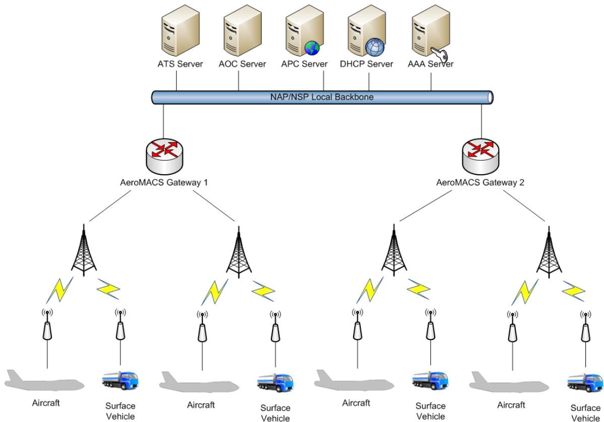
Figure 29 : proposition d'évolution de la topologie réseau AeroMACS (topologie #2)
