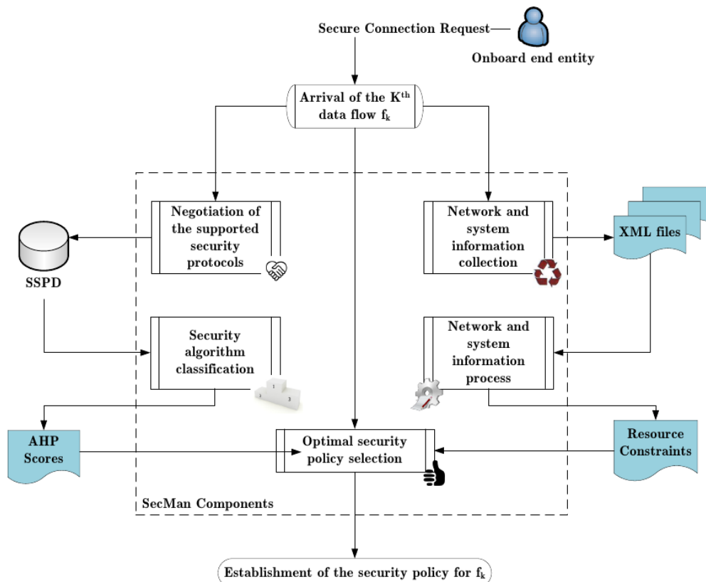
Figure 11 : algorithme de sélection de la politique de sécurité optimale du SecMan
