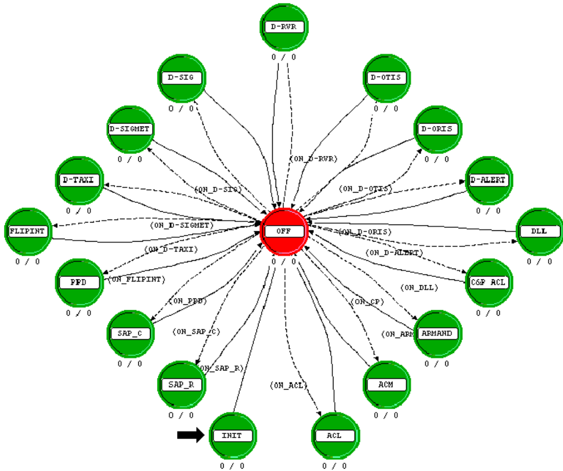
Figure 3 : modélisation à l'aide de machines à états (exemple du trafic ATSC)
