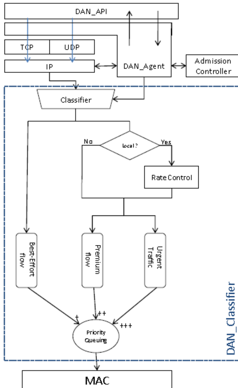
Figure 32 : mécanismes déployés dans l'architecture DAN
