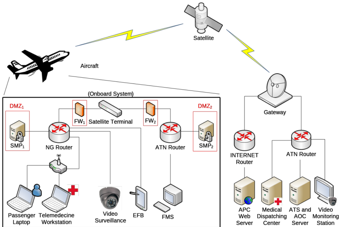
Figure 7 : déploiement du module SecMan (SMP) dans le cadre du projet FAST
