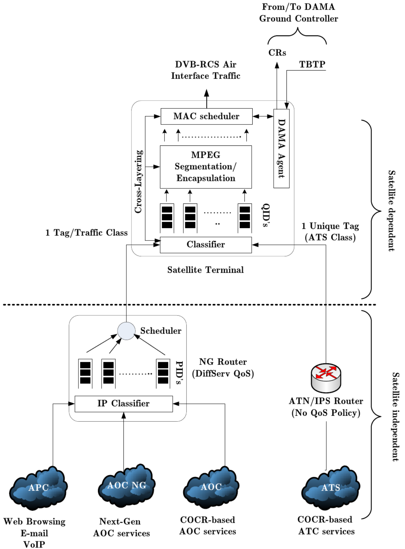
Figure 8 : gestion de la QoS dans le projet FAST
