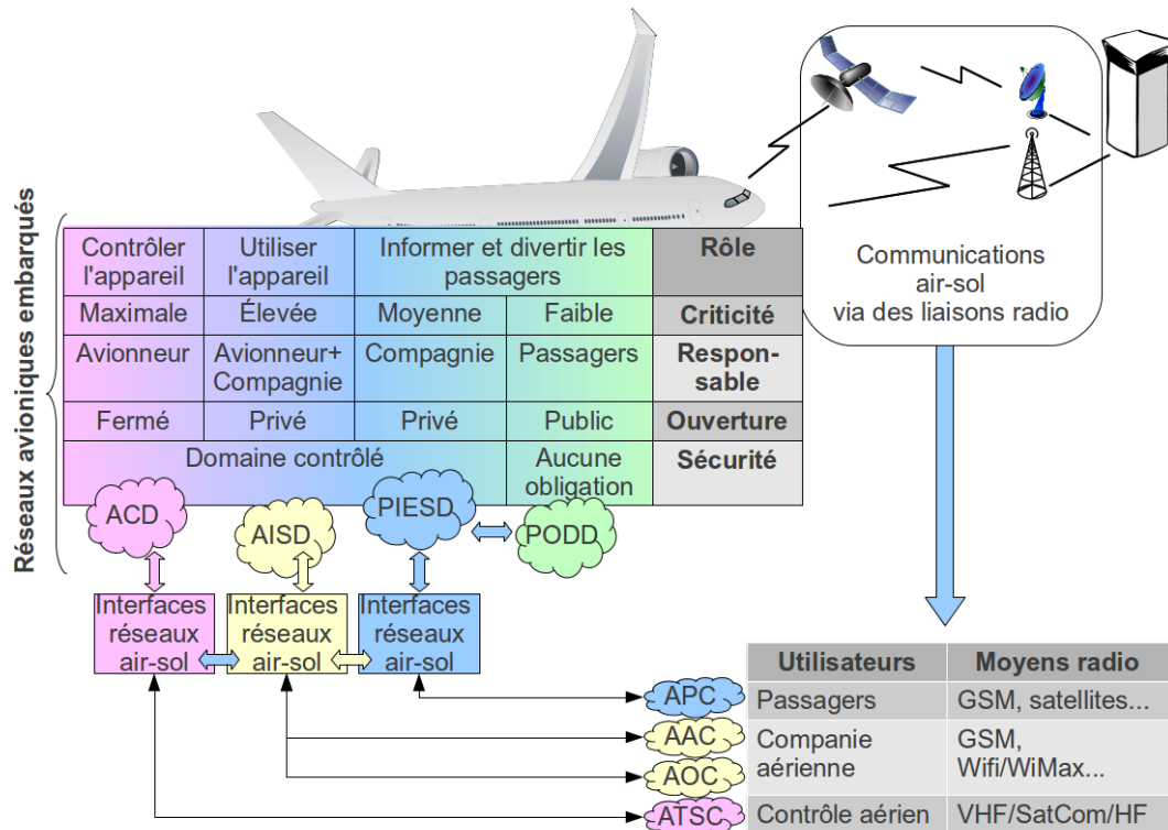
Figure 1 : réseaux avioniques et aéronautiques
