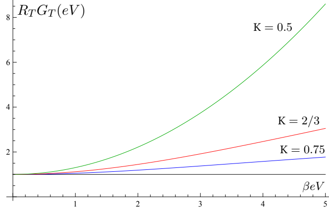
FIGURE II.6 – Conductance différentielle à travers une barrière tunnel en unité de R_T la conductance différentielle à polarisation nulle en fonction de \beta eV pour K = 1 (noire), K = 0.8 (bleue), K = 2/3 (rouge), K = 0.5 (vert).
