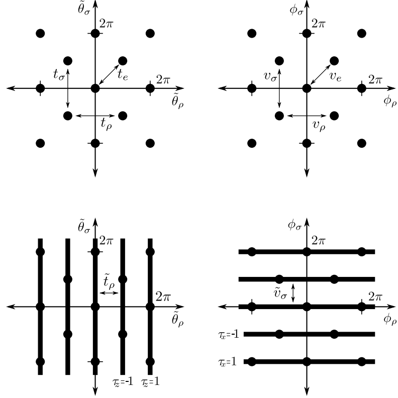
FIGURE III.2 – Schéma des processus de tunneling et de faible rétrodiffusion pour les quatre point fixes, avec, de gauche à droite et de bas en haut les points fixes (Conducteur-Conducteur), (Isolant-Isolant), (Isolant-Conducteur) et (Conducteur-Isolant).
