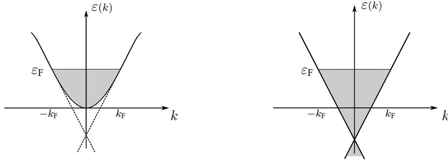
FIGURE II.1 – A gauche spectre d’une particule dans un réseau, à droite spectre linéarisé
