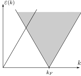
FIGURE II.2 – Spectre d'excitation à une dimension
