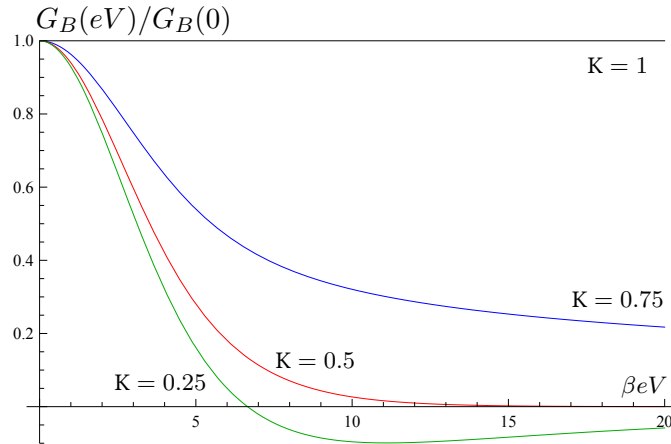
FIGURE II.8 – Ratio entre la conductance différentielle dans le régime de faible rétrodiffusion et sa valeur à polarisation nulle G_B^0(0) , en fonction de \beta e V , pour K = 1 (noire), K = 0.75 (bleue), K = 0.5 (rouge) et K = 0.25 (vert). Pour \beta e V \ll 1 on retrouve bien une loi de puissance en e V^{2K-2} . Pour K = 0.5 , le courant de rétrodiffusion sature.
