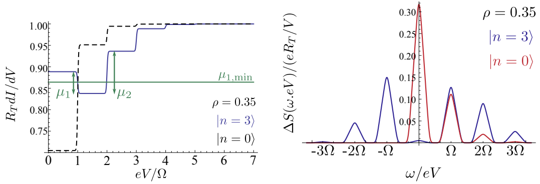
FIGURE VI.4 – À gauche, conductance différentielle d’une jonction tunnel couplée à un oscillateur peuplé par un état de Fock pour \rho = 0.35 , n = 2 . La température électronique est telle que \beta eV = 100 . La courbe rouge aux fluctuations de point zéro. La droite verte marque la borne inférieure établie à l’équation Eq VI.58 pour la première marche de la conductance, nous remarquons que cette inégalité est violée dans le cas d’un état de Fock. À droite, bruit en excès à fréquence finie du même système en fonction de \omega/eV pour \Omega = 3eV . Nous remarquons que le bruit en excès à fréquence nulle est quasiment nul pour un oscillateur peuplé alors qu’il est non nul pour un oscillateur vide. Cette propriété viole directement l’équation VI.49 selon laquelle puisque le pic à \omega = 0 devrait être non nul.
