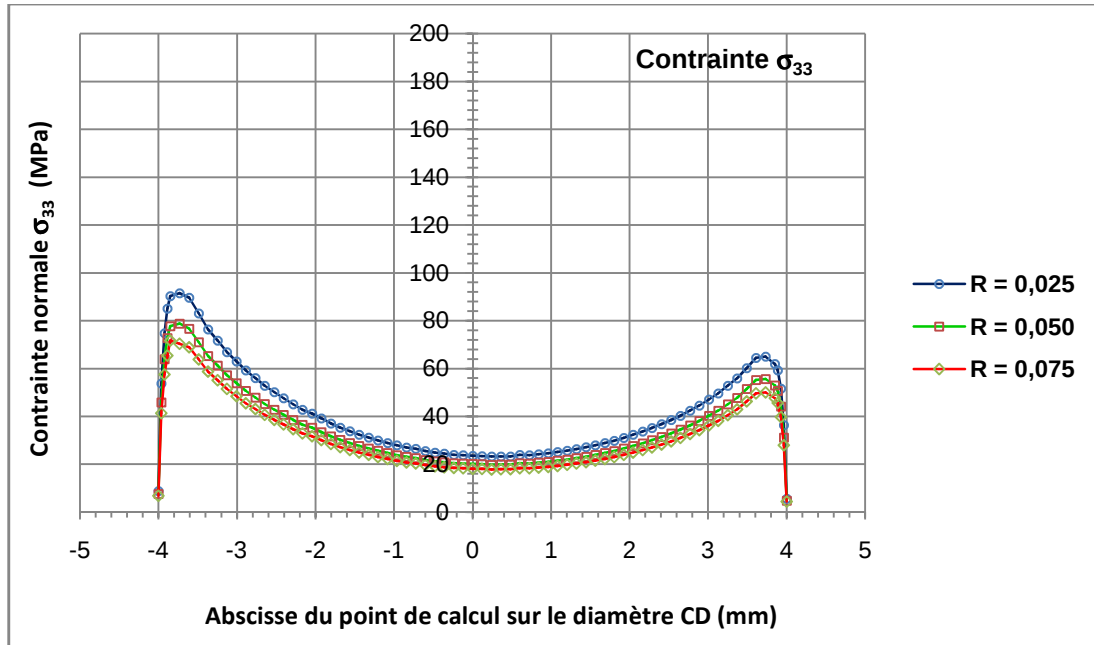
Figure 3.25 – Répartition sur le diamètre CD de la contrainte normale \sigma_{33} pour les trois valeurs distinctes du rayon du congé de raccordement en fond d'entaille
