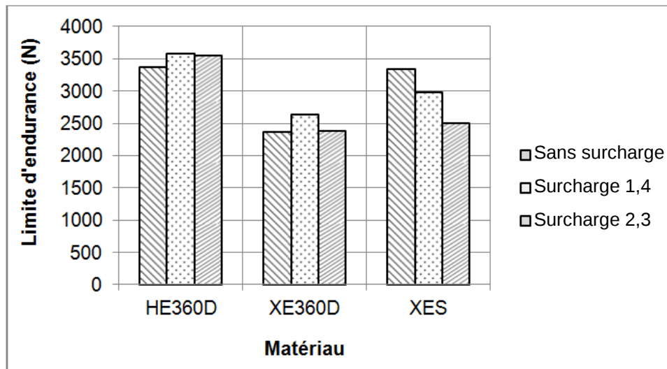
Figure 2.38 – Influence des surcharges incidentelles sur la limite de fatigue à 2.10^6 cycles des éprouvettes soudées par point
