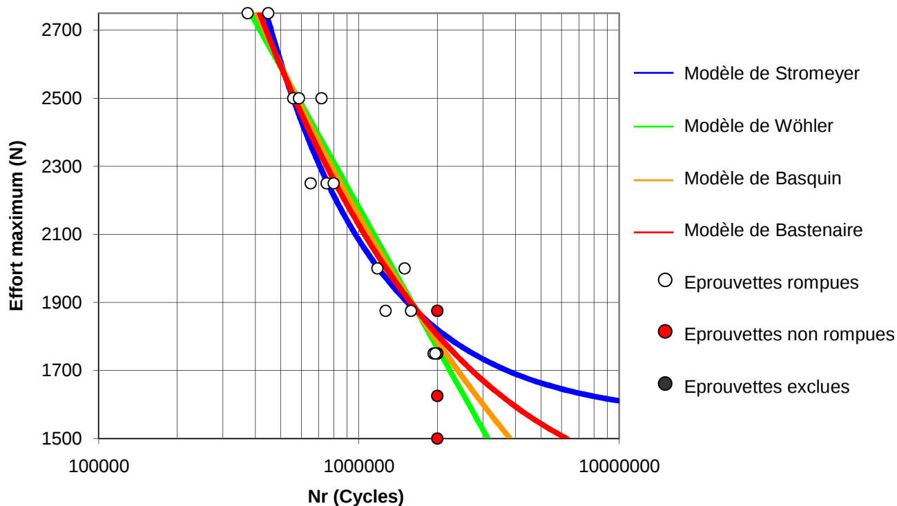
Figure 2.29 – Courbe de référence des éprouvettes soudées par point en acier XE360D
