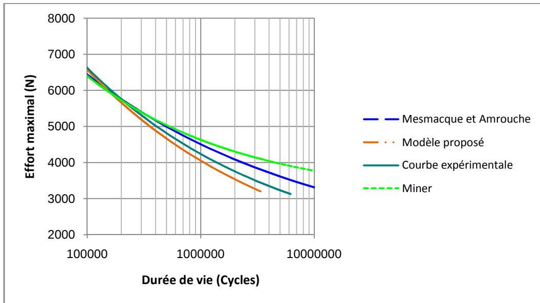
Figure 4.3 – Mat riau HE 360 D, surcharges de rapport 1,4 : courbes de Gassner
