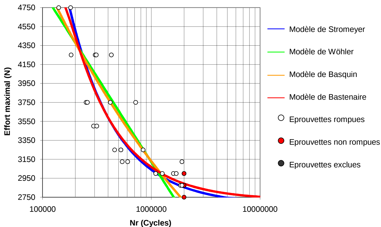
Figure 2.33 – Courbe F-N des éprouvettes en acier XES sous chargement de fatigue avec les surcharges périodiques de rapport 1,4
