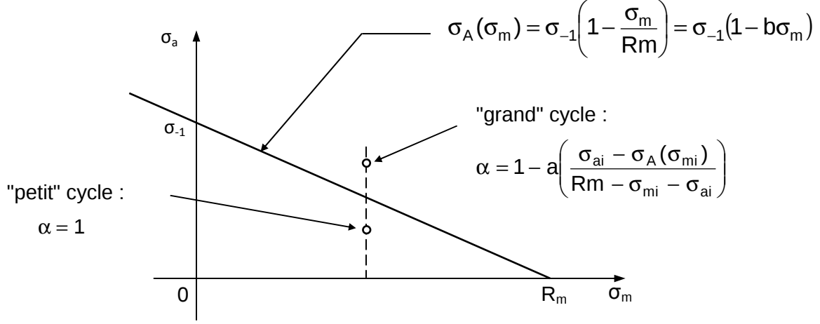
Figure 1.17 – Distinction entre "petit" et "grand" cycles sur le diagramme de Haigh
