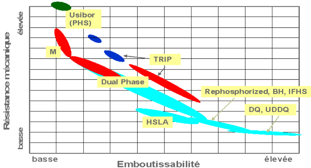
Figure 1.2 – Diagramme résistance mécanique–emboutissabilité des principales nuances de produits plats [ARC08]
