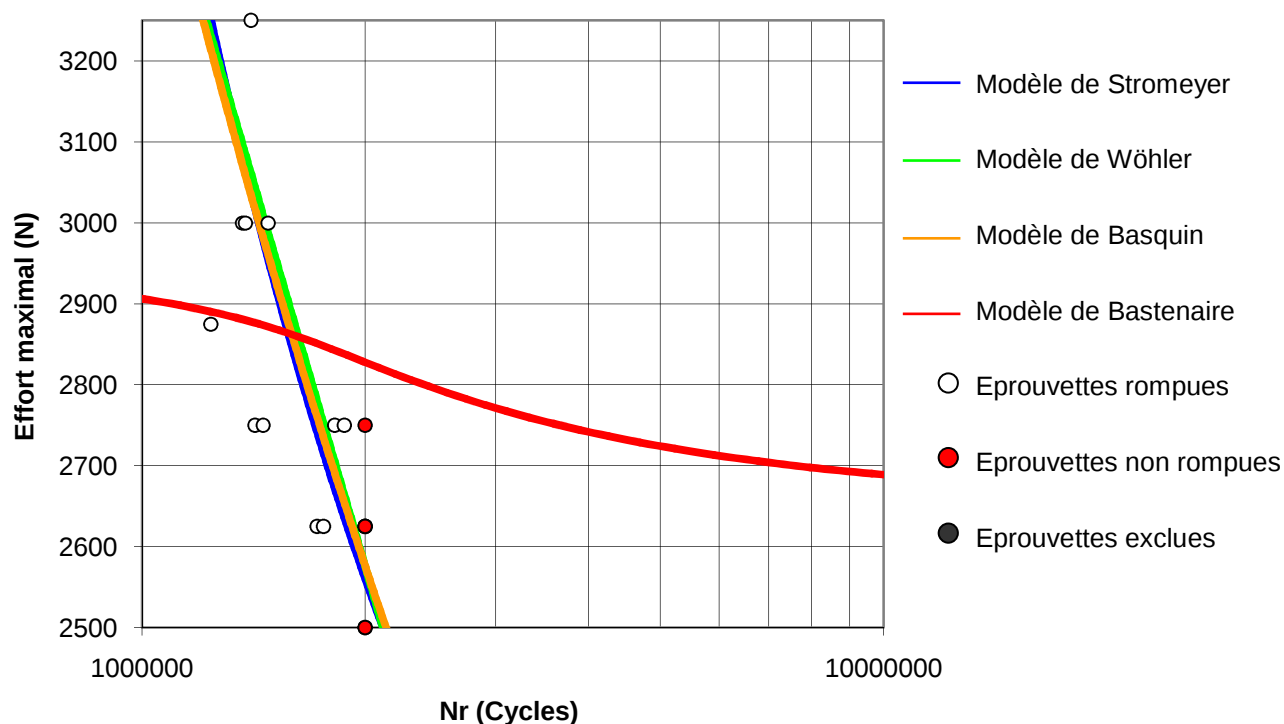
Figure 2.31 – Courbe F-N des éprouvettes en acier XE360D sous chargement de fatigue avec les surcharges périodiques de rapport 2,3
