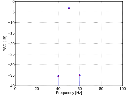
(b) Spectrum via ESPRIT.
