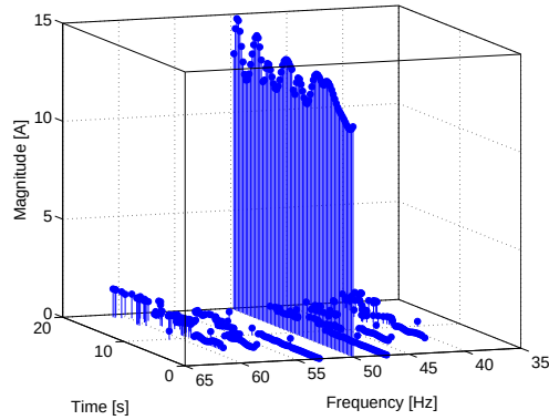
(a) Représentation temps-fréquence basée sur le MD MUSIC.
