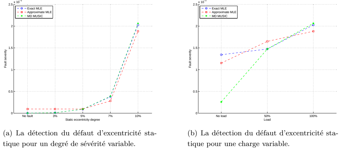
Figure 6.9: Détection du défaut d'excentricité statique en se basant sur les trois techniques proposées.
