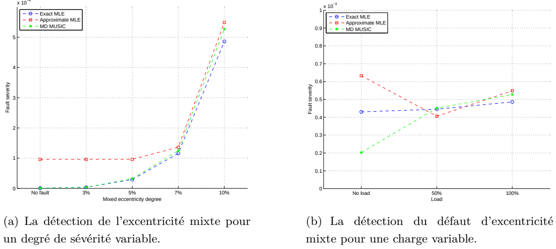
Figure 6.11: Détection du défaut d'excentricité mixte en se basant sur les trois techniques proposées.
