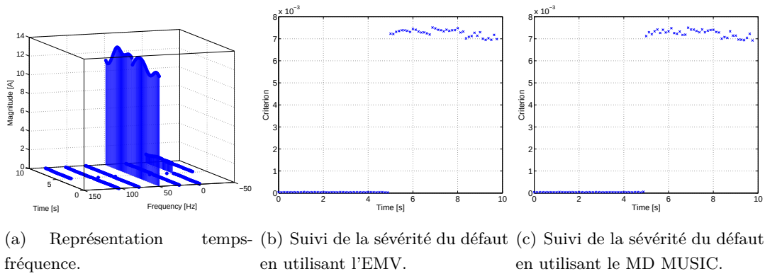
Figure 6.14: Détection de l'excentricité mixte en utilisant les approches non-stationnaires proposées.
