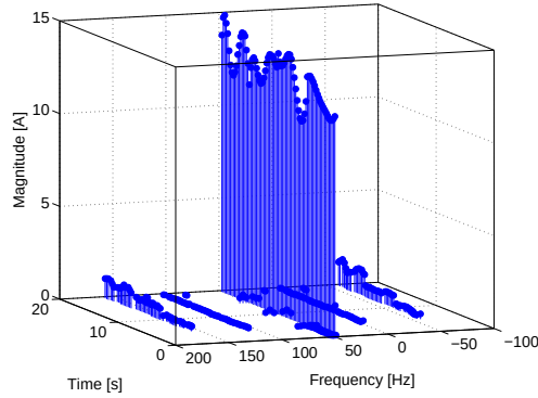
(a) Représentation temps-fréquence basée sur l'EMV.
