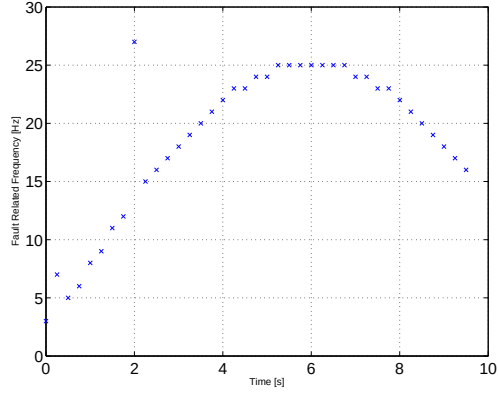
(d) Fault frequency.
