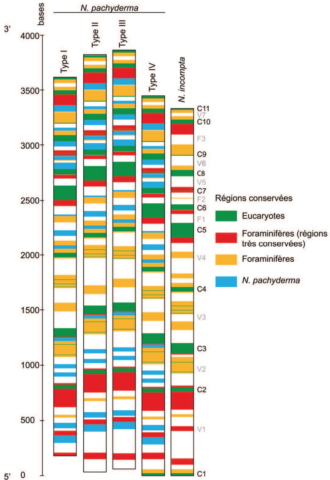
Figure 15: schéma de la SSU complète de Neogloboquadrina pachyderma et Neogloboquadrina incompta . C1 à 9 : régions conservées chez les eucaryotes, V1 à 7 : régions variables, F1 à 3 : régions variables de la fin de la SSU spécifiques des foraminifères (nomenclature d'après Ertan et al., 2004).
