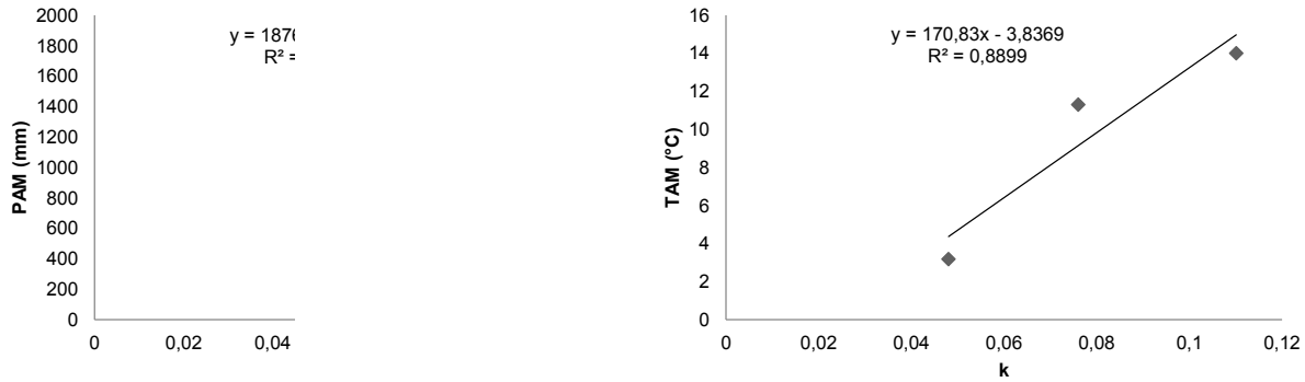
Figure 48 – Corrélations entre les taux de décomposition du bois notés k et les conditions climatiques : PAM (Pluies Annuelles Moyennes) et TAM (Températures Annuelles Moyennes)
