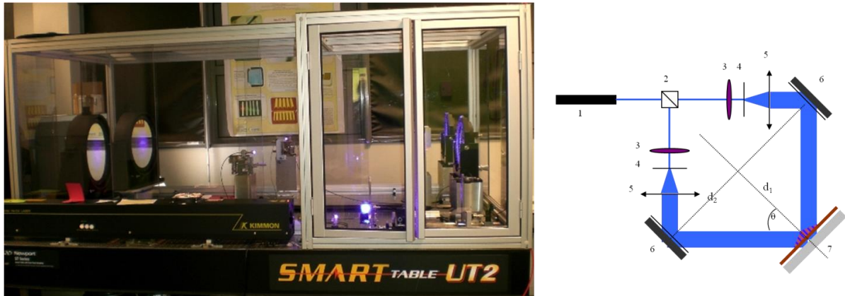
Figure 36 : Banc d’holographie au Laboratoire Hubert Curien (gauche). Le faisceau incident (1) est séparé (2) en deux faisceaux qui passent au travers d’un diaphragme (3) puis sont élargis (4) et collimatés (5) avant d’être renvoyés (6) sur une cible (7).
