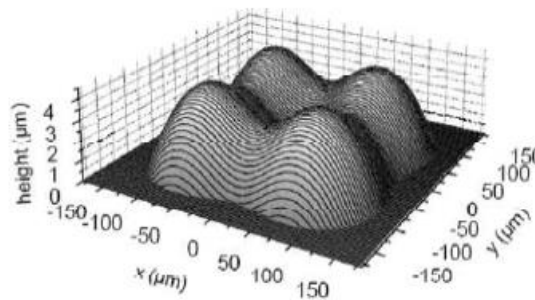
Figure 98 : Profil tridimensionnel de la micro-optique réfractif [6].
