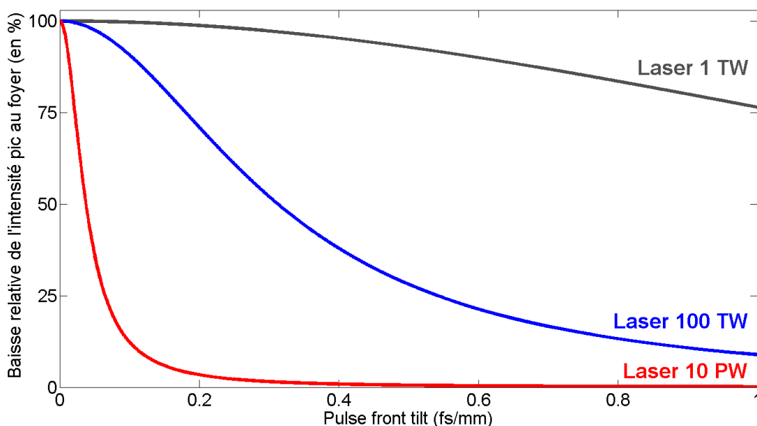
FIGURE 1 – Diminution relative de l'intensité pic au foyer en fonction de la valeur d'un couplage spatio-temporel d'ordre 1 (pulse front tilt). Le pulse front tilt, \xi , exprimé en \text{fs}\cdot\text{mm}^{-1} , correspond à une différence entre le front d'onde et le front d'impulsion. Les trois courbes de ce graphique ont été calculées pour des chaînes lasers Titane-saphire réellement existantes ou en cours de construction, basées sur la technique CPA. Les chaînes délivrant 1 TW et 100 TW correspondent respectivement aux lasers LUCA et UHI 100, sur lesquelles nous avons travaillé durant cette thèse. Le laser LUCA délivrent des impulsions de 45 fs (durée à mi-hauteur) et le faisceau a un diamètre de 2,5 cm. Le durée d'impulsion de la chaîne laser UHI 100 est de 25 fs et le diamètre du faisceau atteint 8 cm. L'installation 10 PW correspond au laser Apollon qui délivrera à terme des impulsions de 15 fs et un faisceau de 40 cm.
