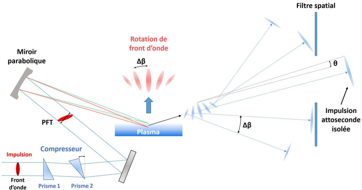
FIGURE A.1 – L'effet phare attoseconde. En focalisant sur une cible une impulsion ultrabrève de haute puissance contenant préalablement du pulse front tilt (dû au désalignement du dernier élément du compresseur optique), la rotation de front d'onde induite au foyer, couplée aux très hautes intensités, va générer un train d'impulsions attosecondes se propageant dans des directions différentes. Dans le cas où la séparation angulaire, \Delta\beta , entre deux impulsions successives est supérieure à la divergence, \theta , des impulsions attosecondes, il est alors possible d'isoler une ou plusieurs de ces impulsions à l'aide d'un filtre spatial. Dans le cas des articles [42, 43], le compresseur optique est composé de prismes et non de réseaux comme nous l'avons vu jusqu'à présent dans cette thèse.
