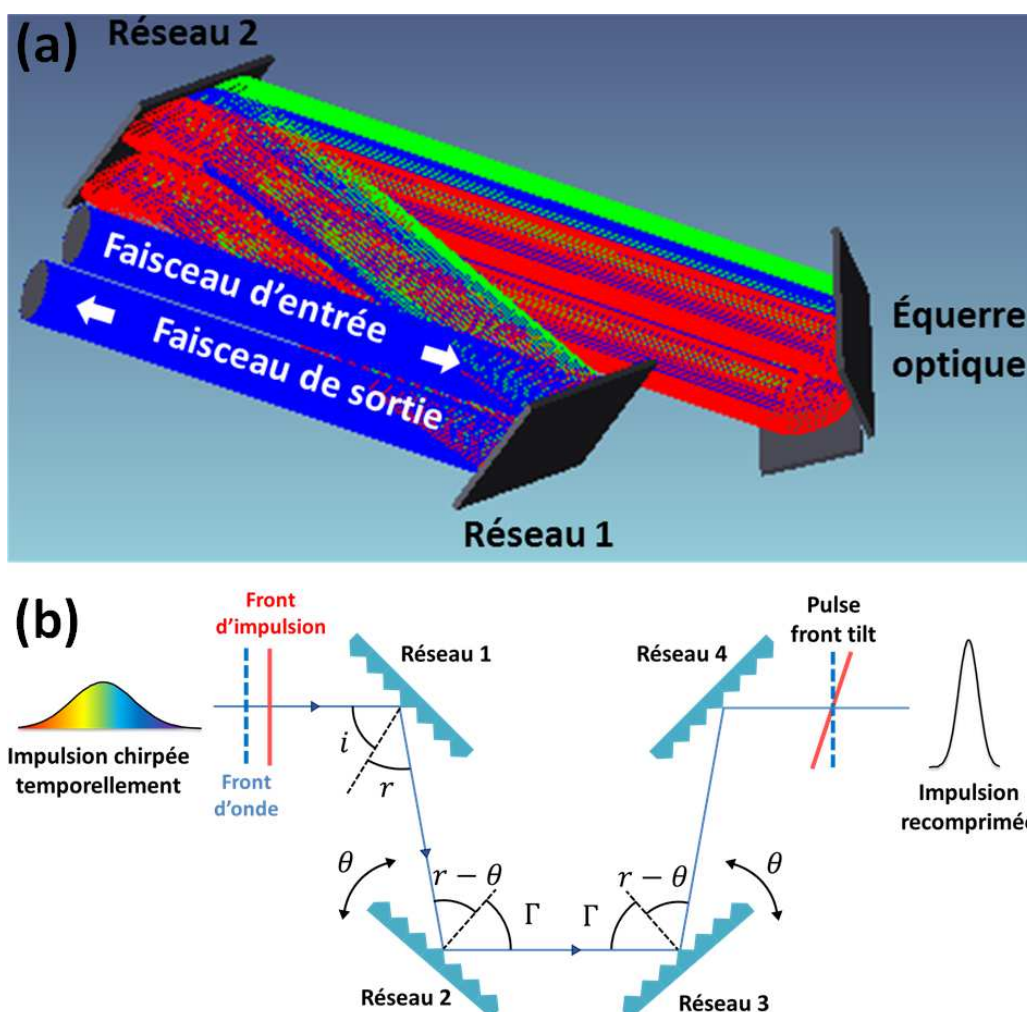
FIGURE 2.7 – Compresseur optique dont le dernier réseau a été désaligné d'un angle \theta . Désalignement d'une paire de réseaux d'un angle \theta . (a) Compresseur optique de la chaîne laser UHI 100 représenté sous Zemax. (b) Schéma d'un compresseur à 4 réseaux équivalent au compresseur (a). Pour générer du pulse front tilt, on désaligne le deuxième réseau du compresseur (a) d'un angle \theta , ce qui revient à désaligner les réseaux 2 et 3 du compresseur à 4 réseaux.
