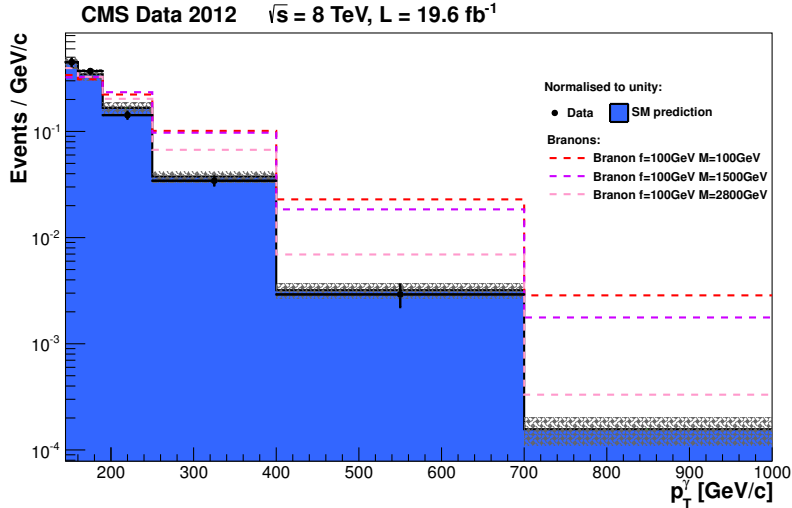
FIGURE 7.48 – Distributions en p_T^\gamma normalisées à l'unité pour les prédictions du modèle standard, les données, et trois modèles de Branons. Les spectres des Branons sont de plus en plus mous à mesure que la masse des Branons augmente.
