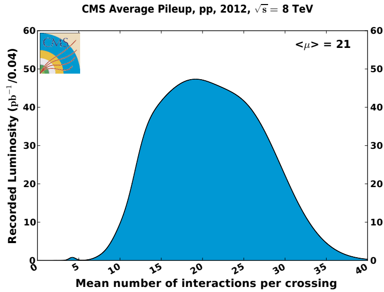
FIGURE 6.5 – Distribution du nombre d'événements d'empilement par croisement de paquets dans les données 2012 [3].
