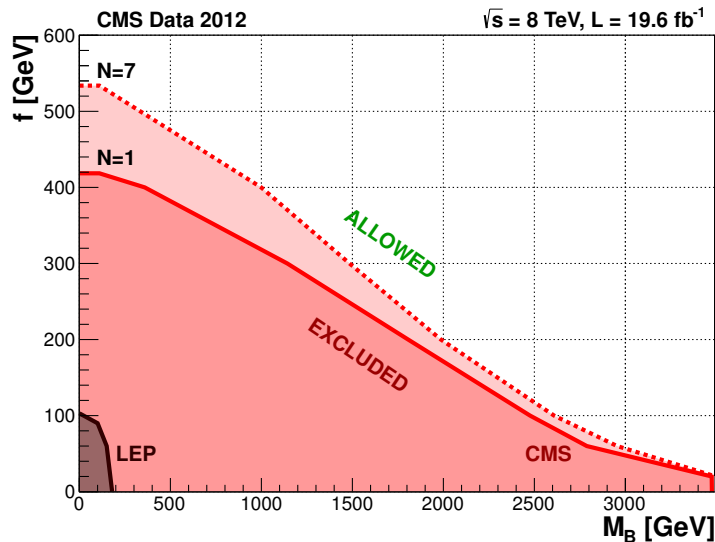
FIGURE 7.50 – Exclusion à 95% de niveau de confiance dans l'espace des paramètres du modèle du Branon par la méthode des formes de spectre, pour deux valeurs du nombre de Branons N .
