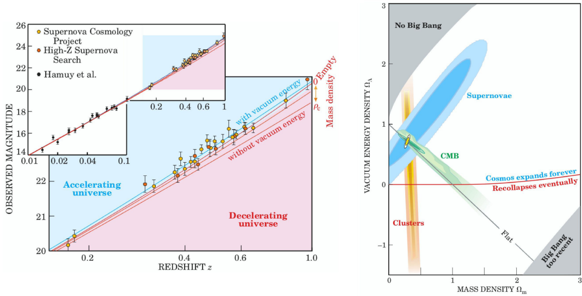
FIGURE 1.11 – Gauche : les mesures des distances de luminosité de 42 supernovae lointaines de type Ia montrent un bon accord avec un modèle \Lambda CDM avec \Omega_\Lambda^0 \approx 0.7 et \Omega_m^0 \approx 0.3 (ligne bleue). Droite : contours de probabilités des paramètres du modèle \Lambda CDM pour différentes sondes ; on voit que sur la ligne \Omega_\Lambda^0 = 0 , fond diffus cosmologique et amas étaient en désaccord ; l'apport des supernovæ a permis de redécouvrir la constante cosmologique. (Figures tirées de la référence [27])
