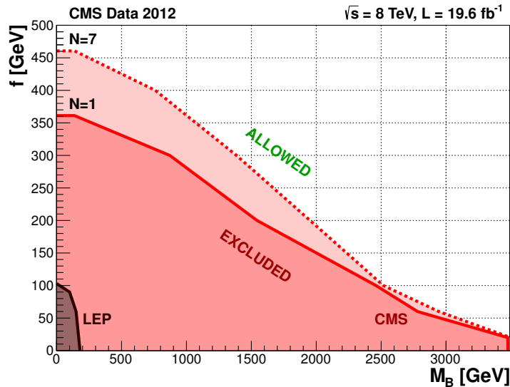
FIGURE 7.47 – Exclusion à 95% de niveau de confiance dans l'espace des paramètres du modèle du Branon par la méthode de comptage, pour deux valeurs du nombre de Branons N .
