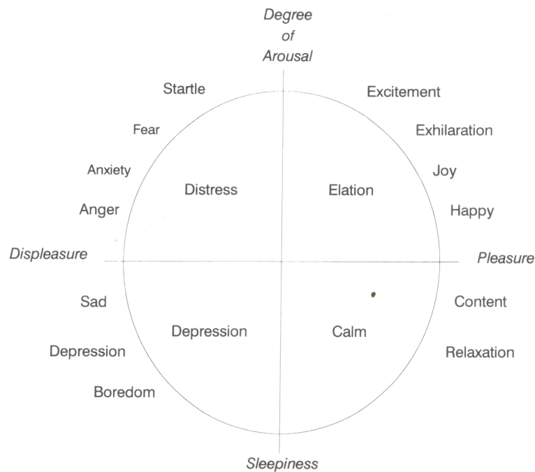
FIG. 5: L'espace plaisir-activation, un espace circomplexe des émotions. Figure tirée de [120].
