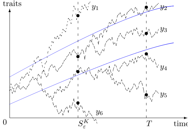
FIGURE 1.2.3 – Le compact \mathcal{K} est la région entre les deux lignes pleines. Les trajectoires dessinées correspondent au support de X_T^K . X_T^K((\mathcal{K}^T)^c) compte les trajectoires qui n'appartiennent pas à \mathcal{K} entre 0 et T : ici, y_1 , y_2 , y_4 , y_5 et y_6 . X_T^K(\{y^{S_\varepsilon^K} \notin \mathcal{K}^{S_\varepsilon^K}\}) compte les trajectoires, au temps T , qui n'appartiennent pas à \mathcal{K} entre 0 et S_\varepsilon^K : ici, y_1 , y_4 , y_5 et y_6 ; en effet, la trajectoire y_2 considérée entre les temps 0 et S_\varepsilon^K appartient à \mathcal{K} . Pour compter les trajectoires qui vont donner X_T^K(\{y^{S_\varepsilon^K} \notin \mathcal{K}^{S_\varepsilon^K}\}) , on compte donc les descendants à T des 3 points au temps S_\varepsilon^K correspondant aux trajectoires y^{S_\varepsilon^K} \notin \mathcal{K}^{S_\varepsilon^K} . On peut également vérifier sur la figure que la relation (1.2.21) est satisfaite.
