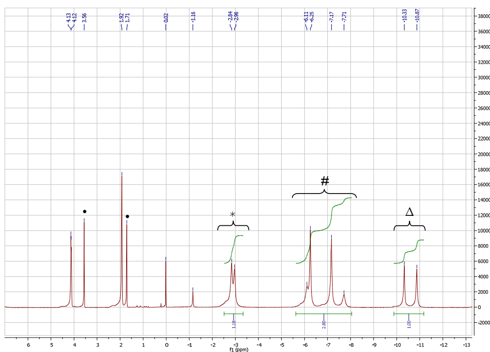
Figure 41 : Spectre de RMN ^1H (500 MHz) du mélange brut de formation de [\{Ce(N^*)_3\}(\mu-CN/NC)\{U(N^*)_3\}][NEt_4] (#) dans le THF- d_8 (•). (*) indique [\{Ce(N^*)_3\}_2(\mu-CN)][NEt_4] ( 2a · [NEt 4 ] ) et (Δ) [\{U(N^*)_3\}_2(\mu-CN)][NEt_4] ( 2b · [NEt 4 ] ).
