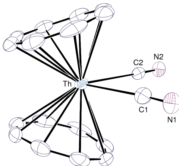
Figure 79 : Vue ORTEP de l'anion [Th(Cot)_2(CN)_2]^{2-} dans le complexe 6 \cdot [N^rBu_4]_2 . Les atomes d'hydrogène et les contre-ions ont été omis.
