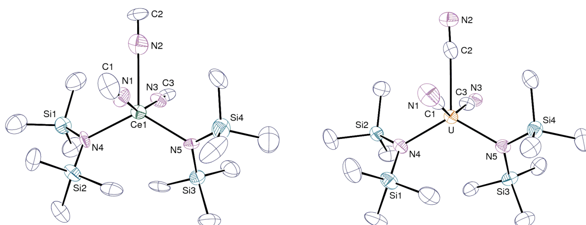
Figure 40 : Vues ORTEP des anions [M_f(N^*)_2(CN)_3]^{2-} dans 4a \cdot [N^u\text{Bu}_4]_2 (à gauche) et 4b \cdot [N^u\text{Bu}_4]_2 (à droite). Les atomes d'hydrogène et les contre-ions ont été omis.
