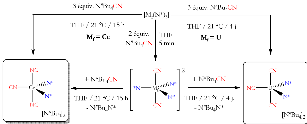
Figure 39 : Formation des complexes tris-cyanures [M_f(N^*)_2(CN)_3][N^u\text{Bu}_4]_2 ( 4 \cdot [N^u\text{Bu}_4]_2 ).
