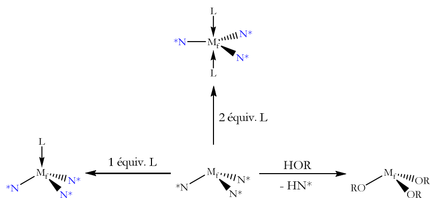
Figure 20 : Réactivité de [M_f(N^*)_3] avec les bases de Lewis ( L ) et les molécules acides.
