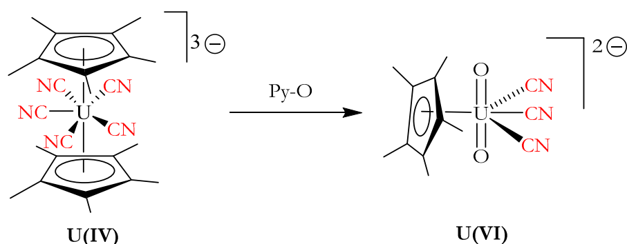
Figure 15 : Synthèse du premier complexe cyclopentadiénylique d'uranyle [\text{UO}_2(\text{Cp}^*)(\text{CN})_3][\text{NEt}_4]_2 .
