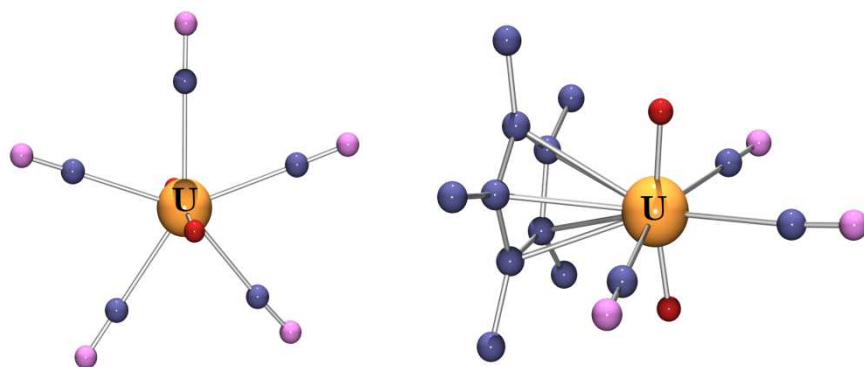
Figure 16 : Structures moléculaires de [\text{UO}_2(\text{CN})_5][\text{NEt}_4]_3 et [\text{UO}_2(\text{Cp}^*)(\text{CN})_3][\text{NEt}_4]_2 .
