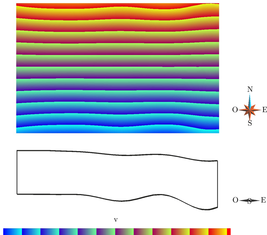
FIGURE 4.9 – Effet de Poisson affectant le calcul de v . Le paramètre v calculé par restauration progressive est affiché en vue de dessus sur le modèle dans son état initial. Le contour des structures est représenté en dessous, vu du Sud, afin d’illustrer la correspondance entre les zones de contraction (intrados des plis) et de dilatation (extrados des plis) de v avec les structures présentes dans le modèle. Cet effet est lié au comportement mécanique du modèle de roche utilisé et plus spécifiquement au coefficient de Poisson.
