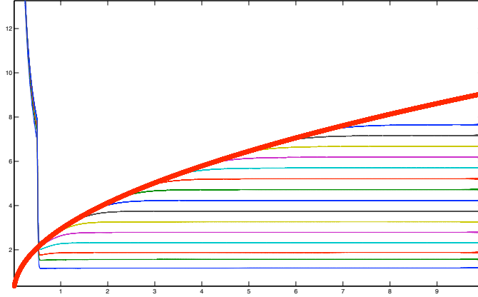
FIGURE 7 – SIMULATIONS NUMÉRIQUES DE (12) AVEC UNE DONNÉE INITIALE DE TYPE "CLOCHE". LA DENSITÉ M EST UNE GAUSSIENNE. CHAQUE TRACÉ CORRESPOND À LA VITESSE DU FRONT POUR UNE TRONCATURE PARTICULIÈRE DE L'ESPACE DES VITESSES. ON OBSERVE QUE L'ENVELOPPE DE CES COURBES EST TRÈS PROCHE DE t \mapsto t^{1/2} . AINSI, LA LOI D'ÉCHELLE POUR LA PROPAGATION AVEC DES VITESSES NON-BORNÉES EST APPROXIMATIVEMENT x \sim t^{3/2} . CE TAUX DE PROPAGATION EST DÉMONTRÉ AU CHAPITRE 2, OÙ L'ON TROUVERA DE MÊME PLUS DE DÉTAILS CONCERNANT CES SIMULATIONS NUMÉRIQUES.
