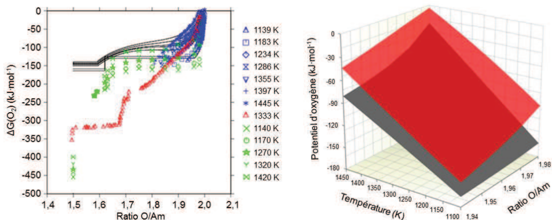
Figure I-7. Comparaison des potentiels d'oxygène des oxydes d'américium mesurés par Chikalla et Eyring [169] (en bleu), Casalza [54,55] (en vert) et Otobe et al. [116] (en rouge) aux données calculées d'après le modèle thermodynamique de Gotcu-Freis et al. [112] (en noir), à gauche, et comparaison des données de Chikalla et Eyring (en rouge) et de Casalza (en gris), selon Gotcu-Freis et al., à droite.
