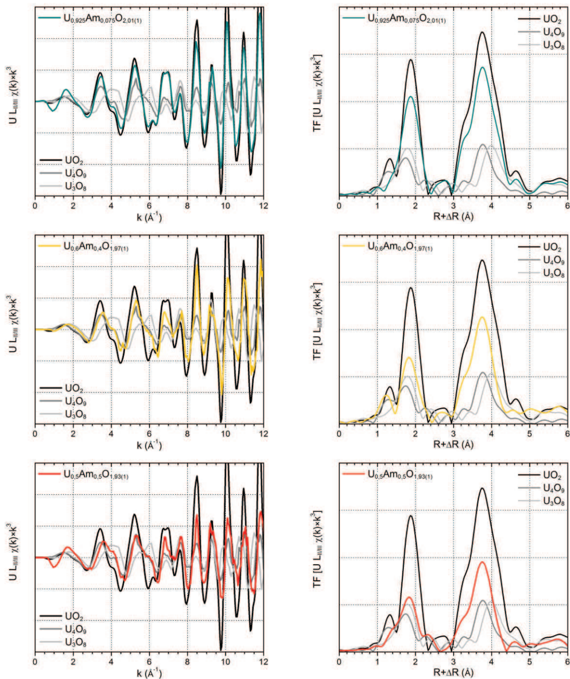
Figure III-14. Spectres EXAFS, à gauche, et transformées de Fourier correspondantes, à droite, au seuil U L II des composés U 1-x Am x O 2±δ de teneurs Am/(U+Am) de 7,5 (—), 40 (—) et 50 %mol (—) comparés à ceux de composés de référence UO 2 , U 4 O 9 et U 3 O 8 .
