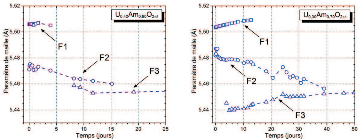
Figure III-6. Évolution durant les premiers jours de suivi par DRX sur poudre des paramètres de maille des phases F1 ( \square ), F2 ( \circ ) et F3 ( \triangle ) des échantillons présentant des teneurs Am/(U+Am) de 60 %mol, à gauche, et 70 %mol, à droite.
