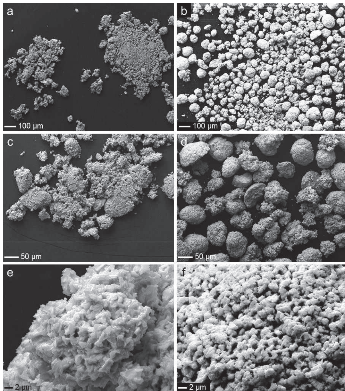
Figure II-5. Micrographies par MEB-FEG en mode électrons secondaires des précurseurs \text{AmO}_2 -Lot 1, à gauche, et \text{AmO}_2 -Lot 2, à droite.
