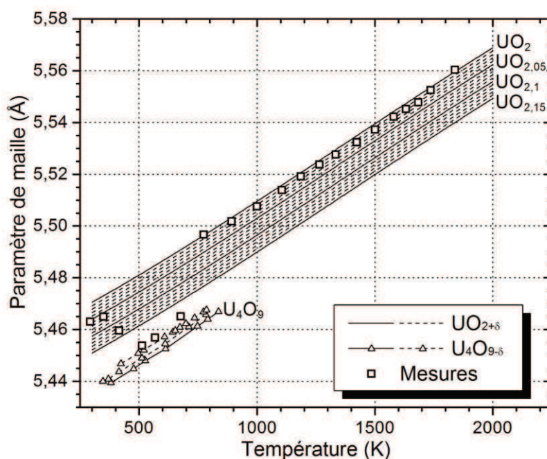
Figure II-14. Comparaison des paramètres de maille de la phase UO_{2+\delta} au cours de la montée en température aux données de la littérature pour les phases UO_{2+\delta} et U_4O_9 [67,83,206].
