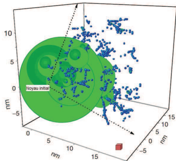
Figure I-22. Exemple (calculé avec SRIM-2003 [256]) de cascade de collisions provoquée par un noyau de recul ( \sim 100 keV) d'une désintégration \alpha dans l' \text{UO}_2 (extrait de [253], page 467). Les sphères vertes représentent les atomes d'uranium, les bleues, les atomes d'oxygène. La taille de la sphère représente, l'énergie transmise lors de la collision. Le cube rouge représente le volume approximatif occupé par huit mailles de type fluorine d' \text{UO}_2 .
