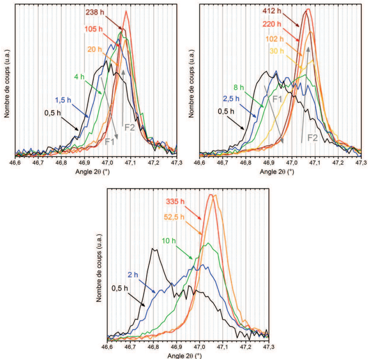
Figure III-2. Extraits des diagrammes de DRX sur poudres des échantillons ayant des teneurs Am/(U+Am) de 30 %mol, en haut à gauche, 40 %mol, en haut à droite, et 50 %mol, en bas, centré sur les pics (2 2 0) de la structure de type fluorine enregistrés en conditions ambiantes après un traitement thermique sous atmosphère réductrice. Les contributions de la raie Cu K_{\alpha 2} et du fond continu ont été retirées.
