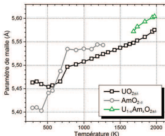
Figure II-13. Évolution des paramètres de maille des phases UO_{2+\delta} , AmO_{2-\delta}/C-Am_2O_{3+\delta} et U_{1-x}Am_xO_{2+\delta} au cours de la montée en température.
