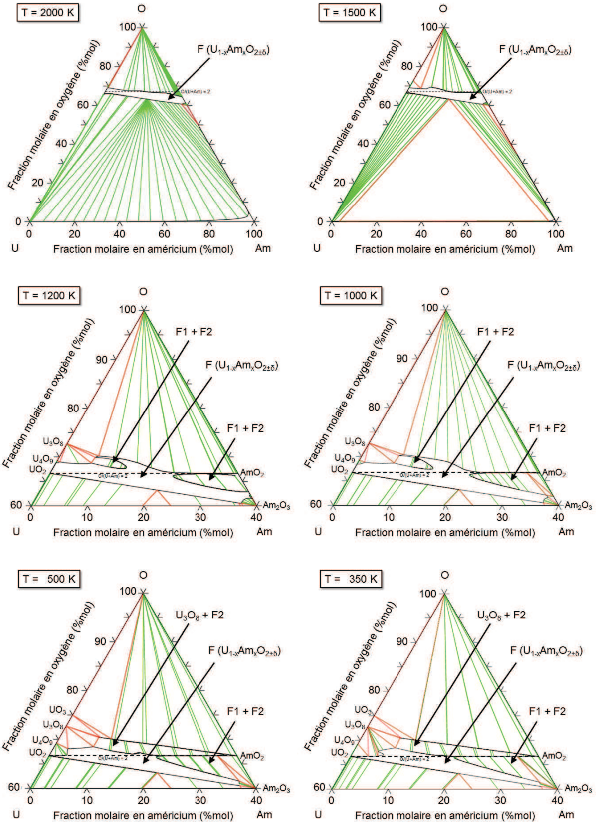
Figure IV-20. Diagrammes de phase ternaires U-Am-O obtenus après ajustement des paramètres à différentes températures : 2000, 1500, 1200, 1000, 500 et 350 K (à P = 1 atm).
