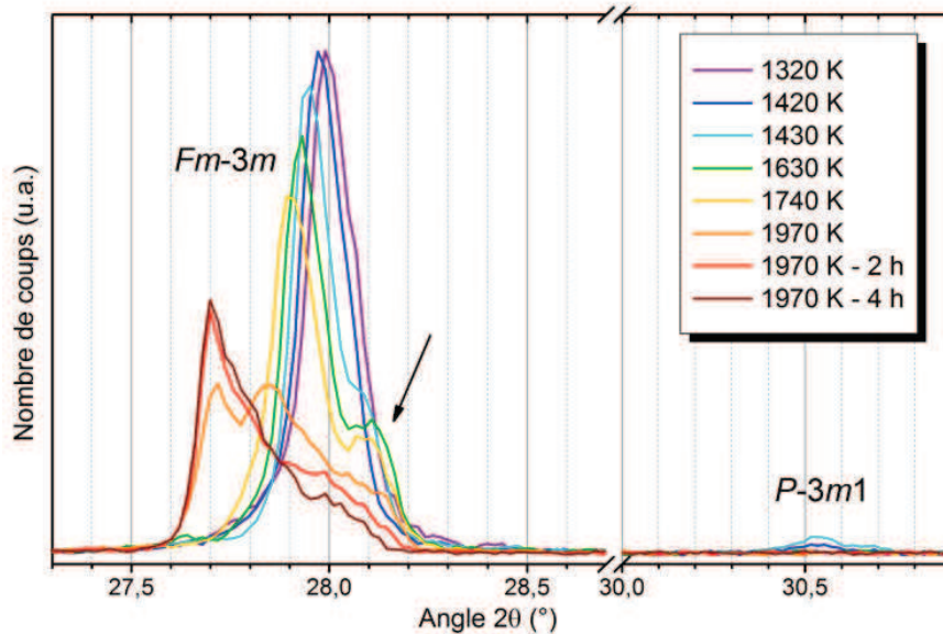
Figure II-15. Extraits des diagrammes de DRX sur poudre obtenus lors du cycle thermique réalisé entièrement sous hélium. Les pics entre 27,5 et 28,5^\circ 2\theta sont les pics principaux des phases de structures de type fluorine, celui proche de 30,5^\circ 2\theta correspond au pic principal de la phase \text{Am}_2\text{O}_3 de type A. Les contributions de la raie \text{Cu } K_{\alpha 2} et du fond continu ont été retirées.
