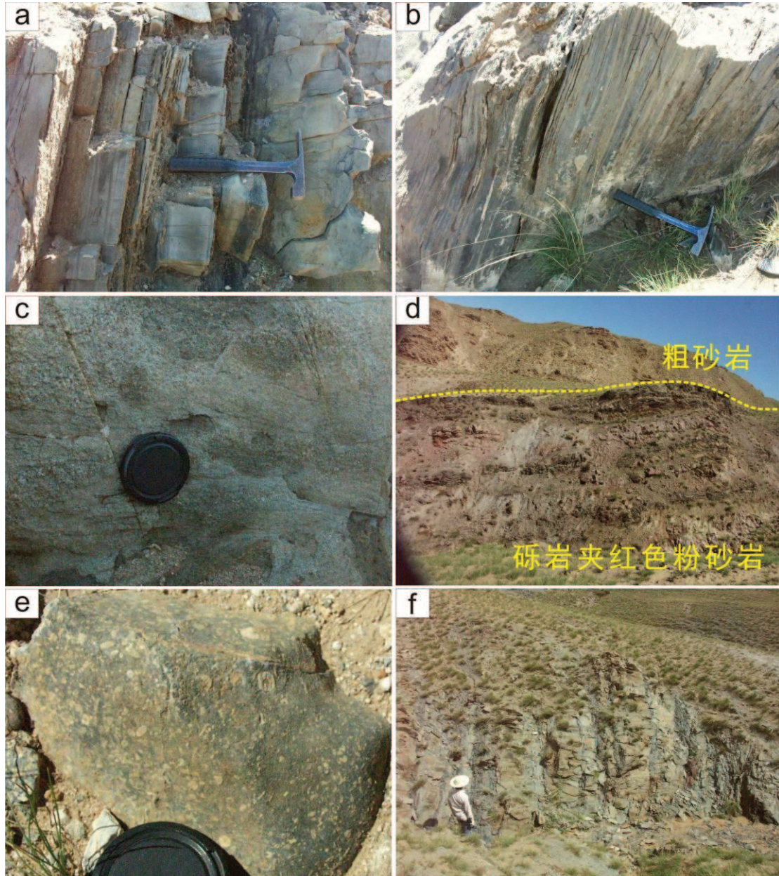
图5-6 温都尔庙地区下二叠统呼格特组野外照片 a, 下部发育水平层理薄层粉砂岩; b, 薄层砂质灰岩; c, 含砾粗砂岩中的斜层理; d, 砾岩夹红色粉砂岩与上部粗砂岩接触; e, 灰岩中的瓣类化石; f, 剖面上部砂岩与黑色粉砂岩互层
