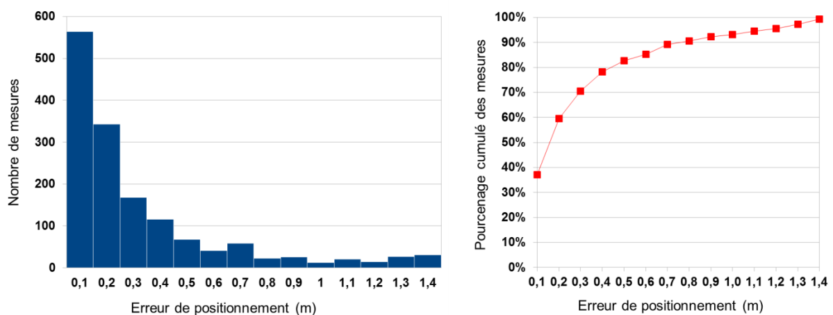
Figure II-29 Erreurs du positionnement basées sur la vision pour 1525 mesures effectuées à une distance de 2, 4, 8 ou 10 mètres d'un point visuel.
