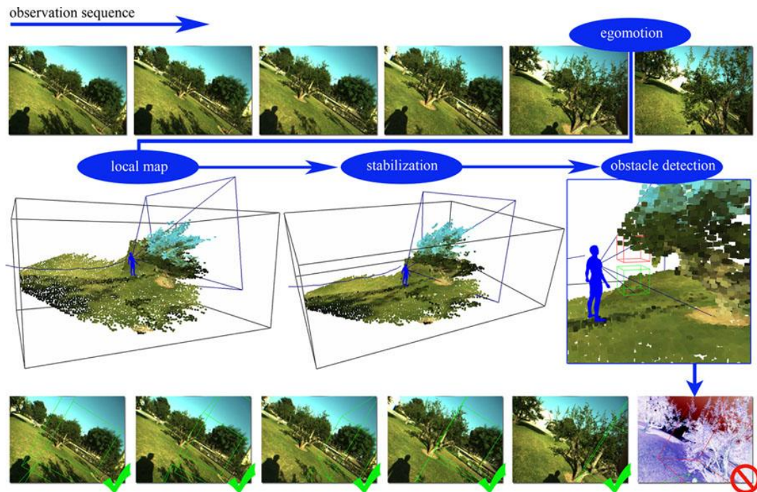
Figure I-43 Architecture de la méthode de détection d'obstacle proposée dans [Martinez et al., 2008]. Celle-ci repose sur la construction d'une carte 3D de l'environnement par odométrie visuelle, puis de sa stabilisation par rapport au plan horizontal, et finalement de la classification des obstacles face à l'utilisateur.
