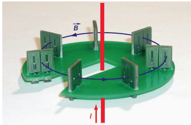
Figure 1.6 : Capteur de courant PRiME développé par LEM [17]
