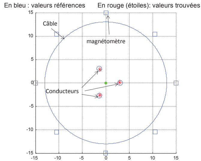
Figure 3.6 : Reconstruction des positions des conducteurs
