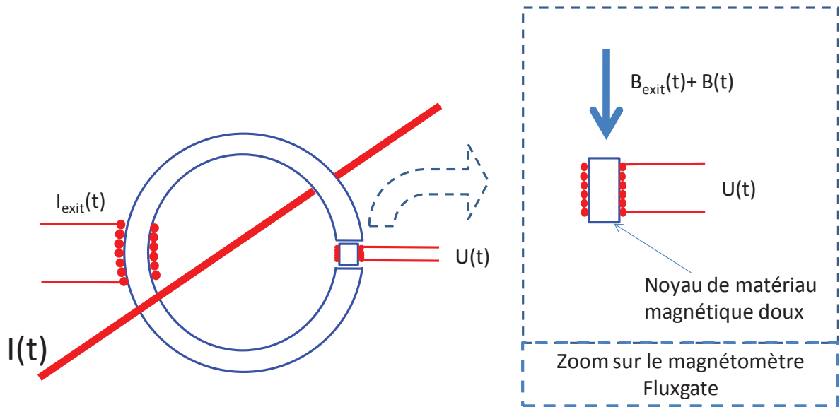
Figure 1.12 : Schéma d'un capteur de courant utilisant un magnétomètre Fluxgate
