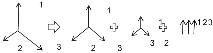
Figure 4.18 : Décomposition d'un système déséquilibré en système direct inverse et homopolaire.
