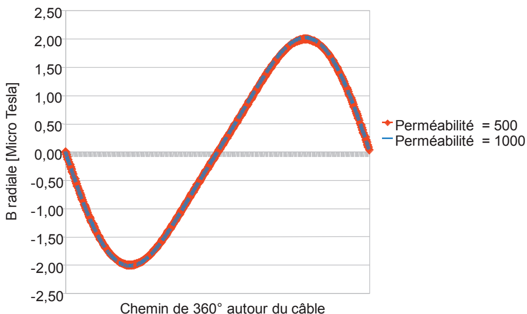
Figure 3.23 : Induction magnétique B radiale pour un diamètre R_{\text{Blind}}=30 mm du blindage E = 0.94 %.
