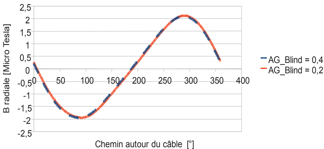
Figure 3.28 : Induction magnétique B radiale pour un entrefer du blindage de AG\_Blind = 0.4 mm (en bleu) et AG\_Blind = 0.2 mm (en rouge). E = 0.1 %.
