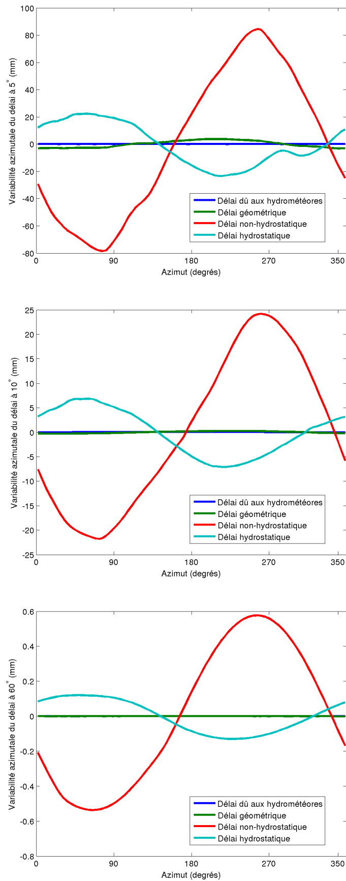
FIGURE 5.42 – Variabilité azimutale des composantes du délai troposphérique à 5^\circ (haut), 10^\circ (milieu) et 60^\circ (bas) d'élévation pour le site TLSE le 2 août 2013 à 00h UTC.
