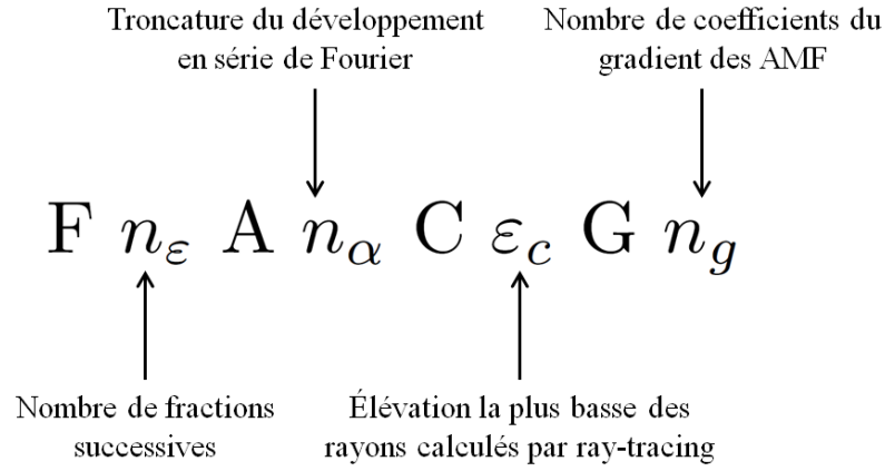
FIGURE 2.2 – Nomenclature de la forme des AMF (ex : F3A4C5G2).
