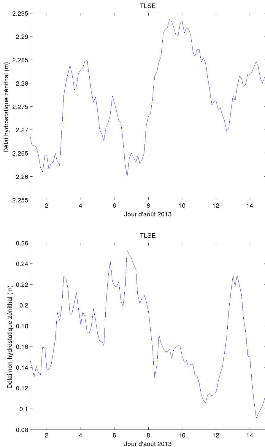
FIGURE 5.34 – Variations temporelles des délais zénithaux hydrostatiques (haut) et non-hydrostatiques (bas) pour le site TLSE pour les 15 premiers jours d'août 2013.
