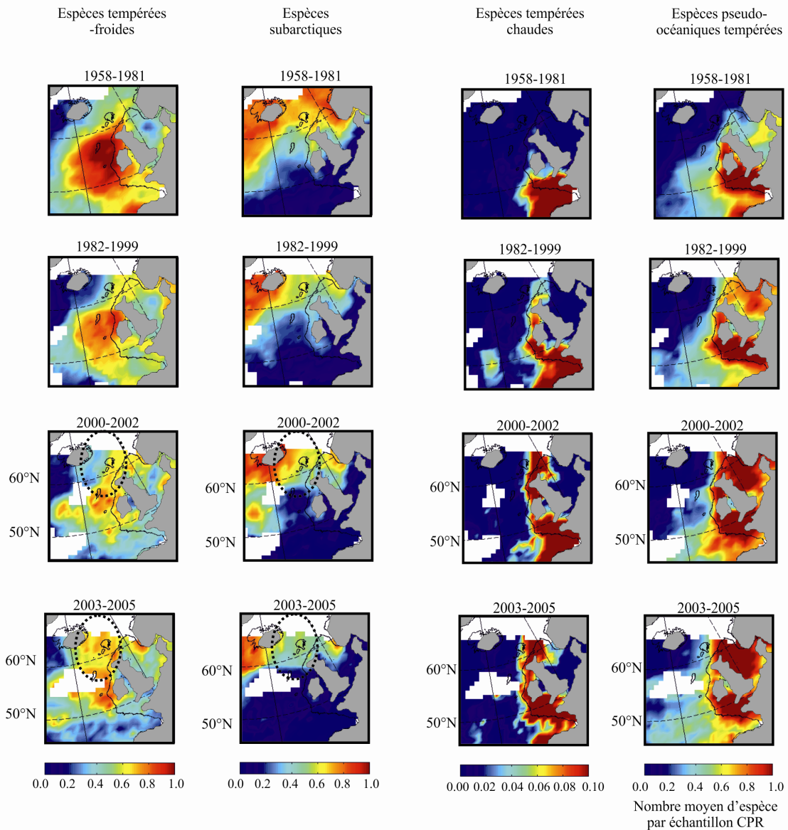
Figure A-I-4. Changements à long-terme de la diversité (nombre d'espèces) de quatre assemblages de copépodes dans l'océan Atlantique Nord-Est pour la période 1958-2005. D'après Beaugrand et al. (2009) .
