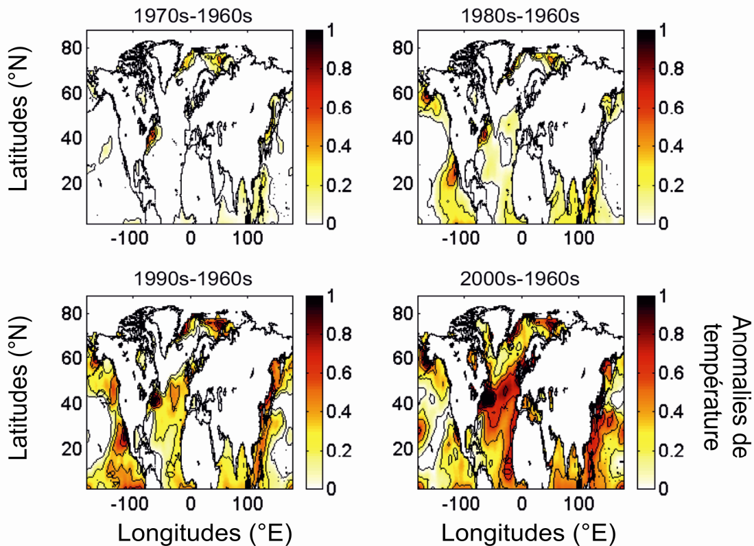
Figure A-I-2. Régionalisation des changements des températures de surface dans l'hémisphère Nord. Les températures ont été moyennées par décennie (à l'exception de la période 2000-2006) et ont été soustraites par la moyenne des températures de surface pour la période 1960-1969. Les données utilisées ici proviennent de la base de données ERSST.v2 (NOAA/OAR/ESRL PSD, Boulder, Colorado, USA, http://www.cdc.noaa.gov/ ). D'après Beaugrand (2009).
