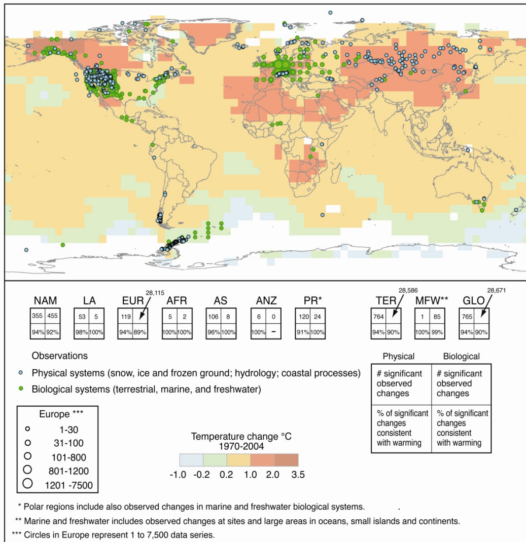
Figure I-2. Emplacement des changements significatifs relevés dans les séries de données sur les systèmes physiques (neige, glace et sol gelé ; hydrologie ; processus côtiers) et les systèmes biologiques (terrestres, marins et dulcicoles) et variations de la température de l'air en surface pendant la période 1970-2004. Quelque 29 000 séries de données ont été retenues sur les 80 000 publiées dans 577 études, sur la base des critères suivants : 1) se terminer en 1990 ou plus tard ; 2) s'étendre sur une période d'au moins 20 ans ; 3) présenter un changement significatif, dans un sens ou dans l'autre, ayant fait l'objet d'une évaluation dans certaines études. Les séries retenues proviennent de quelque 75 études, dont 70 environ ont été réalisées après la parution du TRE. Sur ces 29 000 séries de données, 28 000 environ sont tirées d'études européennes. Les zones laissées en blanc sont des zones où les données d'observation sont insuffisantes pour qu'il soit possible d'y définir une tendance de la température. Les cases 2x2 indiquent le nombre total de séries de données présentant des changements significatifs (rangée supérieure) et la proportion de celles qui concordent avec le réchauffement (rangée inférieure) pour i) les régions continentales : Amérique du Nord (NAM), Amérique latine (LA), Europe (EUR), Afrique (AFR), Asie (AS), Australie et Nouvelle-Zélande (ANZ), régions polaires (PR) ; ii) la planète entière : terres émergées (TER), zones marines et dulcicoles (MFW), globe dans son ensemble (GLO). La somme des différents nombres d'études figurant dans les sept cases des régions continentales (NAM, LA, EUR, AFR, AS, ANZ, PR) ne correspond pas au total de la case du globe dans son ensemble (GLO), parce que ces nombres (à l'exception de celui qui concerne les régions polaires) n'incluent pas les études sur les systèmes marins et dulcicoles (MFW). Les grandes zones marines affectées n'apparaissent pas sur la carte. {GT II figure RiD.1, figure 1.8, figure 1.9 ; GT I figure 3.9b}. D'après IPCC Fourth Assessment Report 2007.
