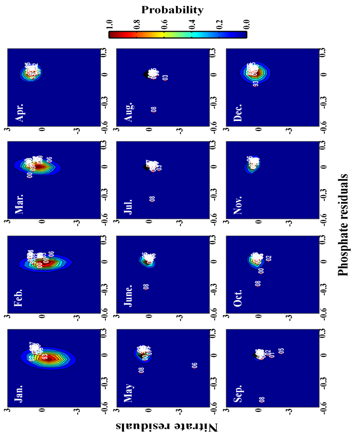
Figure A-V-3. Cartographie des états de référence relatifs pour la station de Villefranche-sur-Mer en fonction des concentrations en nitrate et phosphate d'origine anthropogénique (résidus des analyses de multirégression linéaire multiple, voir Figure V-2) de Janvier (Jan.) à Décembre (Dec.). La couleur symbolise la probabilité qu'une observation appartienne à l'état de référence relatif. Chaque année, de 1993 à 2009 sont superposées à l'espace Euclidien pour le mois donné. La distance entre une année donnée et le centroïde de plus forte probabilités est directement donnée par la probabilité de l'année ( d=1-p , voir méthodes). Les années manquantes sont dues à l'absence d'échantillonnage lors de conditions météorologiques défavorables.
