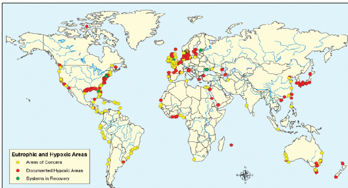
Figure I-4. Cartographie mondiale des systèmes côtiers présentant des phénomènes d'eutrophisation majeurs (en jaune), des zones à événements hypoxiques récurrents (en rouge), et des systèmes en voie de rétablissement (en vert). Les données sont disponibles sur : www.wri.org/project/water-quality et compilées depuis de nombreuses sources par R. Diaz, M. Selman et Z. Sugg. D'après Selman et al. 2008.
