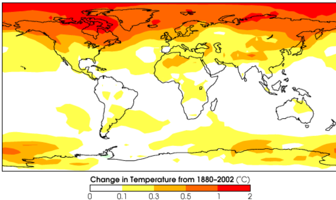
Figure I-3. (a) Changements à long-terme (1880-2007) des températures de surface à l'échelle globale (moyennes annuelles en noir, et données lissées en rouge). (b) Cartographie mondiale des changements à long-terme (1880-2002) des températures de surface témoignant d'un réchauffement plus intense aux latitudes élevées de l'Hémisphère Nord. Les données proviennent du "National Climatic Data Center" (NCDC : http://www.ncdc.noaa.gov/ ).
