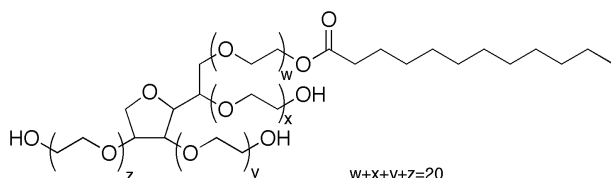
Figure 3.5. Formule chimique du Tween 20 ou Polysorbate 20. On a w+x+y+z = 20 .
