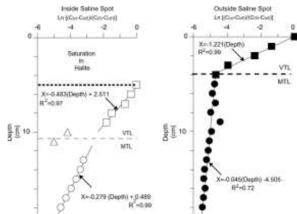
Figure 11 : Décroissances des teneurs en chlorures avec la profondeur et ruptures de pentes dans les 20 premiers cm [AC9].VTL : zone de transfert vapeur, MTL : Zone de transfert mixte
