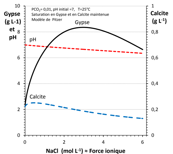
Figure 4 Exemple d'évolution de la solubilité du gypse et de la calcite en fonction de la force ionique d'une solution (Simulation avec Phreeqc). (Figure conçue à des fins pédagogiques-Unpublished)
