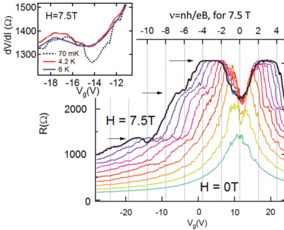
Figure 0.0.3: La résistance différentielle en fonction la grille d'échantillon ReW au champ magnétique de 0 à 7.5T. T=70 mK. L'inséré montre comment le plateau Hall à 7.5T et V_G = 14 V évolue quand la température augmente.
