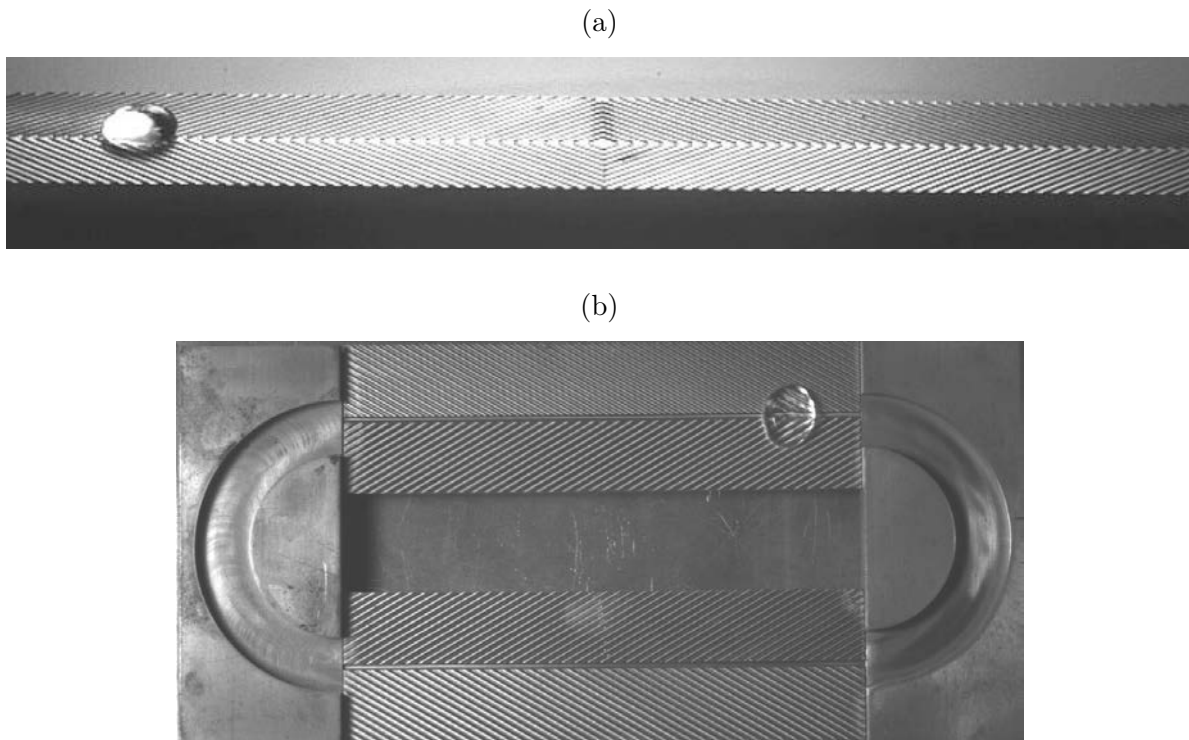
Figure C.3 – Dispositifs utilisant les textures en forme de chevron comme unité de base. (a) Deux chevrons juxtaposés avec des polarités opposées permettent de piéger une goutte à leur intersection. (b) Deux chevrons reliés par des sections circulaires vont faciliter l'observation du mouvement de la goutte sur de très longues distances.
